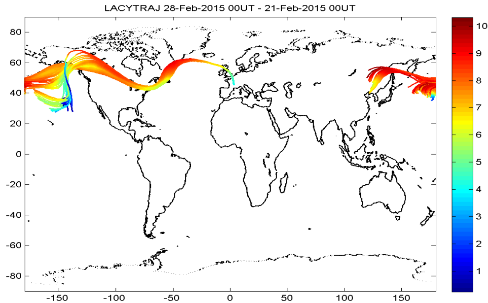
Figure 3.12. Rétro-trajectoires montrant l'évolution de la masse d'air arrivant au-dessus de Clermont-Ferrand le 28 février 2015 à 0h (7 jours de rétro-trajectoires). La couleur indique l'altitude des points de trajectoire (en km).
