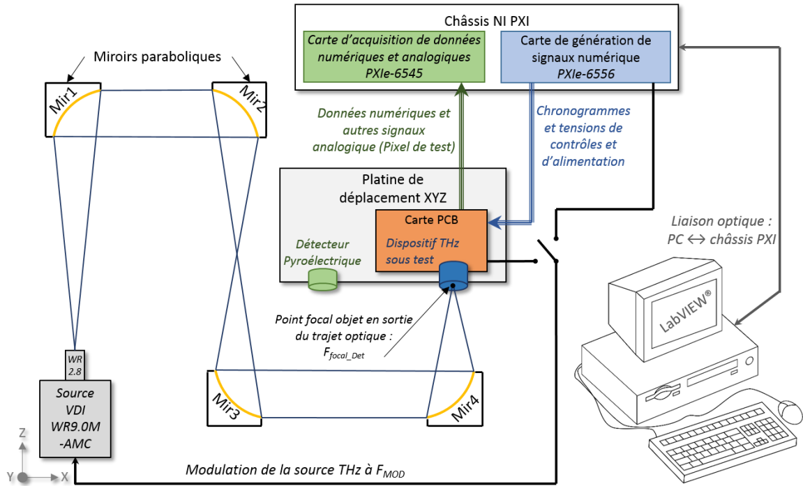
Figure 5.9 : Banc de mesures et caractérisation THz.
