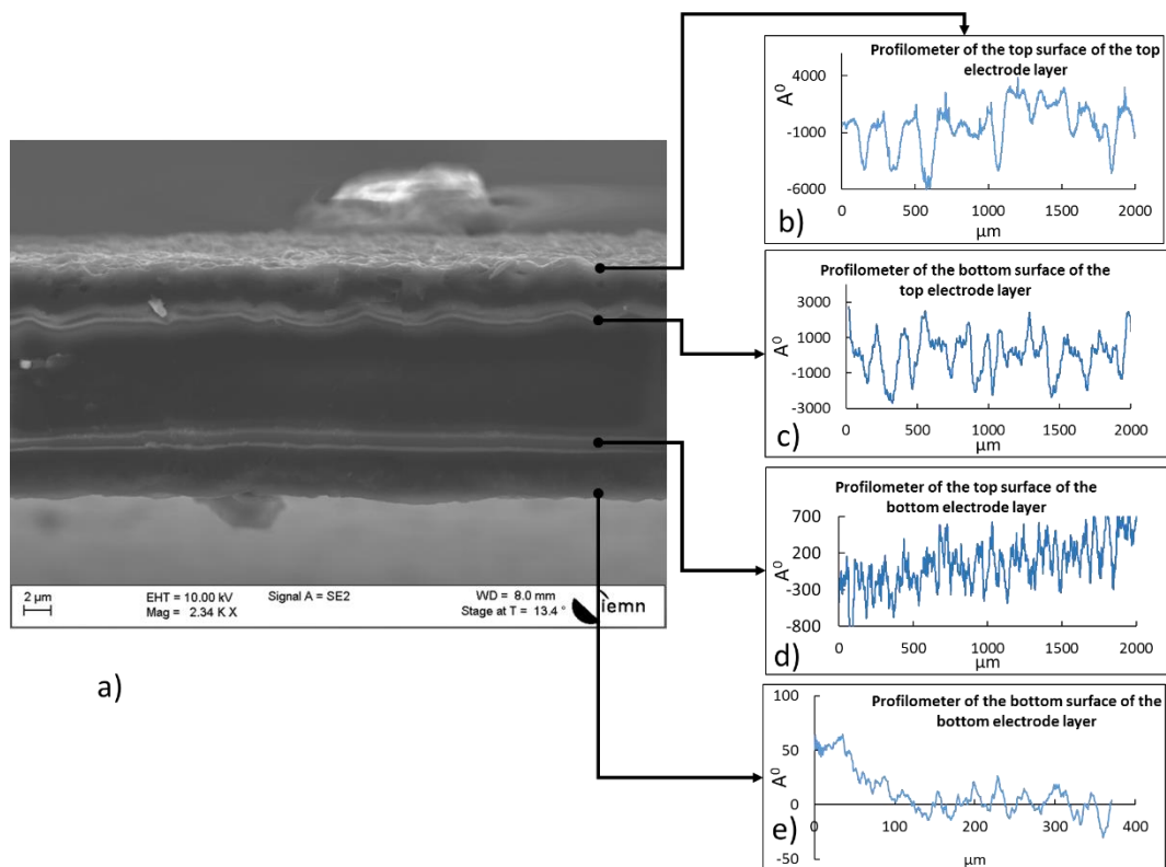
Fig.2 a) Image MEB de la coupe transversale de la tri couche non gonflé de liquide ionique, rugosité de la surface par profilométrie de la surface supérieure de l'électrode supérieure, c) de la surface supérieure du polymère support d'électrolyte (NBR/POE) sur un bicouche PEDOT/SPE, d) de la surface supérieure de l'électrode inférieure, e) de la surface inférieure de l'électrode inférieure
