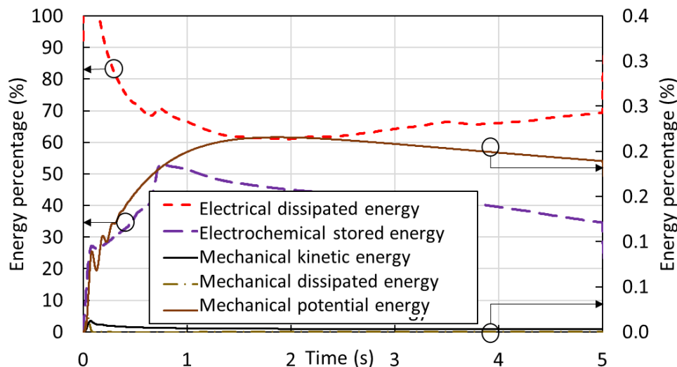
Fig.6 Couplage électrique / mécanique instantané.
