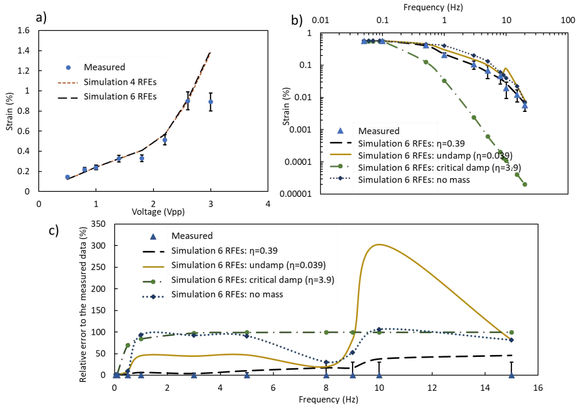
Fig.5 Comparaison entre les simulations et les expériences sur a) La déformation en fonction de l'amplitude de la tension appliquée à une fréquence constante de 0,1 Hz, b) La déformation en fonction de la fréquence de la tension appliquée à une valeur constante de \pm 1,1 V c) L'erreur relative des simulations comparée aux données mesurées.
