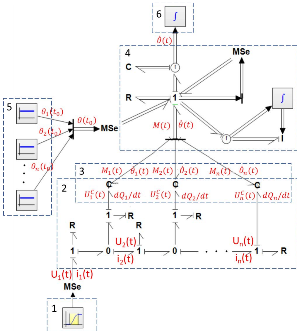
Fig.4 Modèle global de l'actionneur à base de polymère conducteur: 1. Source de tension, 2. Modèle électrochimique, 3. Couplage entre partie électrochimique et partie mécanique, 4. Modèle mécanique, 5. Conditions aux limites: contrainte initiale, 6. Déplacement de sortie.
