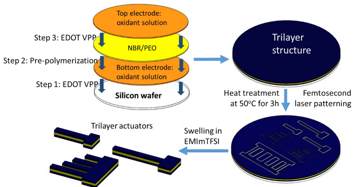
Fig.1 Procédé de fabrication d'un microactionneur montrant le processus multicouche suivi d'un micro-usinage au laser
