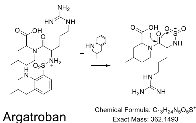
Figure 48 : deuxième voie de fragmentation de l'argatroban.
