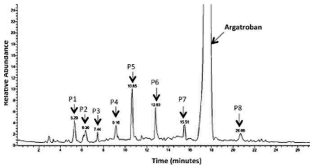
Figure 46 : chromatogramme total d'ions après exposition de l'argatroban à la lumière.
