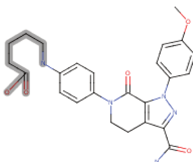
Figure 41 : alerte structurale(en gris) pour DP-4
