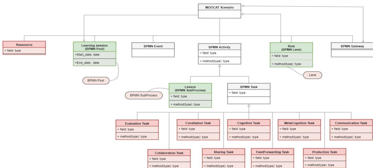
Figure 30 – Extension du méta-modèle BPMN
