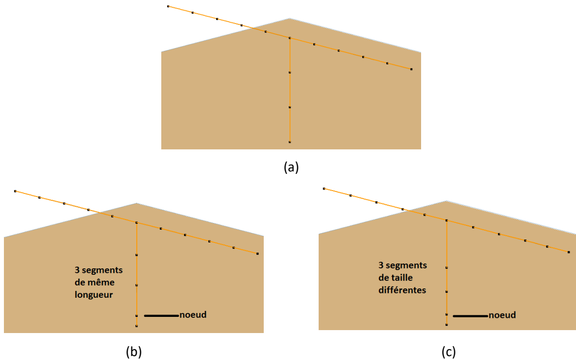
Figure 87 : Maillage fin généré avec FEKO pour l'antenne avec 1T : utilisé précédemment sans nœud permettant la liaison entre les T (a), régulier avec l'option « mesh smoothing » (b) et irrégulier sans l'option « mesh smoothing » (c)
