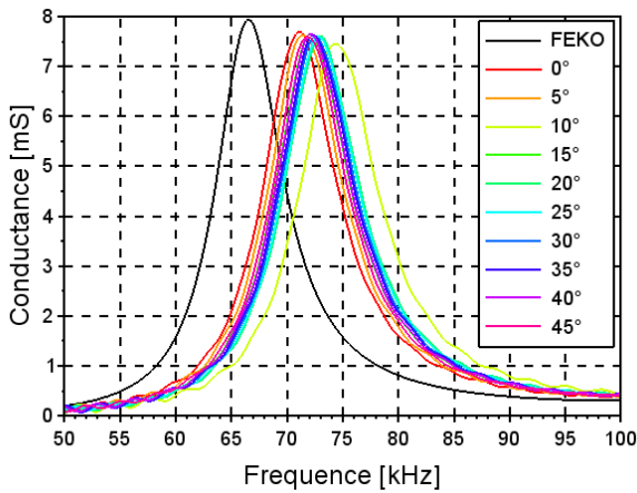
(a) Nœud sphérique
