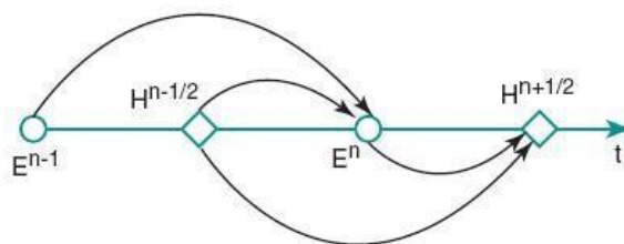
Figure 12 : Schéma « Leap-Frog » pour le calcul des champs
