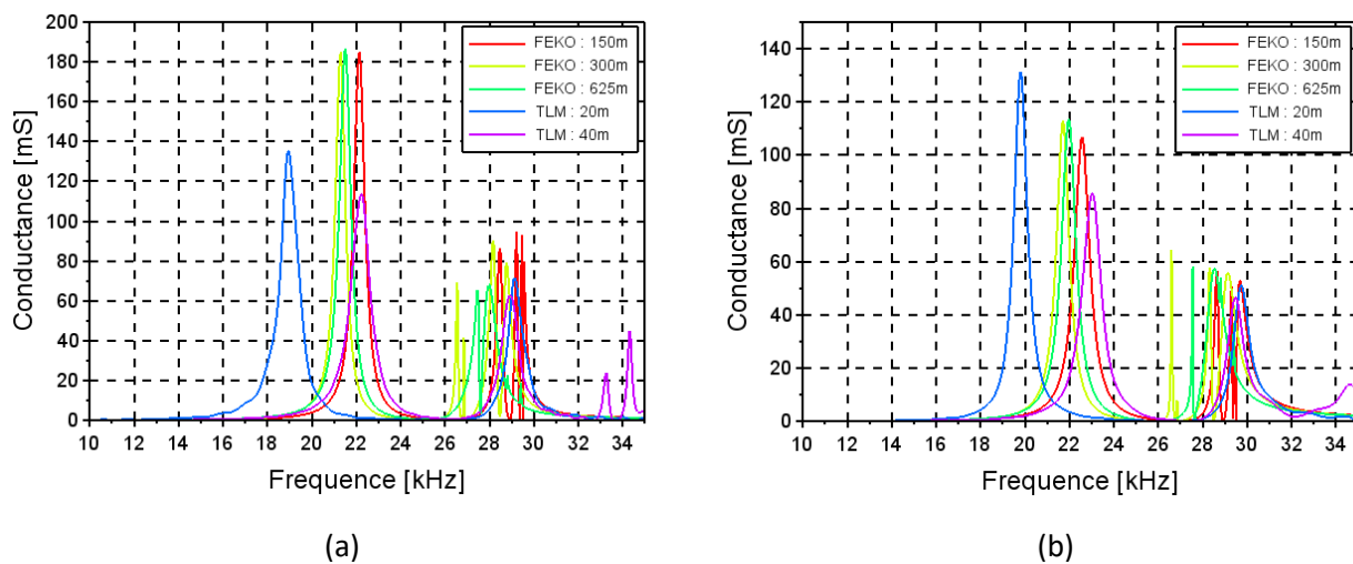
Figure 93 : Conductance de l'antenne simulée avec FEKO et avec la TLM pour différents maillages dans le cas d'une seule antenne alimentée (a) ou des deux antennes sont alimentées (b)
