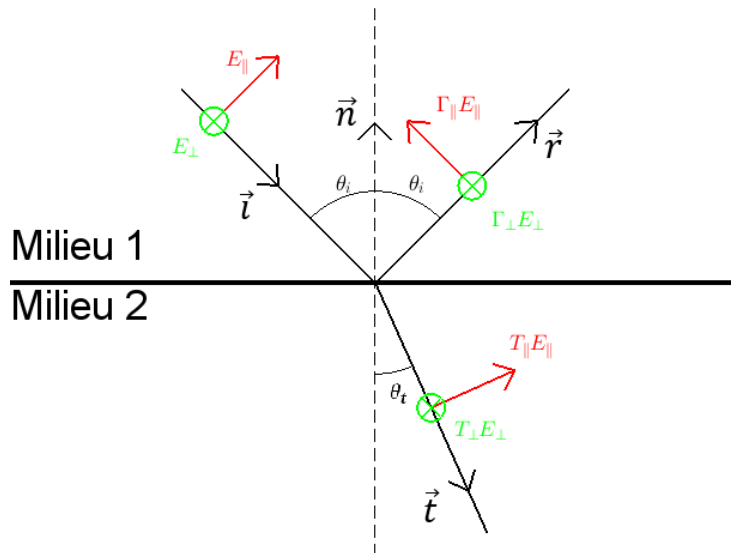
Figure 59 : Schéma du phénomène de réflexion et de réfraction d'une onde plane
