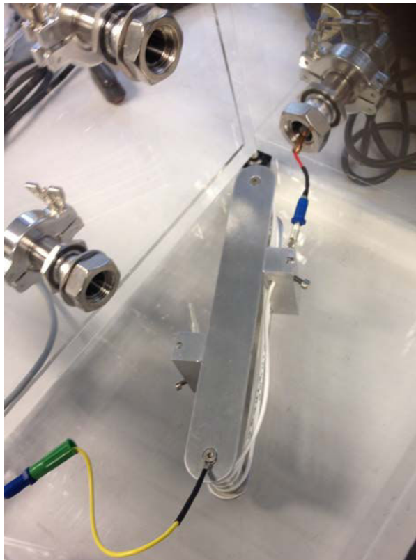
Figure II- 9: Support de vieillissement portant le câble introduit dans l'enceinte étanche pour mesures de décharges partielles
