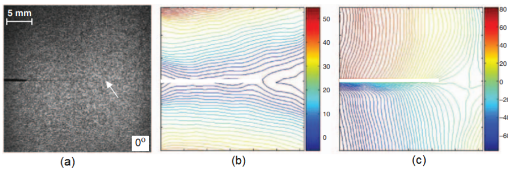
Figure 1.29 – (a) Photographie d'un échantillon avec des fibres orientées à 0° au cours de l'impact (28 \mu s après l'impact); la flèche indique l'avancement de la fissure et la zone noire correspond à la fissure initiale, (b) contours de déplacements perpendiculaires à l'impact (champ u) et (c) contours de déplacements suivant la direction de l'impact et l'ouverture de la fissure (champ v) - la barre de couleur indique les déplacements en \mu m [137]
