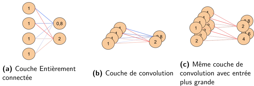
Figure 5.2 : Exemple d'équivalence entre une couche entièrement connectée et une couche de convolution. Le nombre de paramètres est le même, ici 4 * 2 , ils peuvent donc être copiés pour obtenir les mêmes résultats. On peut appliquer la convolution avec une entrée plus grande, en une seule passe.
