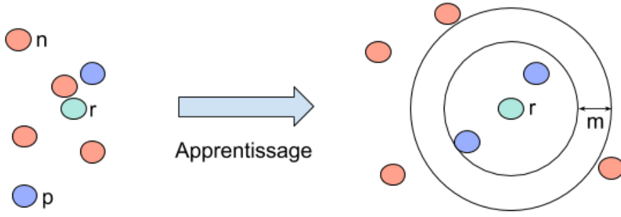
Figure 4.3 : Schéma de l'apprentissage du plongement des images, pour une image de références r , avec les images positives p représentant le même objet, et les images n qui contiennent des objets différents.
