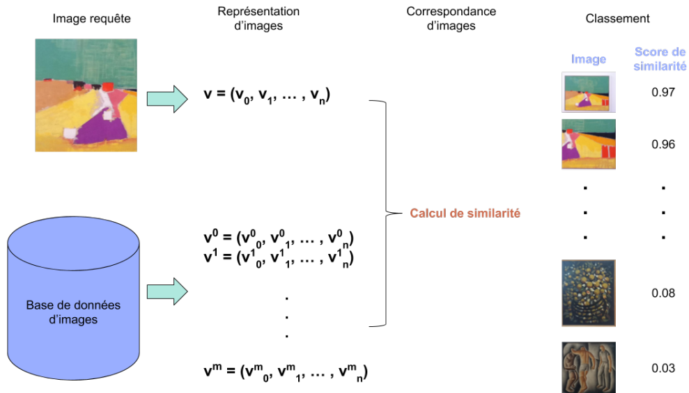
Figure 4.1 : Exemple fictif de recherche d'image par le contenu. Le classement représente la similarité entre les images.
