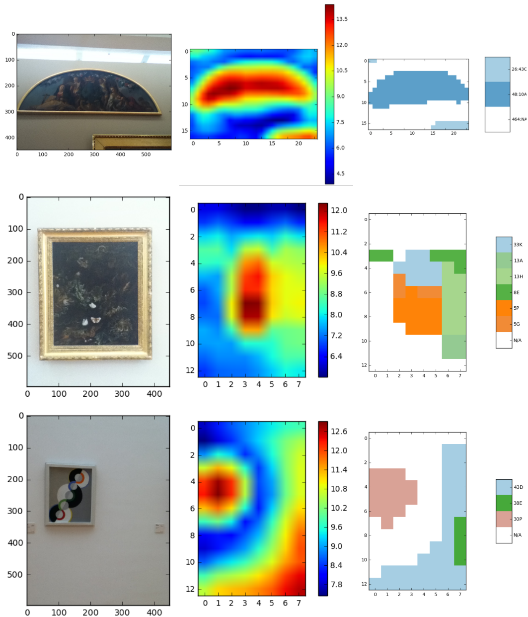
Figure 5.1 : Exemple d'images avec les heat-map des activations maximales, obtenues à partir d'un ResNet-152 après un apprentissage fin. Le réseau est appliqué sur toute l'image de manière strié. Les labels obtenus sur les zones d'activation maximales sont également indiqués.
