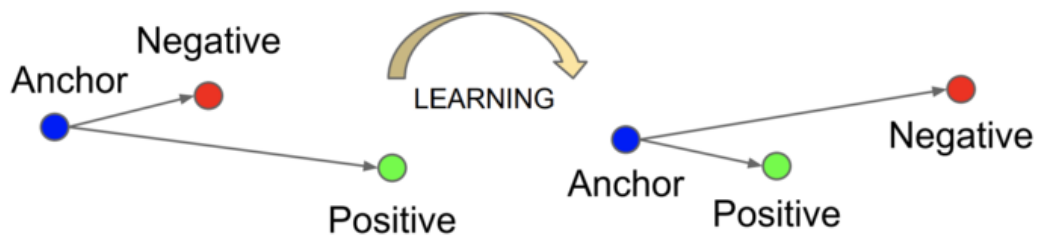
Figure 3.25 : Apprentissage des projection avec un réseau triple (source [15])
