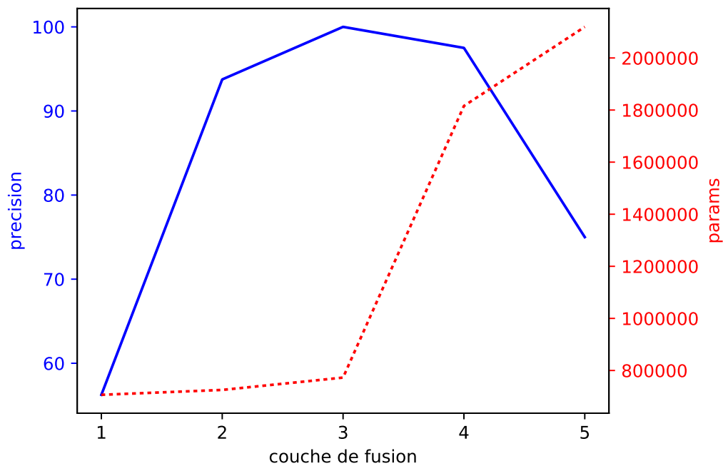
Figure 6.8 : Courbe d'évaluation de la position de la fusion.
