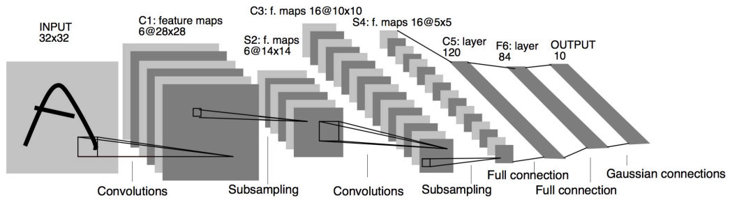
Figure 3.10 : Schéma du réseau profond LeNet [3]
