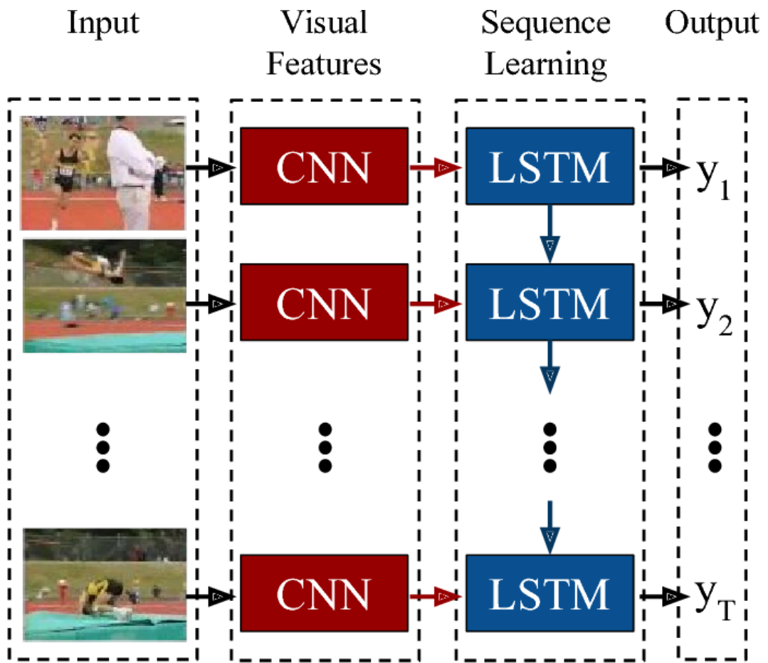
Figure 3.29 : Réseaux récurrents pour la détection d'action dans les vidéos à base de CNN et de LSTM (source [18])
