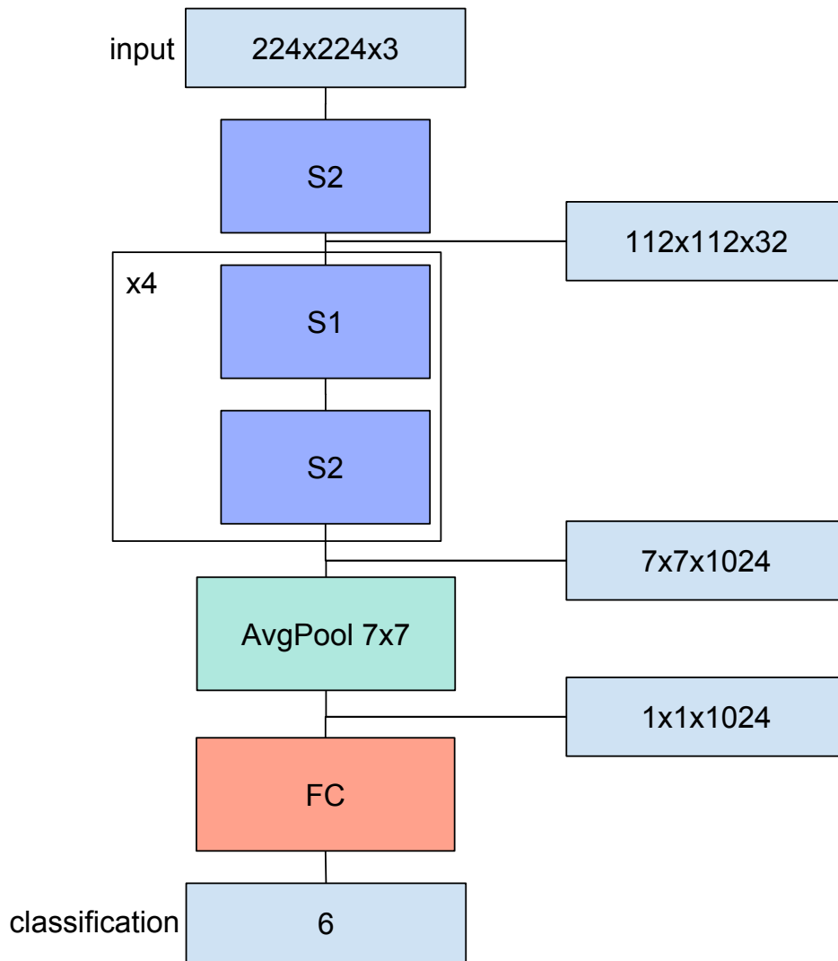
Figure 6.4 : Schéma du réseau proposé pour la reconnaissance de geste, avec entre chaque connexion la taille de la matrice de représentation des données.
