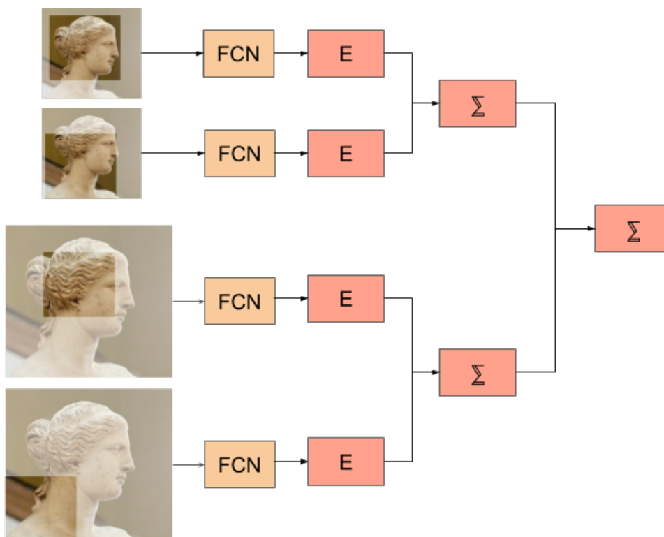
Figure 5.3 : Calcul de la fonction de coût lorsque l'on entraîne le réseau sur différentes régions à différentes échelles. L'entropie croisée E est calculé pour chaque segment d'image avant d'être moyenné (equation. 5.2).
