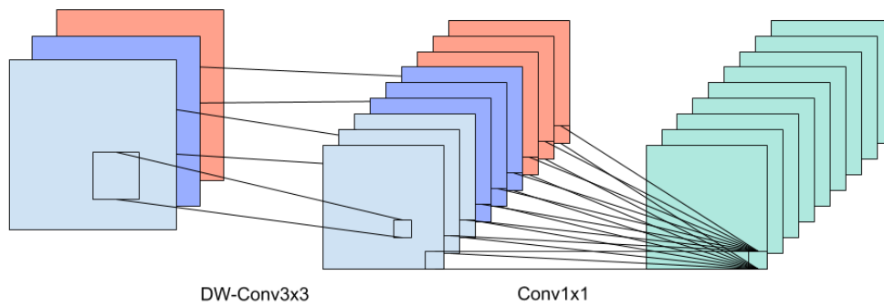
Figure 6.1 : Convolution 3 \times 3 DeepWise suivie d'une convolution 1 \times 1 qui fait office de fusion.
