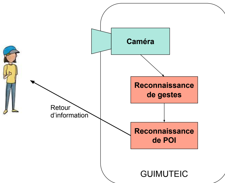
Figure 2.3 : Schéma d'organisation du système d'information GUIMUTEIC.
