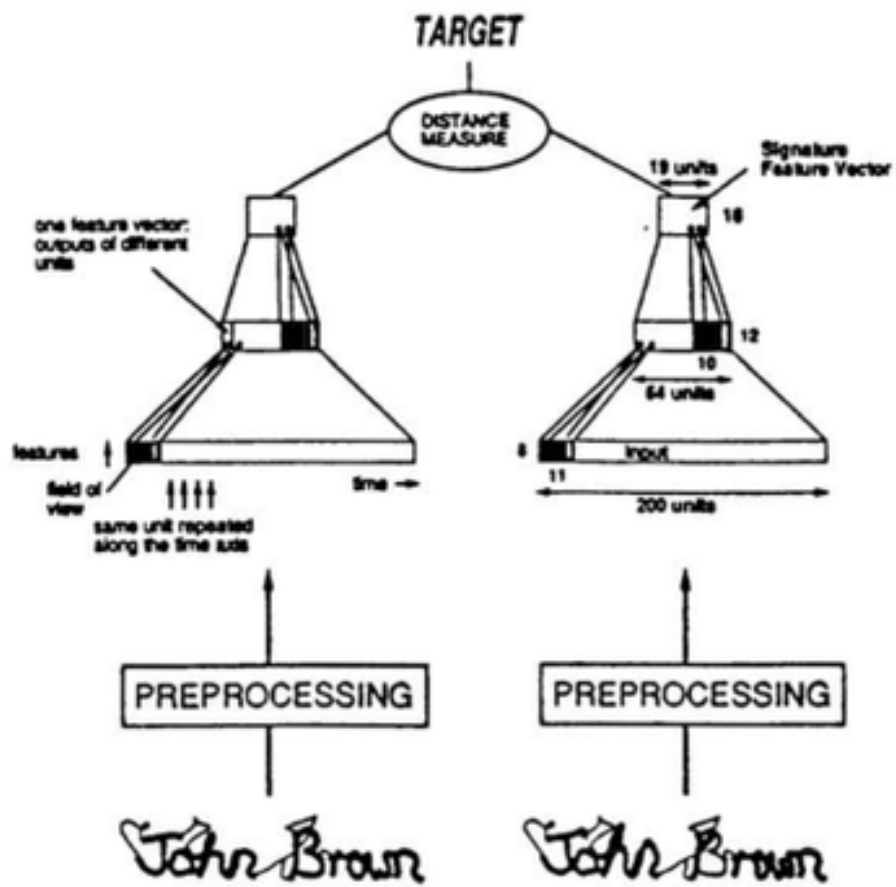
Figure 3.24 : Réseau siamois présenté par [14]
