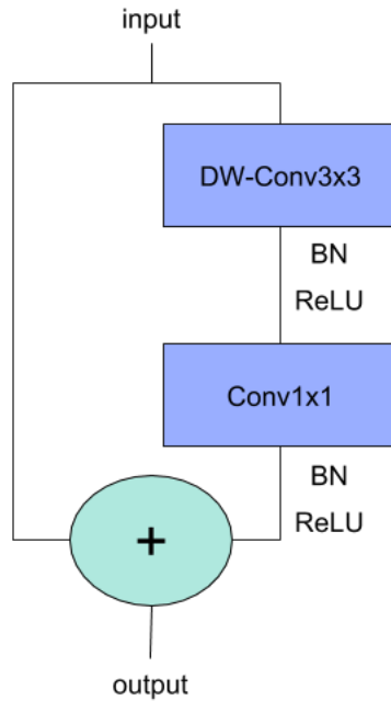
Figure 6.2 : Schéma du module S1.
