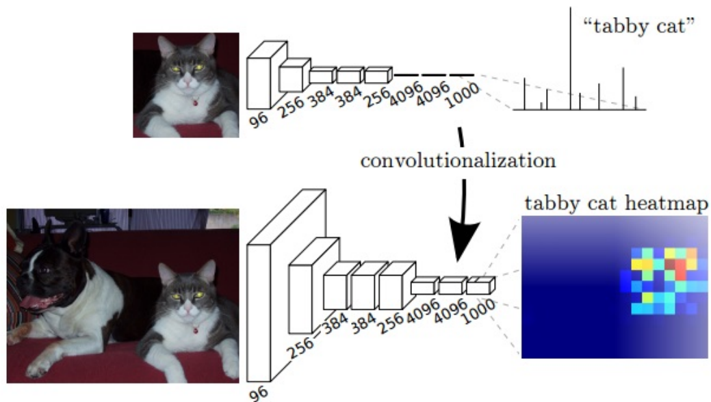
Figure 3.20 : Transformation d'une couche entièrement connectée en convolution pour obtenir une carte d'activation [12]
