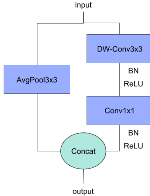
Figure 6.3 : Schéma du module S2.
