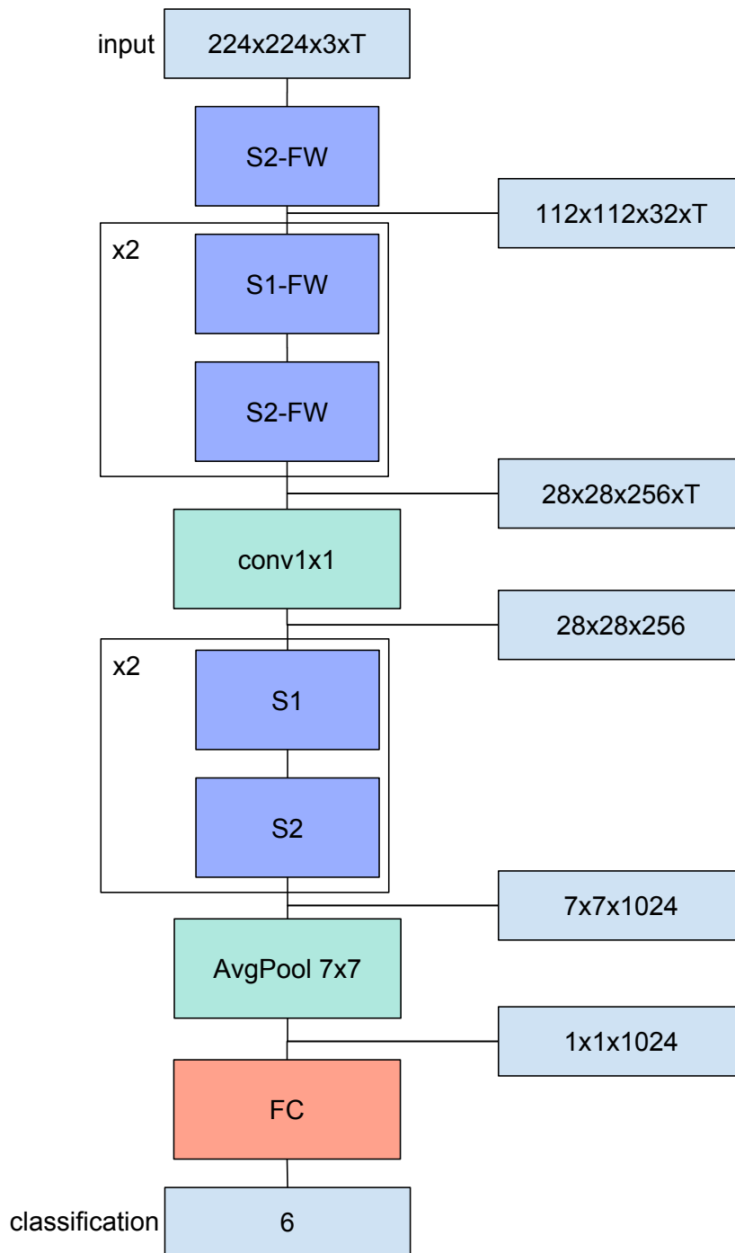
Figure 6.7 : Réseau proposé pour la détection de geste. Les premières couches sont sensibles à la trame (FrameWise), jusqu'à la fusion des N trames par une convolution 1 * 1 .
