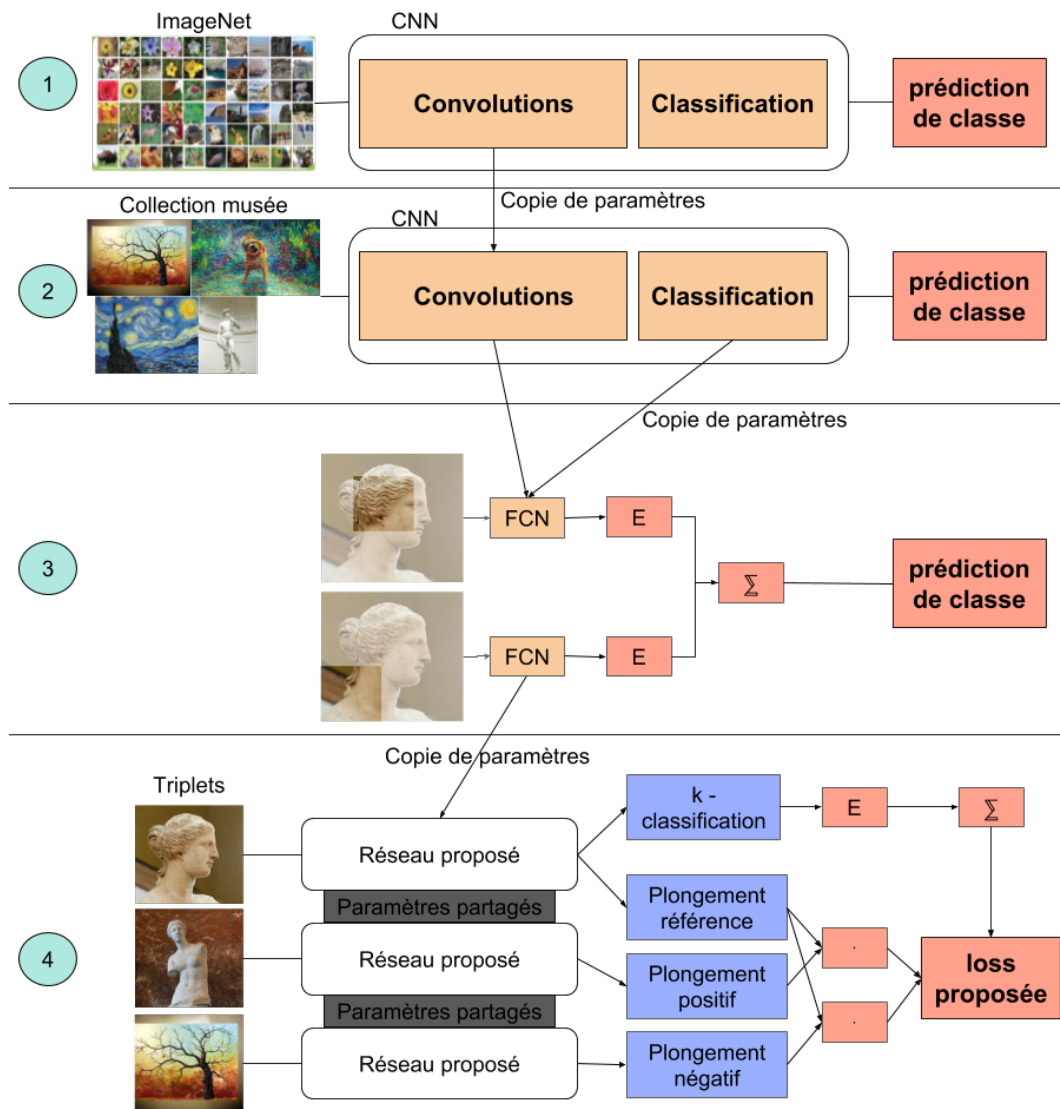
Figure 5.5 : Pipeline final d'apprentissage, avec l'ajout de la détection des régions d'intérêts.
