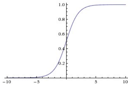
(a) Sigmoide
