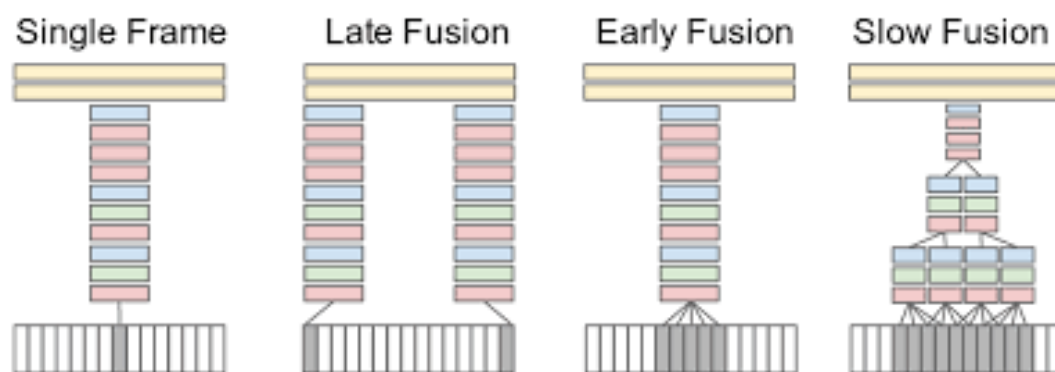
Figure 3.27 : Différentes méthodes de fusion d'information temporelle avec un CNN (source [16]).
