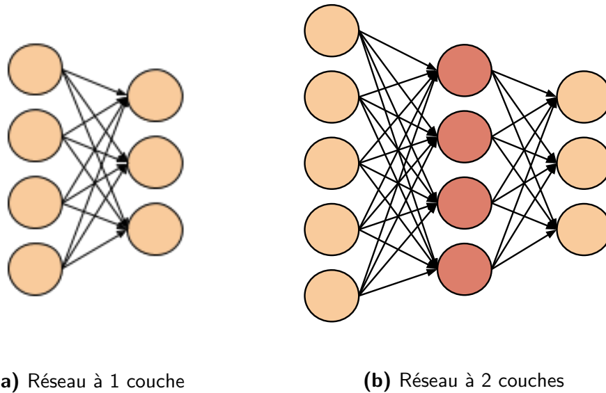
Figure 3.2 : Réseaux de neurones à 1 et 2 couches.
