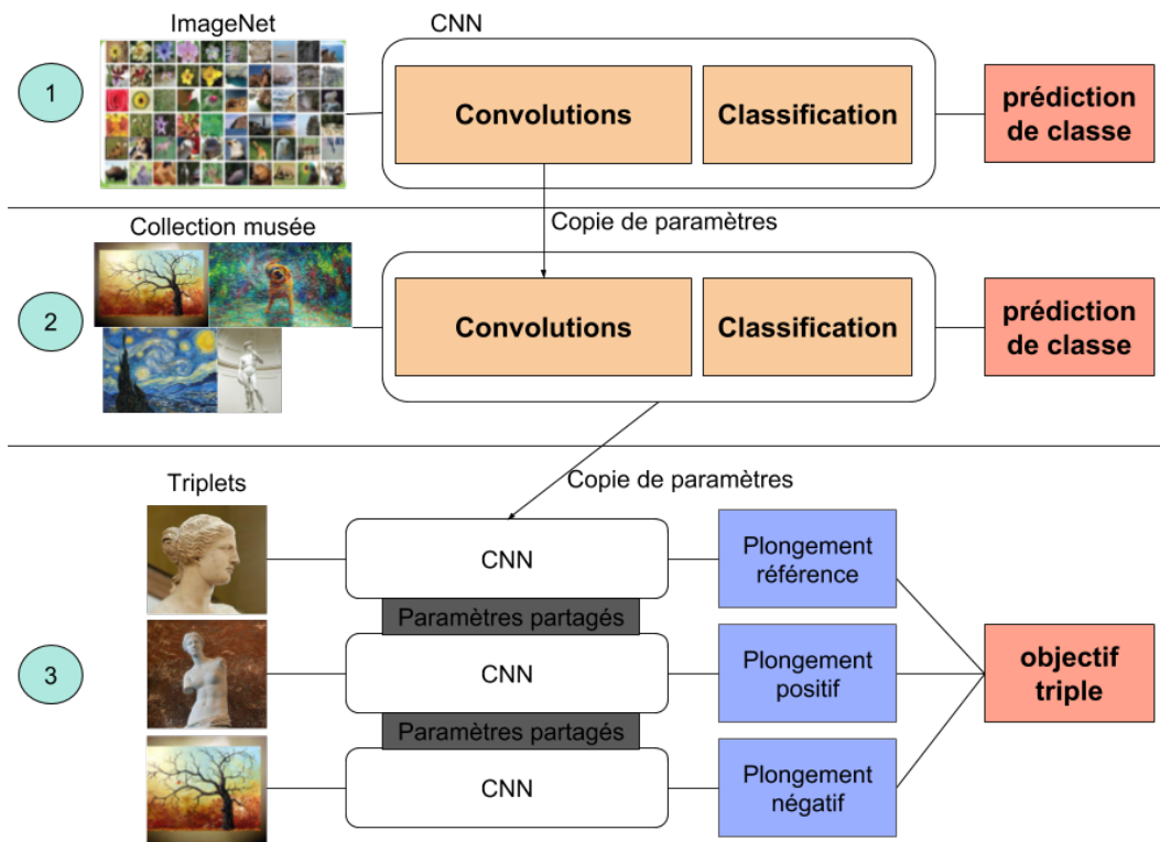
Figure 4.5 : Pipeline d'apprentissage. L'étape 1 correspond à l'apprentissage du réseau sur une grande collection d'image, ici ImageNet. L'étape 2 est le fine-tuning sur la collection du musée. La troisième étape consiste à apprendre à l'aide du réseau siamois triple.
