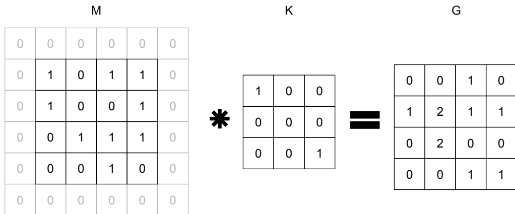
Figure 3.7 : Application d’une convolution 3x3 sur une matrice de taille 4x4 avec un padding de 1 et un pas de 1
