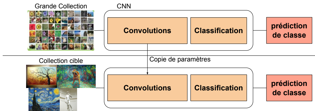
Figure 3.22 : Illustration du fine-tuning, avec apprentissage sur première collection et second apprentissage sur la collection cible.
