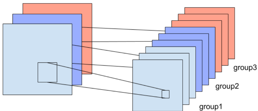
Figure 3.17 : Exemple de DeepWise Convolution ), avec trois groupes pour trois canaux d'entrée.
