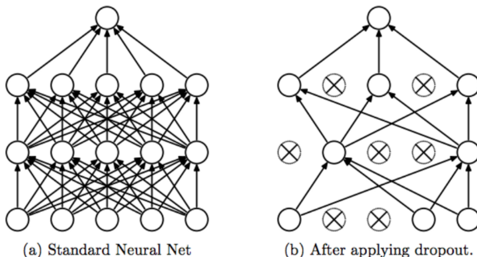
Figure 3.5 : Illustration du dropout pris depuis [2]
