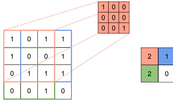
Figure 3.6 : Illustration d'une convolution sur une matrice 4 * 4 .
