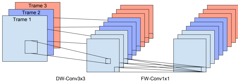
Figure 6.5 : Bloc de convolution utilisant DeepWise Convolution et FrameWise Convolution.
