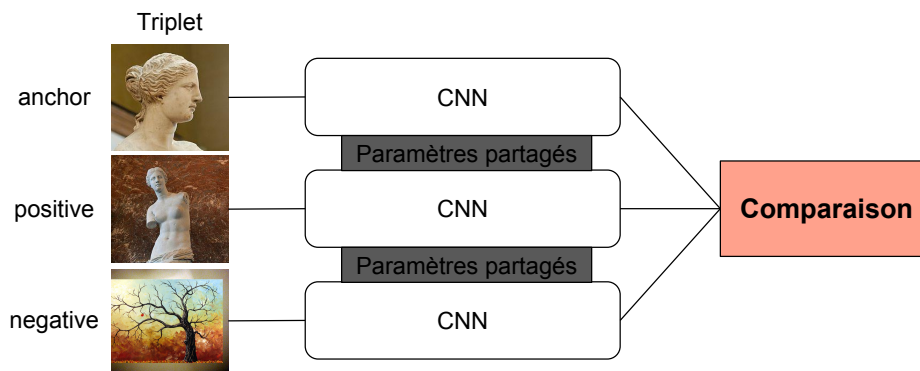
Figure 3.26 : Réseau siamois à trois branches
