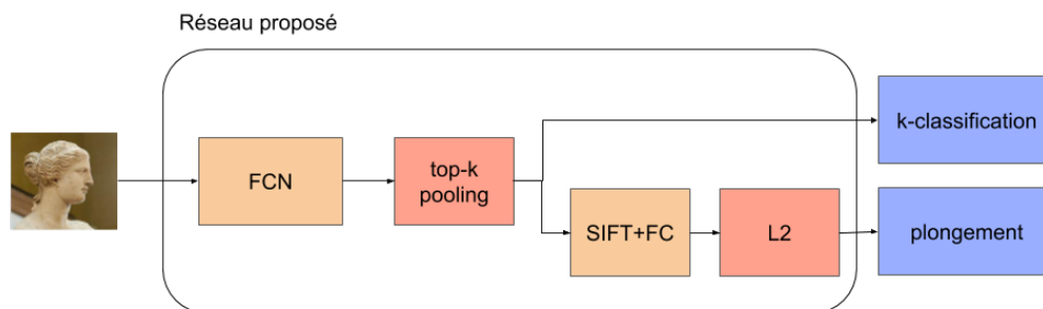
Figure 5.4 : Architecture du réseau proposé basé sur un réseau entièrement connecté pré-entraîné pour détecter les régions d'intérêt.
