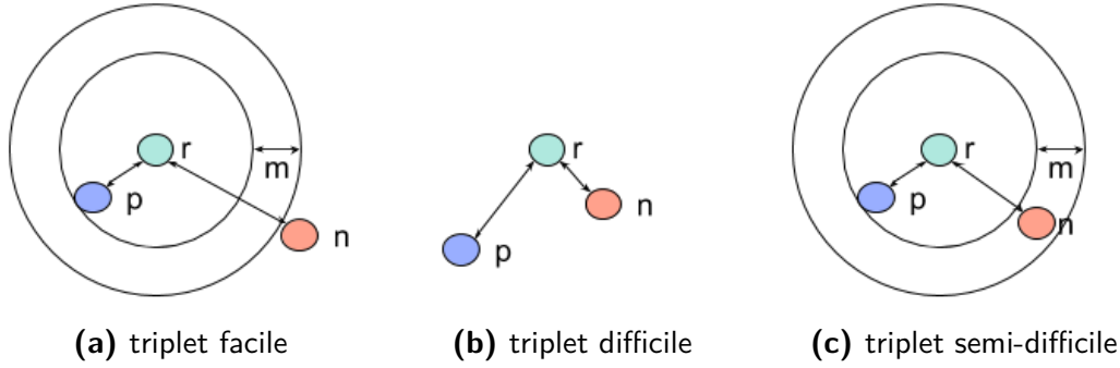
Figure 4.4 : Exemple des différentes configuration des projections possibles. La projection de l'image de référence r est plus ou moins proche des projection de l'image positive p ou de l'image négative n .
