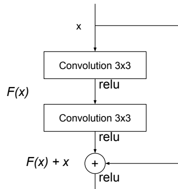
Figure 3.13 : Exemple d'un bloc résiduel de ResNet (source [6]).
