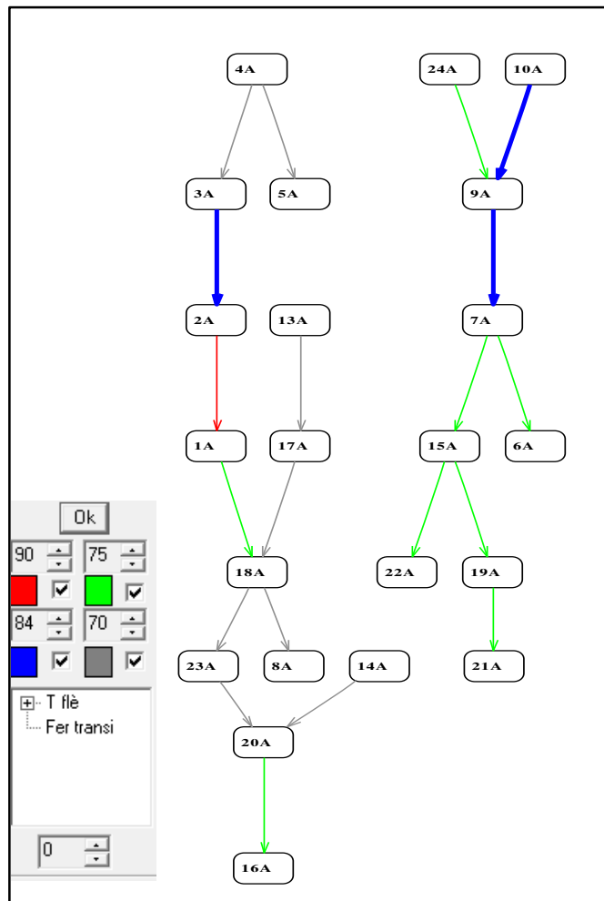
Image 3: Graphe implicatif - rapport au savoir mathématique au début de la scolarité
