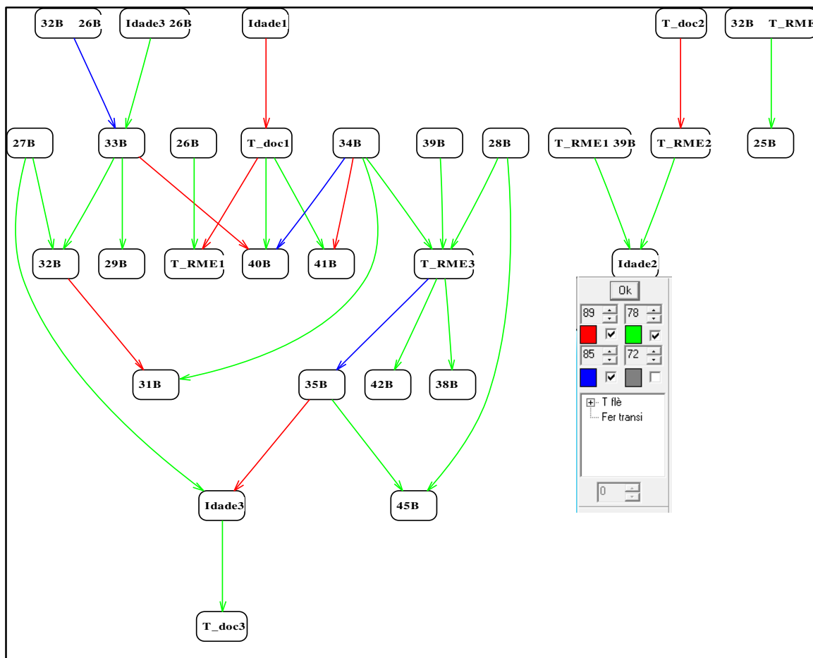
Image 6: Graphe implicatif - formation mathématique des professeurs
