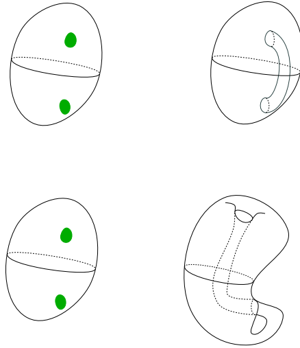
FIGURE 1.11 – La classe s ne détermine pas entièrement la chirurgie : il faut aussi connaître la trivialisaton du fibré normal d’un représentant de s .
