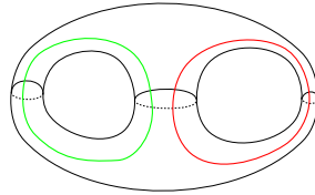
FIGURE 1.4 – La variété à bord \Sigma^{t+1} est le tore à deux anses plein et en rouge et vert sont représentées ses deux classes d'homologies non nulles.
