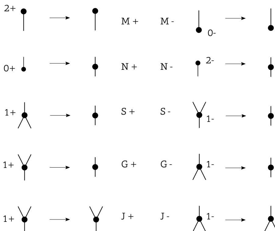
FIGURE 2.3 – Modèles locaux des transformations du graphe de Curley en le graphe de Reeb du double d’une éventuelle extension.
