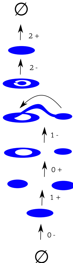
FIGURE 2.5 – Niveaux de la variété à bord V sur laquelle \tilde{f} s'étend sans points critiques.
