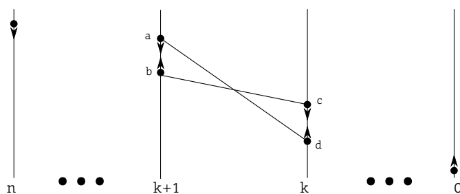
FIGURE 2.15 – Forme canonique du FMC de \tilde{f}_0 , quand \text{Car}(\mathbb{F}) \neq 5 .
