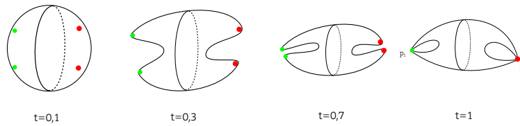
FIGURE 1.3 – Chemins \gamma et \gamma' associés à p_1 (en vert) et ceux associés à p_2 (en rouge) dans les variétés de niveaux.
