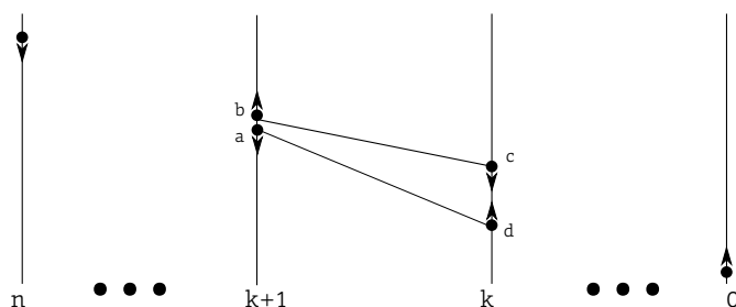
FIGURE 2.17 – Une autre modification possible de la forme canonique du FMC de \tilde{f}_0 .
