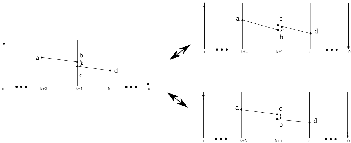
FIGURE 2.11 – Croisement de deux sommets de même indice.
