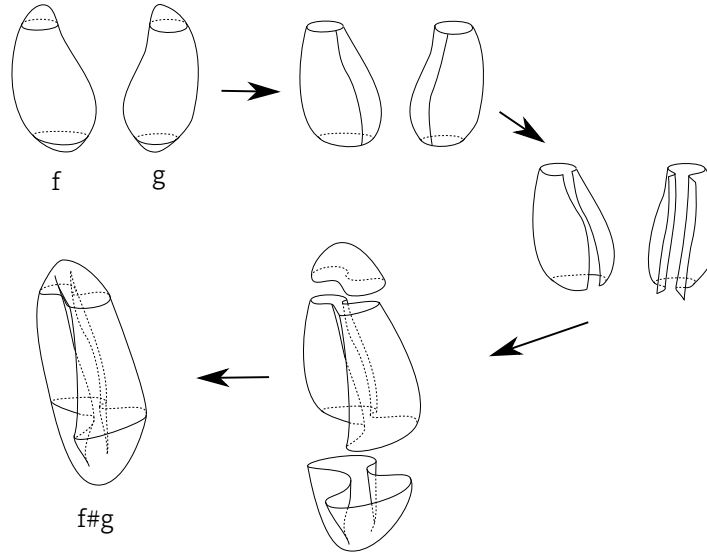
FIGURE 3.3 – Somme f\#g de deux fonctions de Morse ordonnées f et g . On enlève tout d’abord des voisinages des extremums de f et de g , puis on découpe chacune des sphères selon des lignes de gradients. On recolle les deux sphères sur les lignes de gradients, niveau par niveau avec une somme connexe. On rajoute enfin des calottes pour obtenir une sphère.
