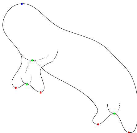
FIGURE 1.9 – La fonction hauteur sur ce plongement de la sphère représente une fonction de Morse sur un morse. Sont représentés en rouge les minimums, en vert les points selles et en bleu le maximum.
