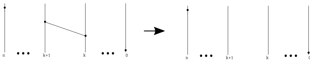
FIGURE 2.12 – Mort d'une paire de points critiques.
