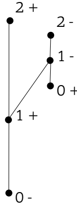
FIGURE 2.4 – Graphe de Curley d'un germe qui ne s'étend pas sur la boule sans points critiques.
