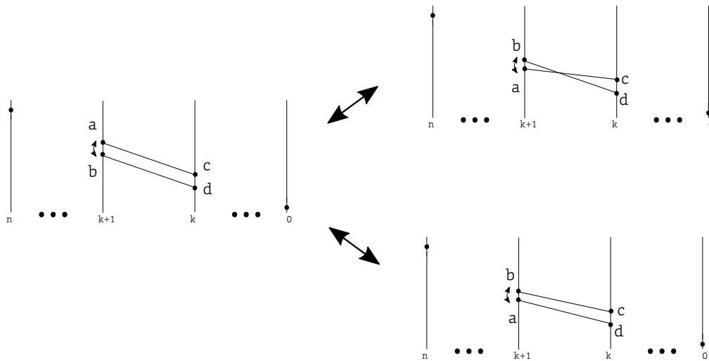
FIGURE 2.9 – Croisement de deux sommets de même indice.
