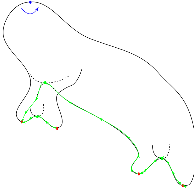
FIGURE 1.13 – Orientations des variétés instables des points d'indices 2 et 1. Les variétés instables des points d'indice 1 sont représentées dans leurs entières. Les variétés instables des points d'indice 0 ont l'orientation "+1". On rappelle que les lignes de gradients, elles, sont toujours orientées vers le bas.
