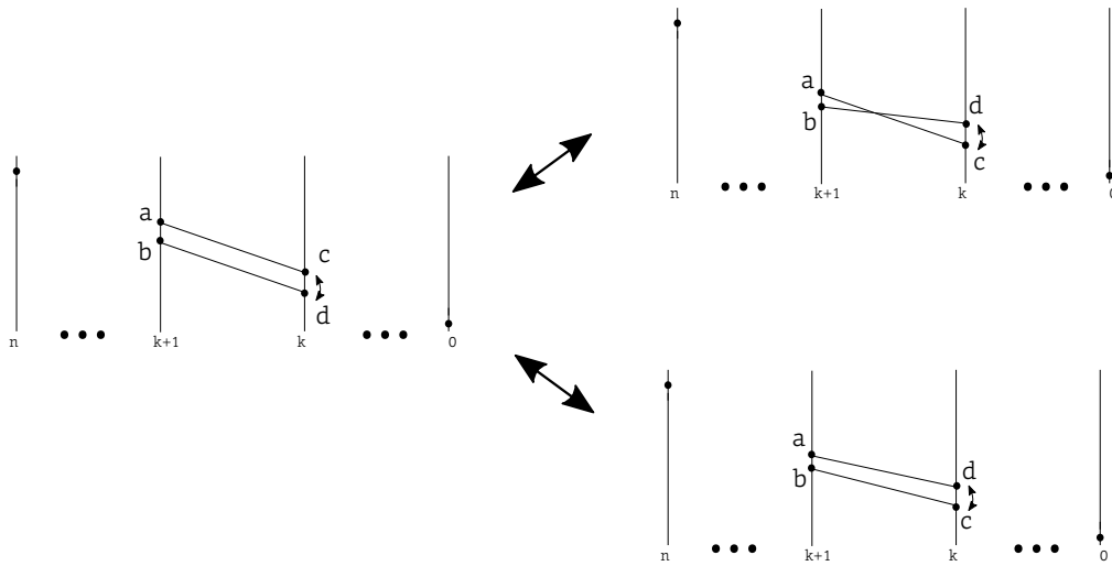
FIGURE 2.10 – Croisement de deux sommets de même indice.
