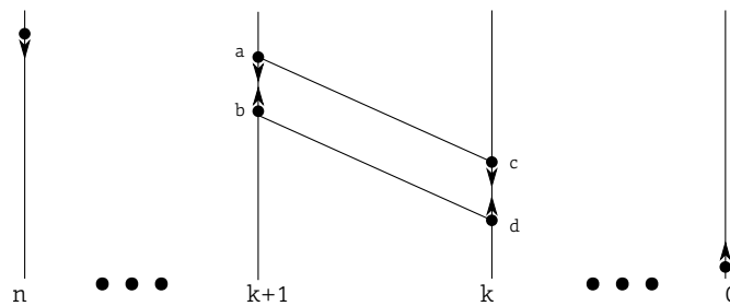
FIGURE 2.14 – Forme canonique du FMC de \tilde{f}_0 , quand \text{Car}(\mathbb{F}) = 5 .
