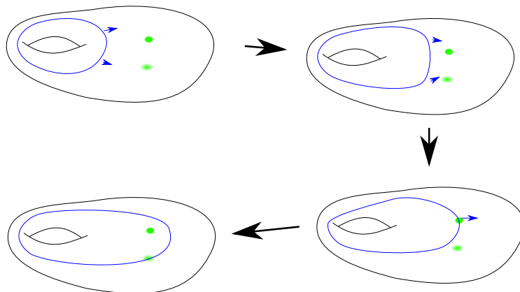
FIGURE 1.18 – Réalisation du glissement d’anses de s_1 au-dessus de s_2 , effet dans la variété de niveau entre s_1 et s_2 .
