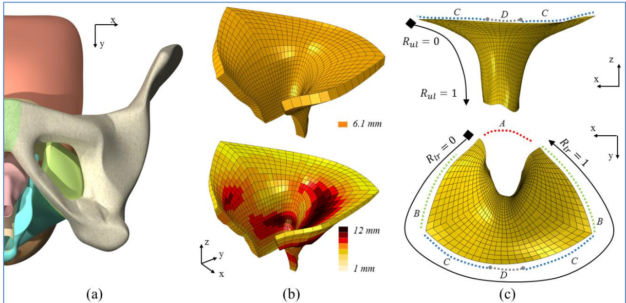
Figure 21- Modèle surfacique du LAM et maillage. Reconstruction à épaisseur constante et épaisseur variable a) Modèle numérique 3D b) Maillage du LAM avec épaisseur constante (en haut) et variable (en bas) c) Repérage des points de référence pour la localisation des déformations
