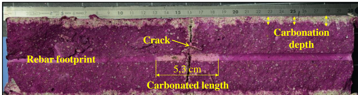
Figure 2 : Estimation de la longueur d'endommagement de l'interface acier/liant
