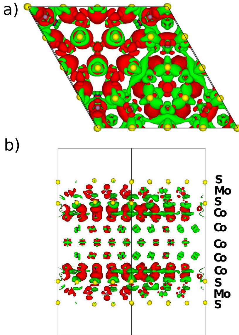
FIGURE 4.16: Vue de dessus (a) et vue de côté (b) du transfert de charge des électrons de spin minoritaire \Delta_{n\downarrow} , à l'interface de la supercellule. Les valeurs positives et négatives sont indiquées en rouge et en vert respectivement. Les sphères jaune, violet clair et bleu (lorsqu'elle sont visibles) indiquent respectivement la position des noyaux de S, de Mo et de Co.
