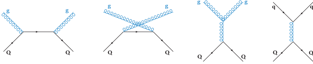
FIGURE II.9 – Diagrammes de Feynman à l’ordre dominant (LO) de la diffusion d’un quark lourd avec un parton léger.
