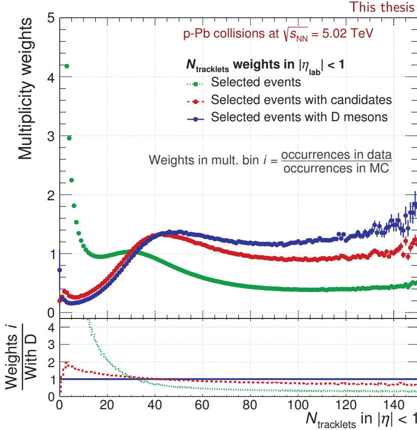
FIGURE V.20 – Poids en multiplicité pour diverses classes d’événements réels p–Pb à \sqrt{s_{NN}} = 5,02 TeV, en fonction du nombre de tracklets dans |\eta_{\text{lab}}| < 1 : événements sélectionnés (vert), événements sélectionnés avec des candidats D (rouge), événements sélectionnés avec des mésons D (bleu). Voir texte.
