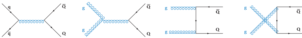
FIGURE II.2 – Diagrammes de Feynman à l'ordre dominant (LO) pour la production d'une paire de quarks lourds Q\bar{Q} .
