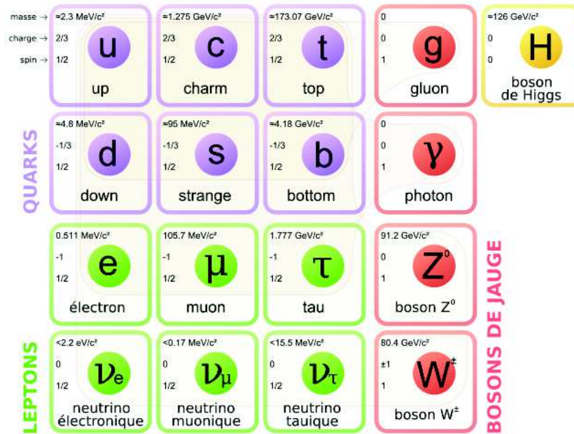
FIGURE I.1 – Famille des particules élémentaires du modèle standard de la physique des particules [4].
