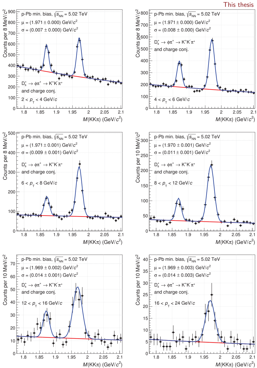
FIGURE IV.17 – Spectres de masse invariante M(K^\pm K^\mp \pi^\pm) ajustés pour chaque intervalle en impulsion transverse utilisé dans les collisions p-Pb de biais minimum à \sqrt{s_{NN}} = 5,02 TeV. Le pic de droite est celui du D_s^+ , le pic de gauche est celui du D^+ .
