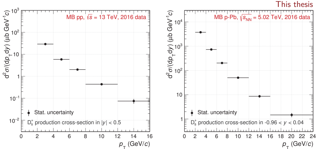
FIGURE IV.28 – Section efficace différentielle de production des mésons \text{D}_s^+ en fonction de leur impulsion transverse, pour les collisions pp à \sqrt{s} = 13 TeV (gauche) et p-Pb à \sqrt{s_{\text{NN}}} = 5,02 TeV (droite).
