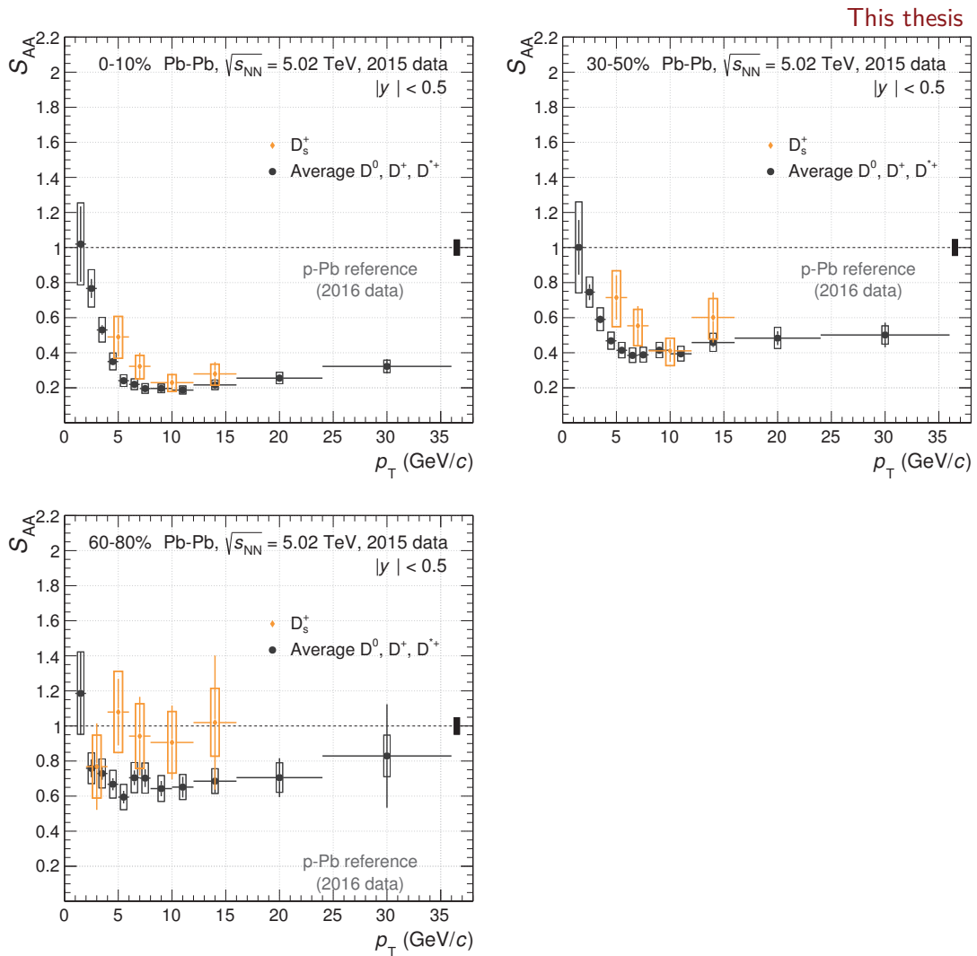
FIGURE VI.17 – Comparaison des observables S_{AA} des mésons D_s^+ prompts et des D^0 , D^+ et D^{*+} prompts moyennés, dans les collisions Pb–Pb à \sqrt{s_{NN}} = 5,02 TeV pour trois classes de centralité différentes : 0–10%, 30–50% et 60–80%. La boîte noire à S_{AA} = 1 représente l'incertitude sur la normalisation ( \mathcal{L}_{\text{int}}^{\text{p-Pb}} et \langle T_{AA} \rangle^{\text{cent}} ).
