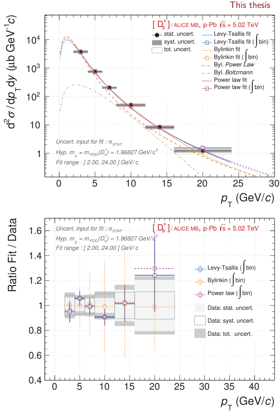
FIGURE VI.10 – Haut : ajustement de la section efficace différentielle de production des mésons D_s^+ , dans les collisions p-Pb à \sqrt{s_{\text{NN}}} = 5,02 \text{ TeV} , par une loi de puissance, une fonction de Tsallis-Lévy et de Bylinkin. Pour cette dernière, les contributions des termes exponentiels (Boltzmann) et loi de puissance sont présentées. Bas : Rapport de l'intégrale des courbes ajustées aux données, par intervalle d'impulsion transverse.
