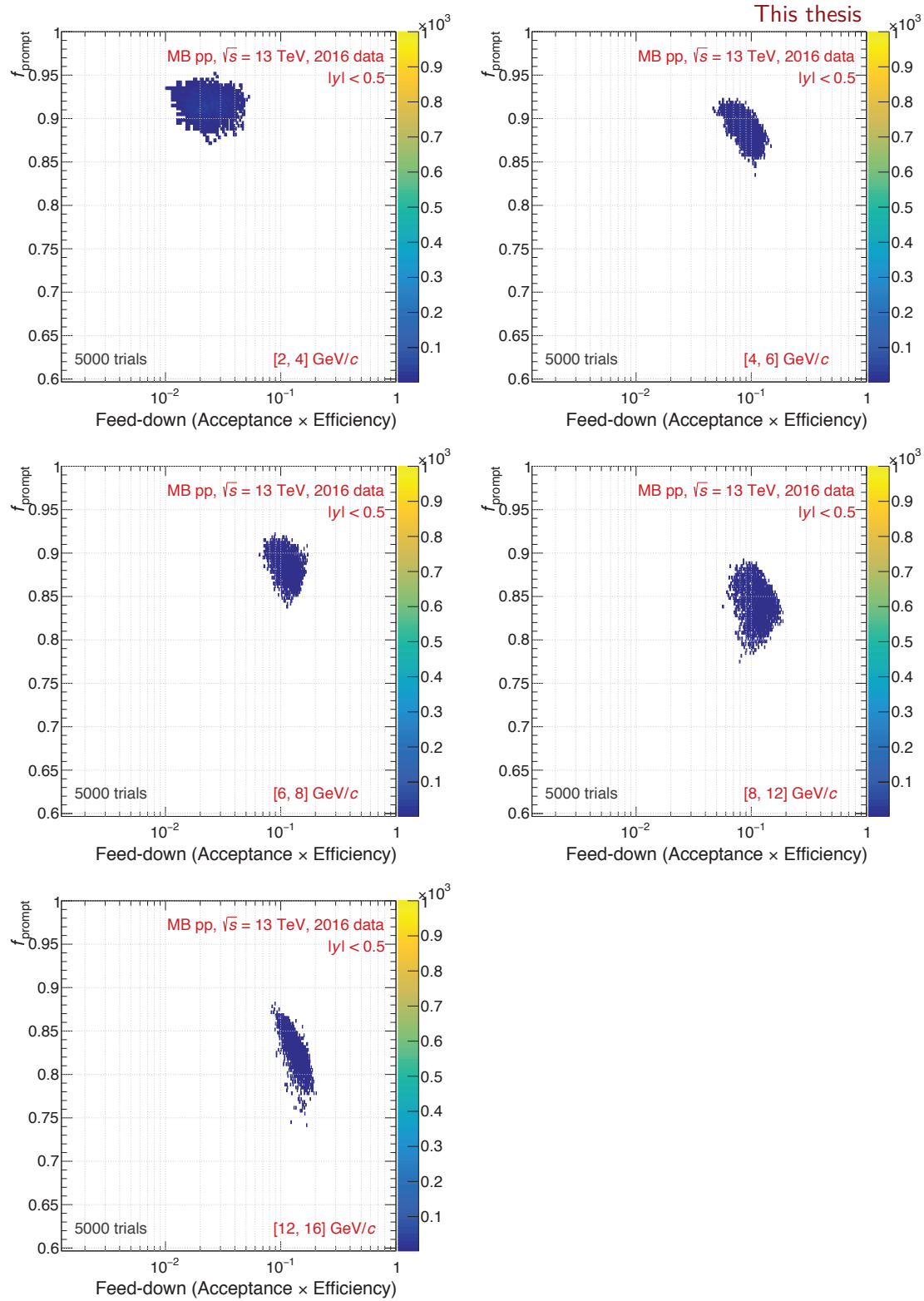
FIGURE IV.27 – Fraction de mésons D_s^+ prompts en fonction des termes \text{Acc} \times \text{Eff} des D_s^+ non-prompts, pour chaque intervalle d'impulsion transverse, dans les collisions pp à \sqrt{s} = 13 \text{ TeV} , avec la méthode statistique à 5 000 jeux de coupures.
