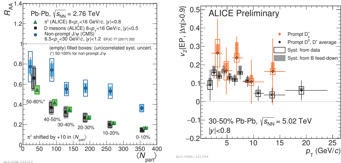
FIGURE II.11 – Gauche : facteurs de modification nucléaire des mésons \pi^\pm , D et J/\psi \leftarrow B en fonction de \langle N_{\text{part}} \rangle dans les collisions Pb–Pb à \sqrt{s_{\text{NN}}} = 2,76 TeV [115]. Droite : écoulement elliptique des mésons D^0 et D^+ (moyennés) et D_s^+ pour la classe de centralité 30–50% dans les collisions Pb–Pb à \sqrt{s_{\text{NN}}} = 5,02 TeV [114].
