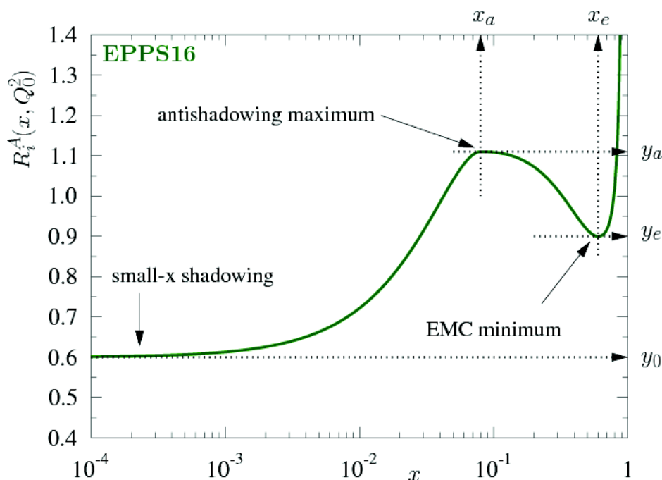
FIGURE II.7 – Exemple de facteur de modification nucléaire R_i^A , de paramétrisation EPPS16 [83] évaluée à Q_0^2 = (1,3 \text{ GeV})^2 .
