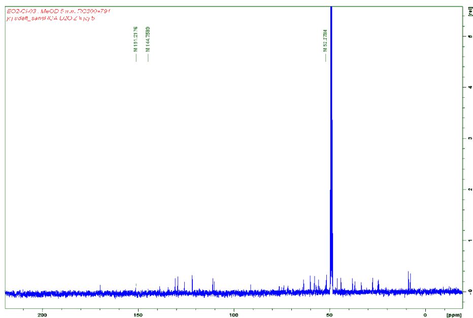
Spectre RMN ^{13}\text{C} de l'hydrogénosulfate-criophylline ( 3 ) (MeOH \text{d}_4 , 100 MHz)
