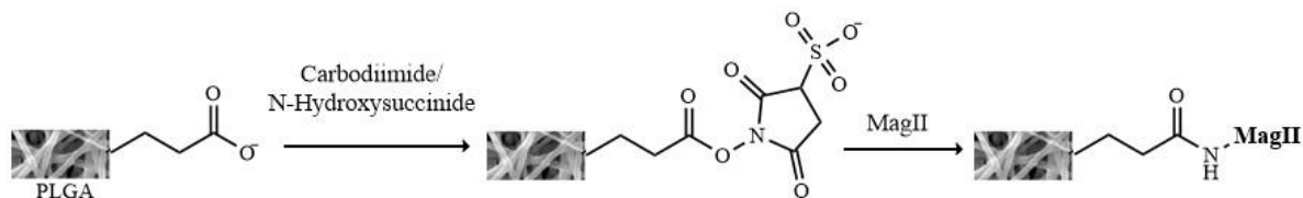
Figure 37: Schéma de l'immobilisation de la Magainine II sur les fibres de PLGA [81]
