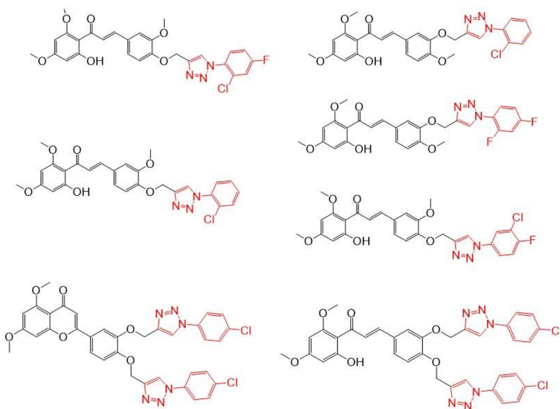
Figure 88: Molécules possédant les meilleures activités antibactériennes [153]
