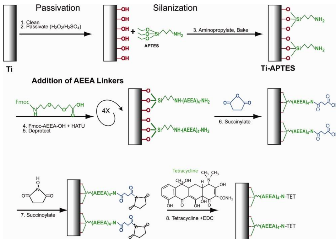
Figure 7: Schéma de couplage de la tétracycline à une surface de titane [37]
