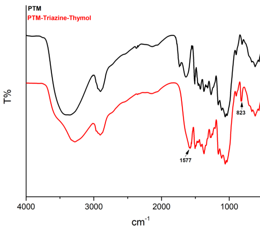
Figure 70: Spectre IR de la pâte thermomécanique et du matériau PTM-Triazine-Thymol
