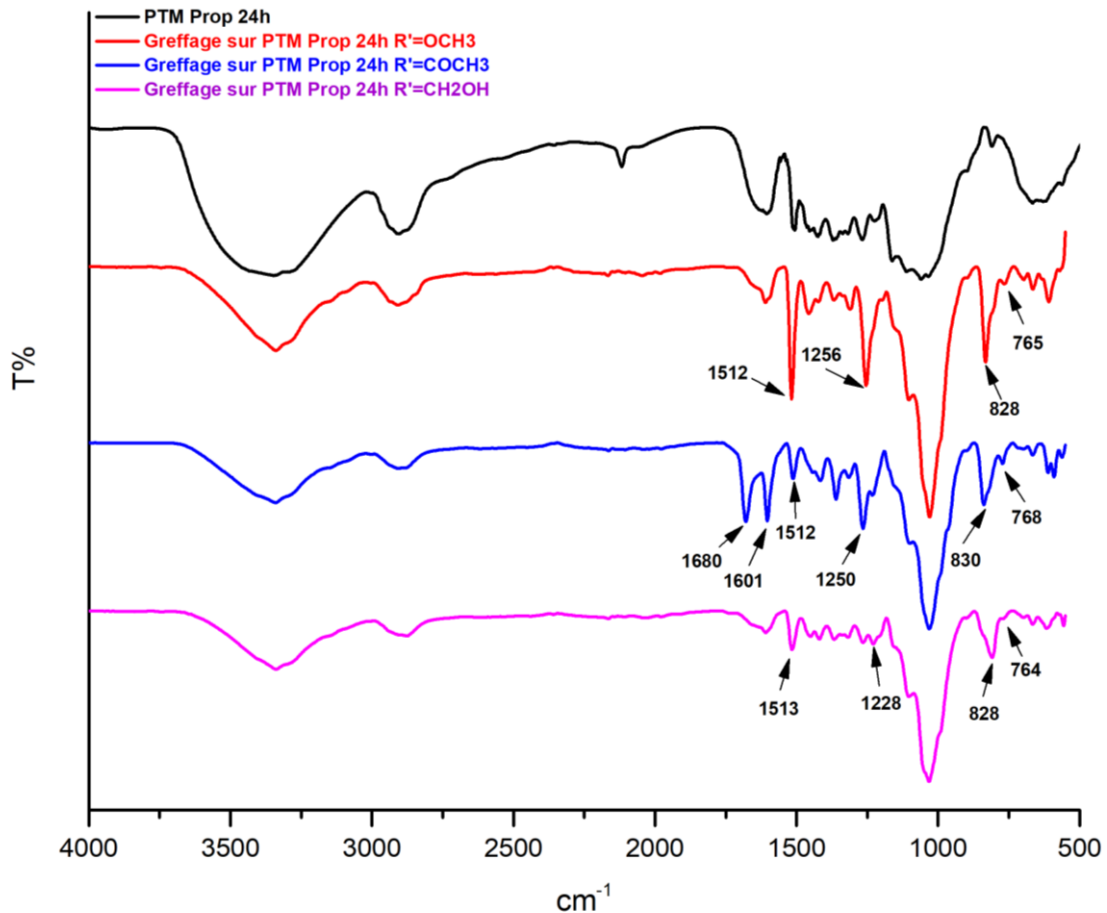
Figure 124: Spectre IR de la pâte thermomécanique propargylée après 24h et des matériaux portant les substituants méthoxyle, acétyle et hydroxyméthyle
