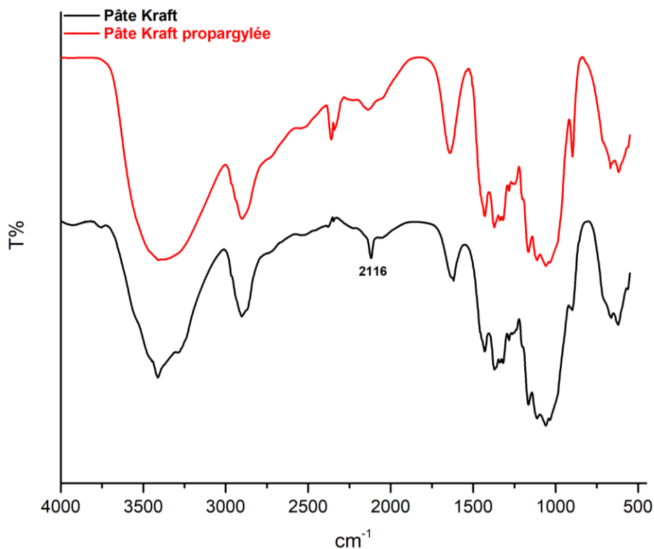
Figure 102: Spectre IR de la pâte Kraft non modifiée et la pâte kraft propargylée
