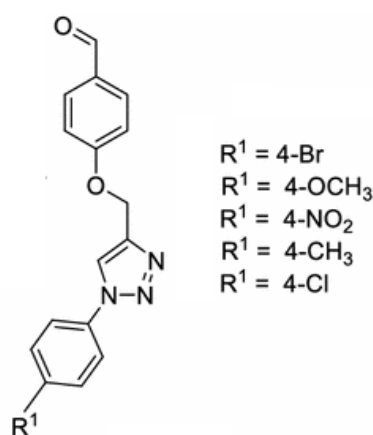
Figure 111: Les différents dérivés triazolés synthétisés [175]
