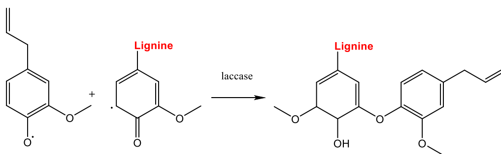
Figure 45: Greffage d'eugénol sur les fibres de coco [112]
