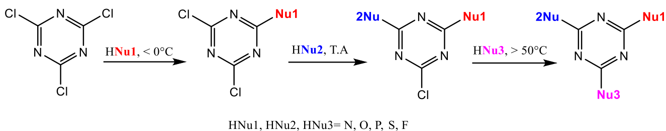
Figure 47: Réactivité thermo-dépendante du chlorure cyanurique
