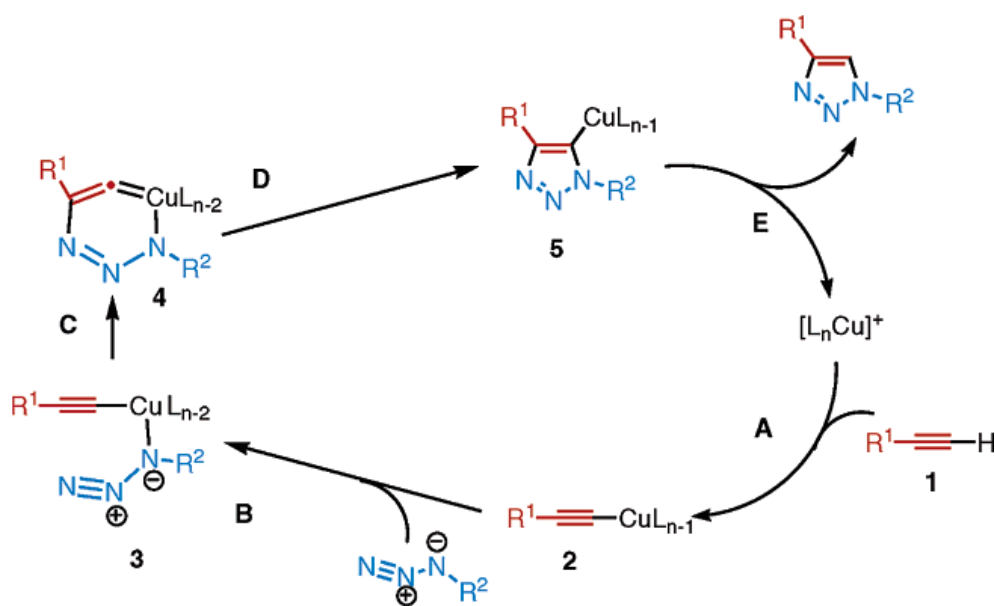
Figure 82: Mécanisme de cycloaddition 1,3-dipolaire azoture/alcyne catalysée par le cuivre
