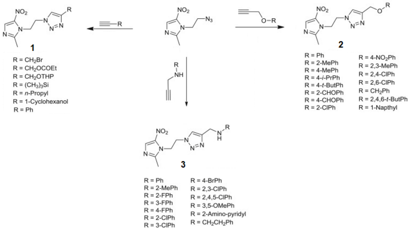
Figure 90: Schéma de synthèse des drivés de métronidazole [154]
