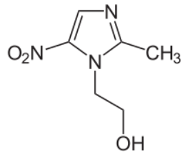
Figure 89: Structure de métronidazole
