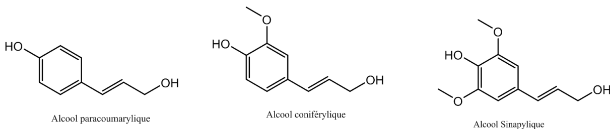
Figure 27: Structure des trois principaux constituants de la lignine
