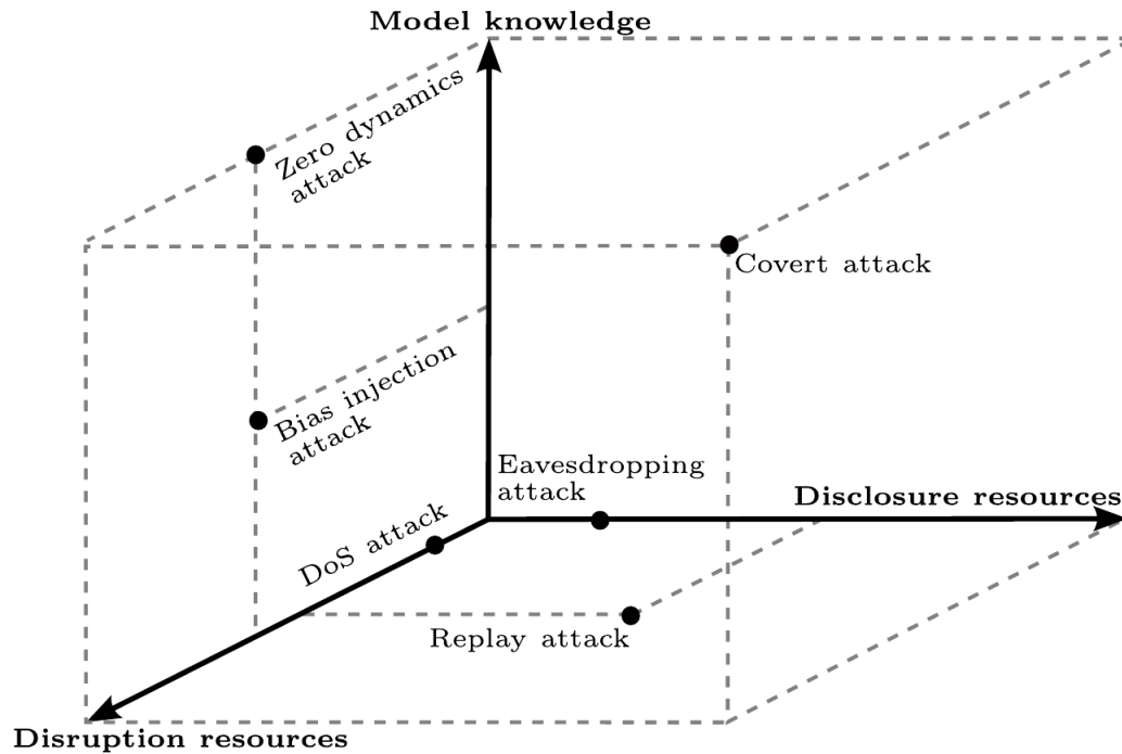
Figure 2: Différents tyoes d’attaques visant les CPS [82]
