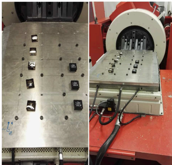
Figure 4-25 :Essai de vibration selon l'axe X
