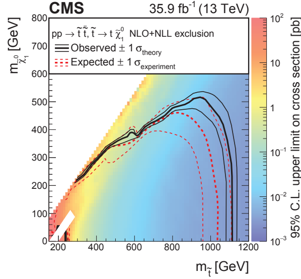
Figure A.11: Les limites d'exclusion à 95% CL sur le modèle T2tt correspondant à une luminosité intégrée de 35.9 \text{ fb}^{-1} . L'interprétation est fournie dans le plan de la masse du stop par rapport à la masse du neutralino. Le code de couleur indique la limite supérieure de 95 % CL sur la section efficace en supposant un rapport de branchement de 100% pour \tilde{t}_1 \rightarrow t\tilde{\chi}_1^0 . Les contours rouge et noir représentent respectivement les limites d'exclusion attendues et observées. La zone sous la courbe épaisse noire indique la région exclue des points de signal.
