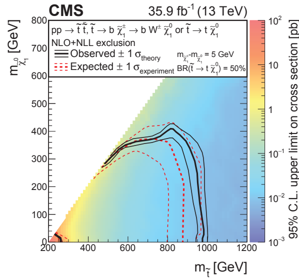
Figure A.13: Les limites d'exclusion à 95% CL sur le modèle T2tb correspondant à une luminosité intégrée de 35.9 fb -1 . L'interprétation est fournie dans le plan de la masse du stop par rapport à la masse du neutralino. Le code de couleur indique la limite supérieure de 95% CL sur la section efficace en supposant un rapport de branchement de 50% pour \tilde{t}_1 \rightarrow t\tilde{\chi}_1^0 et 50% pour \tilde{t}_1 \rightarrow b\tilde{\chi}_1^\pm . Les contours rouge et noir représentent respectivement les limites d'exclusion attendues et observées. La zone sous la courbe épaisse noire indique la région exclue des points de signal.
