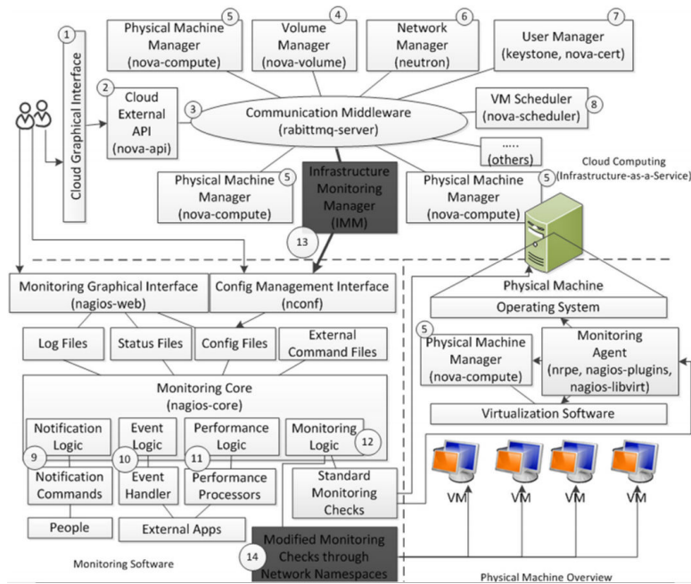
FIGURE 2.8 – Architecture de IaaS Mon [GUTIERREZ-AGUADO et al. 2016] (IMM (13) intercepte les communications entre les services d’Openstack et CMC (13) intercepte les names spaces utilisés au niveau des machines physiques)
