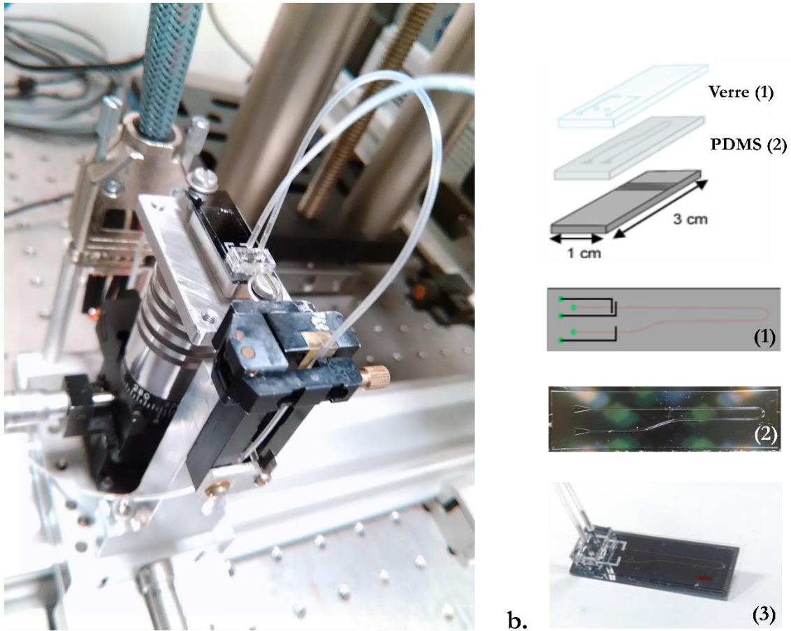
Fig. 4 – a. Puce optofluidique montée avec le système de fluide sur le porte-échantillon. b. Système de microfluidique développé permettant l'injection de fluide et l'arrêt du flux (vannes). Une lamelle de verre dans laquelle sont usinés des canaux à air comprimé est déposée sur une couche de PDMS dans laquelle se trouve un canal épais de 10 \mu\text{m} et large de 200 \mu\text{m} . (1) Dessin des canaux gravés dans la lamelle de verre. (2) Moule en résine permettant de fabriquer les canaux dans le PDMS. La puce optofluidique complète est montrée en (3).
