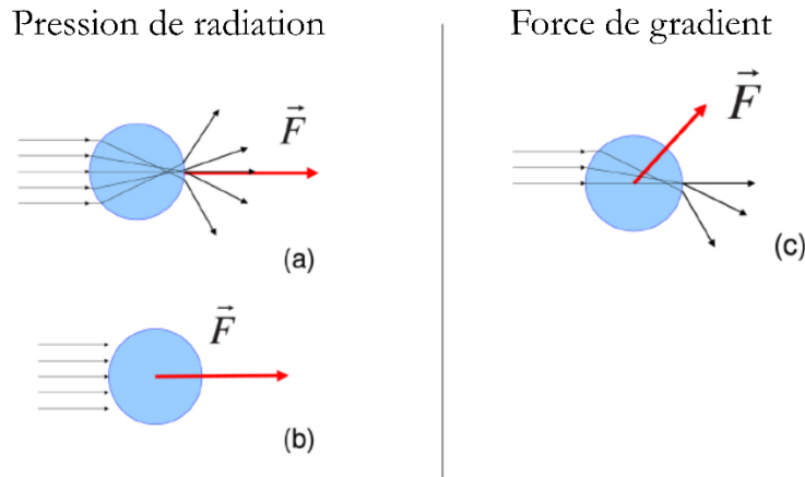
Fig. I.6 – Illustration des forces optiques de pression de radiation (a-b) et de gradient (c) dans le cas d’une sphère transparente (extrait de [ref 13]). Dans le cas d’un éclairage uniforme, la lumière peut être soit réfractée (a) soit absorbée (b), ce qui entraîne une variation de quantité de mouvement (et donc un déplacement) selon la direction de propagation de la lumière. Dans le cas d’un éclairage non uniforme la lumière est réfractée (c) ce qui entraîne un déplacement vers les régions de l’espace où l’intensité est la plus forte (c).
