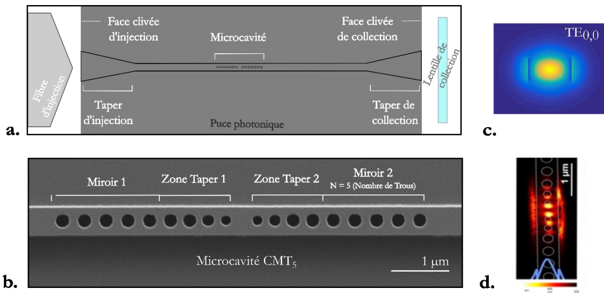
Fig. I.17 – a. Description d'une puce photonique comportant une microcavité linéique dite CMT (cristal photonique 1D). La lumière est injectée par la fibre d'injection dans le taper d'injection et est collectée par la lentille de collection après son passage dans la microcavité. Schéma de principe, les différents éléments ne sont pas à l'échelle. b. Image MEB d'une microcavité CMT_5 et du rôle des différents trous du cristal photonique. c. Mode TE_{0,0} pour lequel sont dimensionnées ces structures optiques, vue en coupe du guide d'onde. d. Image champ proche de la répartition de champ dans la microcavité.
