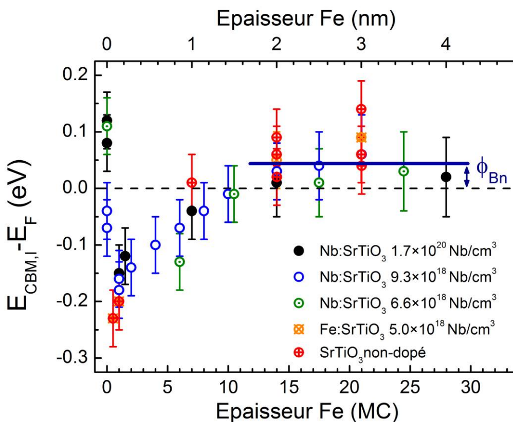
Figure IV-14 : Position relative du bas de bande de conduction E_{\text{CBM,I}} par rapport au niveau de Fermi E_{\text{F}} en fonction de l'épaisseur de fer déposée. E_{\text{CBM,I}} a été déduite de la position du Sr3d 5/2 mesurée à chaque épaisseur de fer. Des substrats de SrTiO 3 dopés n (Nb), p (Fe) et non-dopés ont été utilisés.
