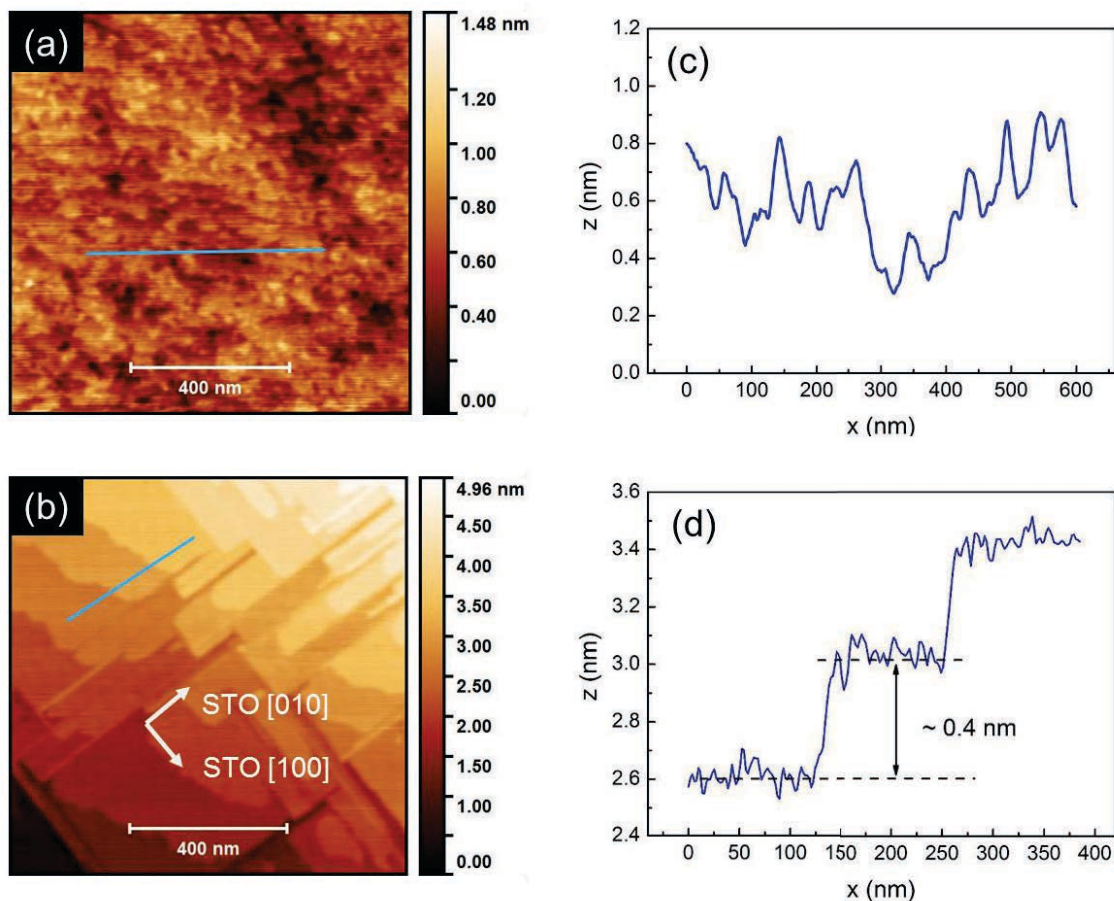
Figure II-1 : Images AFM 1 \times 1 \mu\text{m}^2 d'une surface de SrTiO 3 dopé n à 6,6 \cdot 10^{18} \text{ Nb/cm}^3 (a) Après traitement à l'acétone et propanol (b) Après recuit à 950^\circ\text{C} . Les profils correspondant à la ligne bleue tracée sur les deux images sont affichés à droite, respectivement en (c) et (d).
