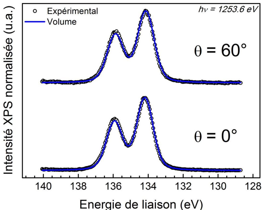
Figure II-7 : Spectres de photoélectrons normalisés après soustraction du fond pris avec la raie d'excitation MgK\alpha ( h\nu = 1253,6 eV) en émission normale et rasante du niveau de cœur Sr3d sur un substrat de SrTiO 3 dont la surface a subi une attaque à l'acide BHF. Le spectre du haut a été pris en émission rasante ( \theta = 60^\circ ) et celui du bas en émission normale ( \theta = 0^\circ ). Une seule composante a été utilisée pour réaliser l'ajustement de ces deux spectres (paramètres dans le Tableau B-2 en annexe B).
