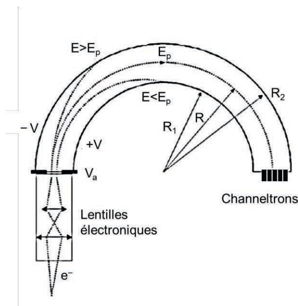
Figure I-11 : Représentation schématique de l'analyseur hémisphérique OMICRON EA 125 utilisé dans ce travail. D'après [26].
