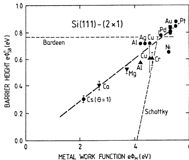
Figure IV-3: Figure extraite de [45] montrant des mesures expérimentales de hauteur de barrière Schottky de jonctions métaux/Si(111)-(2 x 1) pour les électrons e\phi_{SB}^n en fonction du travail de sortie des différents métaux e\phi_M . Les modèles de Schottky-Mott et Bardeen sont représentés en pointillés.
