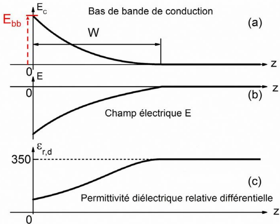
Figure V-1 : Représentation schématique pour une interface métal/SrTiO 3 pour un échantillon dopé n en régime d'appauvrissement (a) du profil du bas de bande de conduction E_c(z) par rapport à sa valeur en volume ; E_{bb} correspond à la courbure de bande en surface (b) du profil du champ électrique E(z) (c) du profil de la permittivité diélectrique relative différentielle \epsilon_{r,d}(z) .
