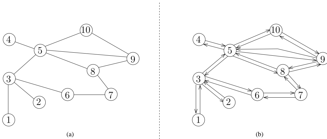
FIGURE A.2 – Exemples de graphe : (a) graphe non orienté, (b) graphe orienté.
