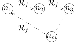
FIGURE 4.10 – Induction impossible d'un cas d'interblocage : boucle sur \mathcal{R}_f .
