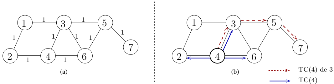
FIGURE 1.13 – Exemple d’un petit réseau de 7 nœuds pour OLSR : (a) graphe initial, (b) diffusion du message TC généré par le nœud 4.
