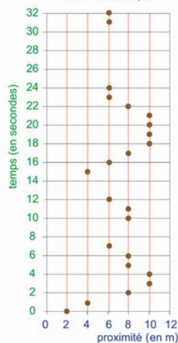
Figure 124: Principe de discrétisation spatio-temporelle des données.
