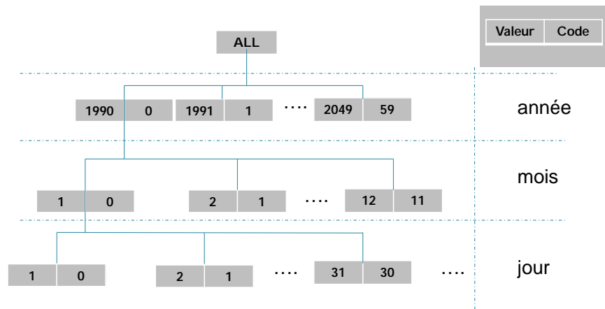
Figure 6 Exemple de dimension codée par des clés dans l'approche de [Yan et al 2015]
