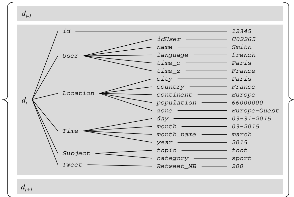
Figure 18 Exemple de document par traduction imbriquée
