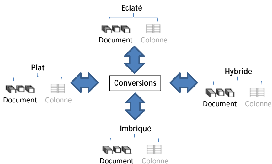
Figure 29 Processus de conversions logiques orientées documents
