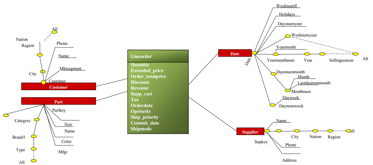
Figure 36 Le modèle conceptuel en étoile du SSB
