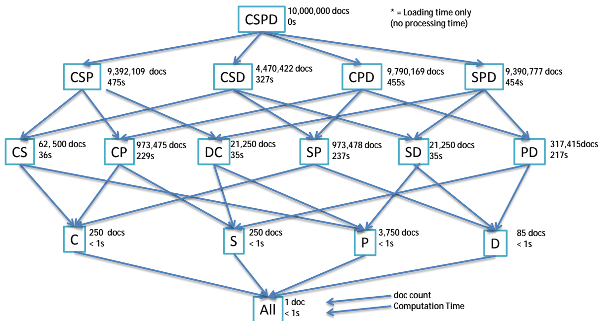
Figure 46 Treillis d'agrégats avec le temps de calcul (en secondes) et la taille (en enregistrement/ documents). Le nom des dimensions est abrégé ( D : Date , P : Part , S : Supplier , C : Customer )
