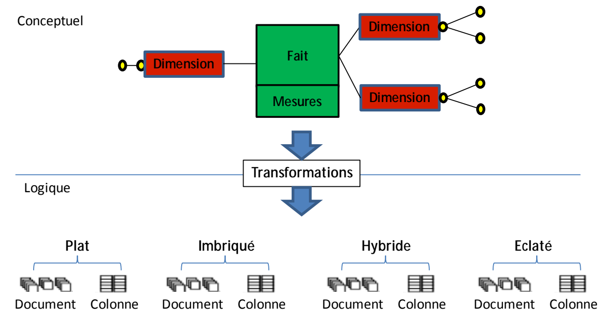
Figure 28 Processus de transformations conceptuelle - logique
