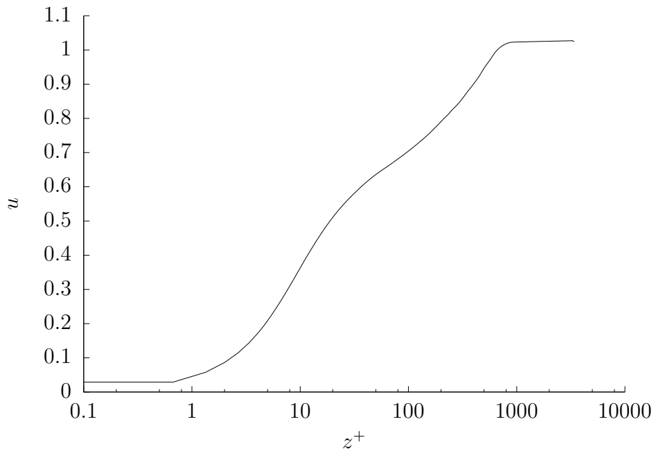
FIGURE 2.3 – Profile de vitesse moyenne dans la couche limite d'un écoulement au dessus d'une plaque laissant apparaître les différentes sections.
