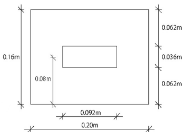
Figure 2.7 : géométrie étudiée expérimentalement par Tominaga et Blocken (Tominaga and Blocken, 2016)
