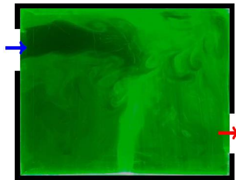
Figure 3.5 : Régime d'écoulement interne pour le cas d'un vent opposé à la flottabilité
