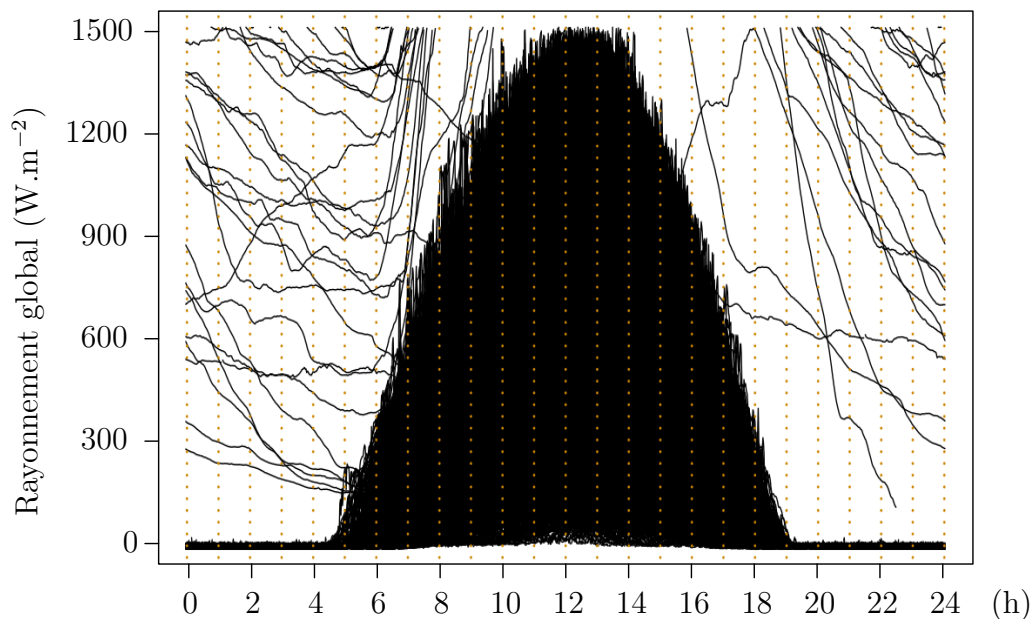
FIGURE II.4. – Représentation de l'ensemble des profils journaliers des données du laboratoire pour l'année 2014. Visualisation complémentaire des séries temporelles des deux capteurs avec les valeurs aberrantes de nuit en figure annexe A.1.
