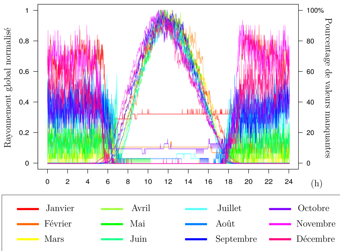
FIGURE II.3. – Profils moyens du rayonnement solaire et répartitions horaires des valeurs manquantes du site n°1 du laboratoire pour chaque mois de l'année ; Les profils mensuels sont normalisés selon leur valeur maximale ; Le ratio de valeurs manquantes est entre 0 et 100% des valeurs disponibles dans le mois.
