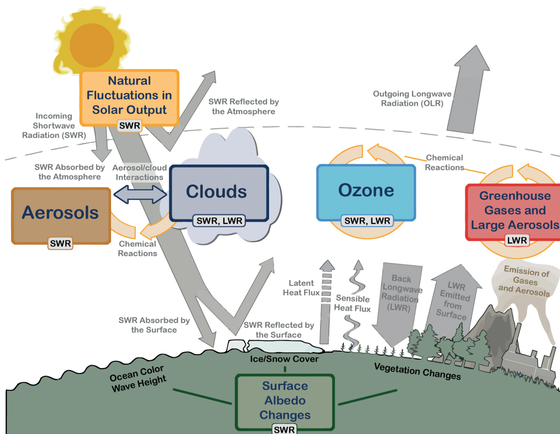
FIGURE I.3. – Schéma des acteurs atmosphériques interagissant avec le rayonnement électromagnétique, repris de IPCC (2014, Chapitre 1, Fig 1.1) , dont la légende initiale est :
