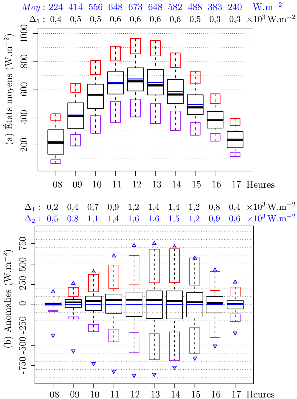
FIGURE IV.1. – Évolution diurne de la distribution des états moyens (a) et des anomalies (b); Le formalisme utilisé pour les boîtes à moustache est le même que pour toutes les figures précédentes; Pour les anomalies, des triangles bleus descendants (montants) pour localiser le minimum (maximum) de la distribution de l'heure; Au-dessus des graphes et pour chaque heure, « Moy » est la valeur de la moyenne, « \Delta_1 » est l'amplitude entre le minima du rectangle mauve et le maxima du rectangle rouge et « \Delta_2 » est l'amplitude entre le minimum et le maximum des valeurs extrêmes.
