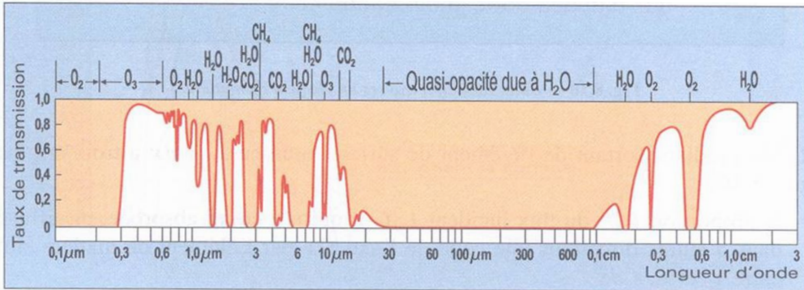
FIGURE I.4. – Spectre de l'atmosphère terrestre. Figure empruntée à Malardel (2005)
