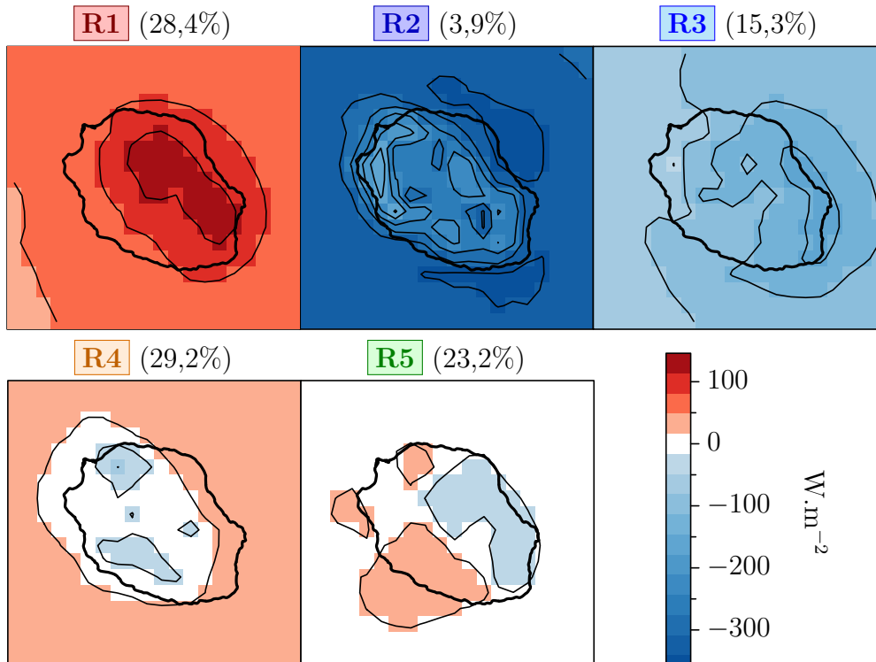
FIGURE IV.5. – Cartes des anomalies moyennes de chacun des régimes; Dans chaque sous-titre des cartes se trouve le pourcentage de jours concerné par le régime.
