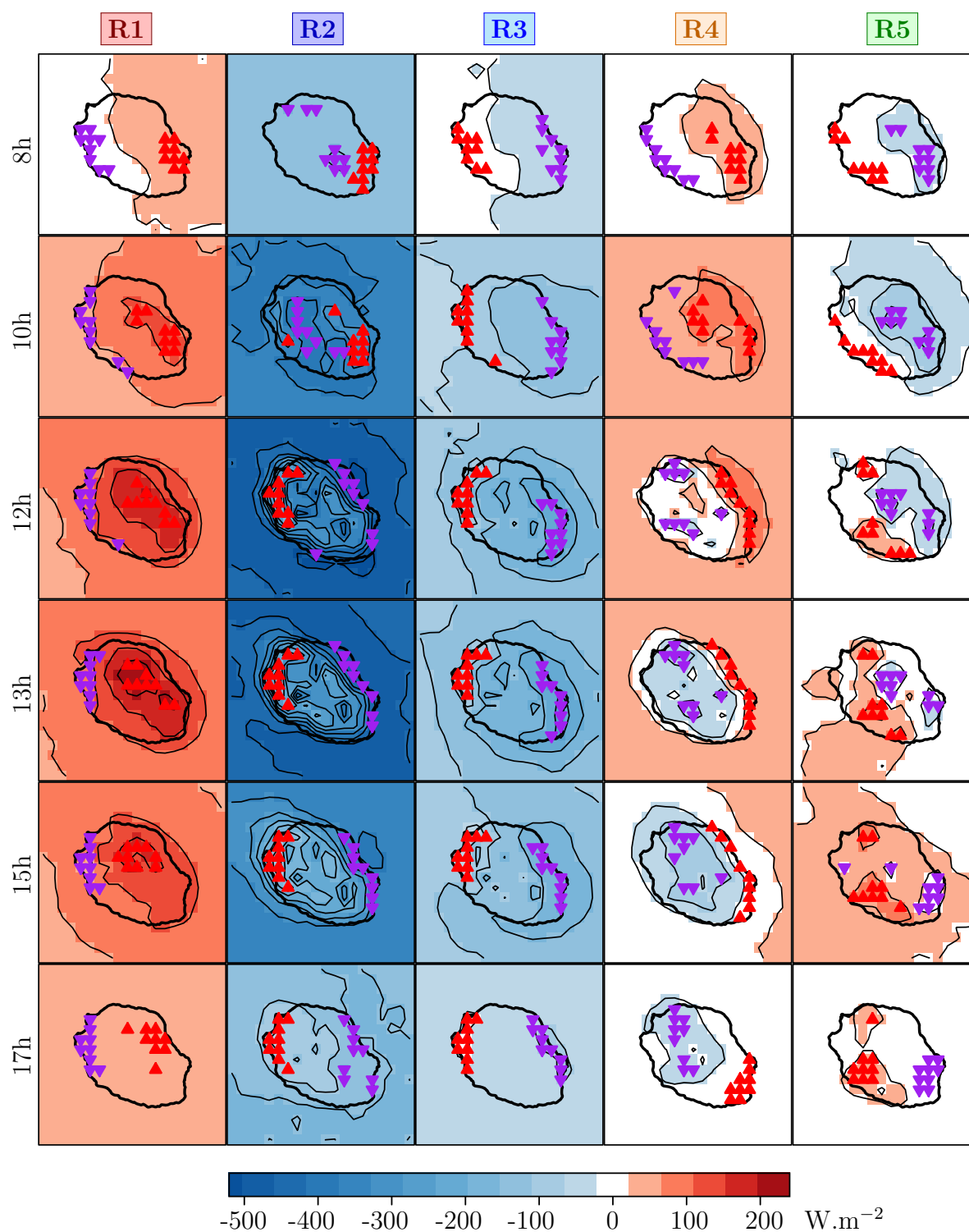
FIGURE IV.6. – Évolution diurne de chaque régime d'anomalie ; Les 10% maxima (minima) de l'île sont localisés par des triangles montants en rouge (descendants en mauve) ; La figure se voulant synthétique, nous sélectionnons 6 heures parmi les 10 disponibles qui, par ailleurs, se trouvent dans leur totalité en annexe F.
