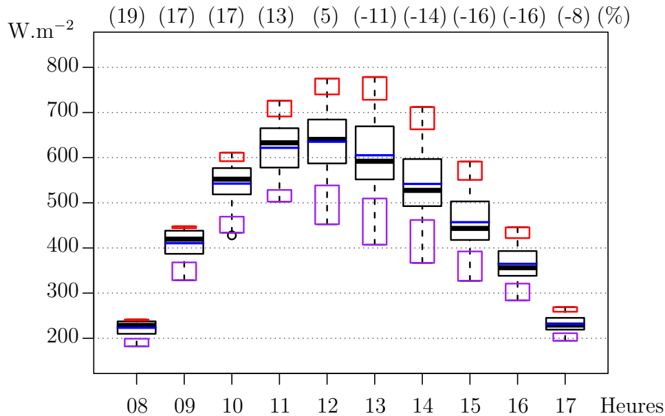
FIGURE III.4. – Évolution diurne de la distribution des pixels sur La Réunion selon des boîtes à moustaches; Les boîtes à moustaches représentent la distribution des moyennes sur chacun des 89 pixels sur l'île de La Réunion. Leurs couleurs associées sont les mêmes qu'en figure III.1; Au-dessus du graphe, les valeurs entre parenthèses sont les pourcentages d'écart entre moyenne et médiane, normalisés par les écarts interquartiles respectifs.
