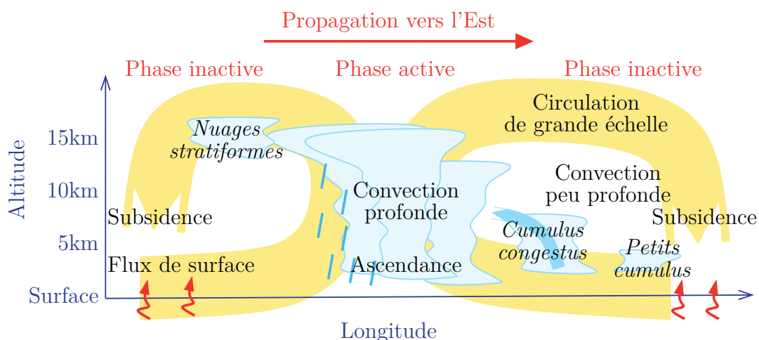
FIGURE I.11. – Schéma synthétique de la structure de la MJO en fonction de l'altitude et de la longitude, en un instant donné, figure provenant de Risi and Duvel (2014). Comme la MJO se propage vers l'est, ce schéma peut aussi représenter la structure de la MJO en fonction de l'altitude et du temps, à une longitude donnée. Les nuages dessinés représentent les types de nuages dominants. En réalité, les différentes types de nuages cohabitent dans des proportions diverses.
