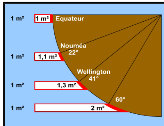
FIGURE I.2. – Étalement du rayonnement solaire incident associé à une surface d'un mètre carré selon la latitude. Figure empruntée à Maitrepierre and Divoul (2001).
