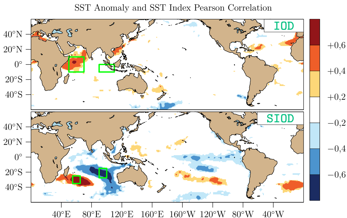
FIGURE I.14. – Représentation des dipôles de l’Océan Indien (IOD et SIOD) selon les boîtes utilisées pour l’estimation de leur indice et avec la corrélation de ces indices aux anomalies de températures de surface de la mer (de l’anglais « Sea Surface Temperature (SST) »). Figure adaptée de Hoell et al. (2017, Fig.1) dont la légende est : « Correlation of December-March 1979-2014 SST anomaly and the IOD index anomaly and the SIOD index anomaly. Shading indicates correlations significant at p < 0.10 . The IOD index is defined as areal average SST over 10^{\circ}\text{S}-0^{\circ}\text{N} ; 90^{\circ}\text{E}-110^{\circ}\text{E} subtracted from areal average SST over 10^{\circ}\text{S}-10^{\circ}\text{N} ; 50^{\circ}\text{E}-70^{\circ}\text{E} , both of which are shown as green outlines. The SIOD index is defined as areal average SST over 28^{\circ}\text{S}-18^{\circ}\text{N} ; 90^{\circ}\text{E}-100^{\circ}\text{E} subtracted from areal average SST over 37^{\circ}\text{S}-27^{\circ}\text{S} ; 55^{\circ}\text{E}-65^{\circ}\text{E} , both of which are shown as green outlines »
