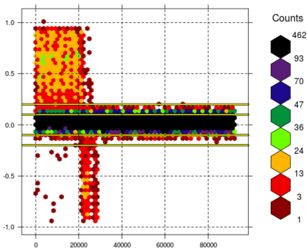
FIGURE C.2. – Corrélation (en ordonnée) de chaque grille disponible (numérotation en abscisses) avec une grille aberrante. Les lignes jaunes localisent les corrélations à \pm 0,1 et à \pm 0,2 . Les hexagones et leurs couleurs renseignent sur la densité des grilles présentes.
