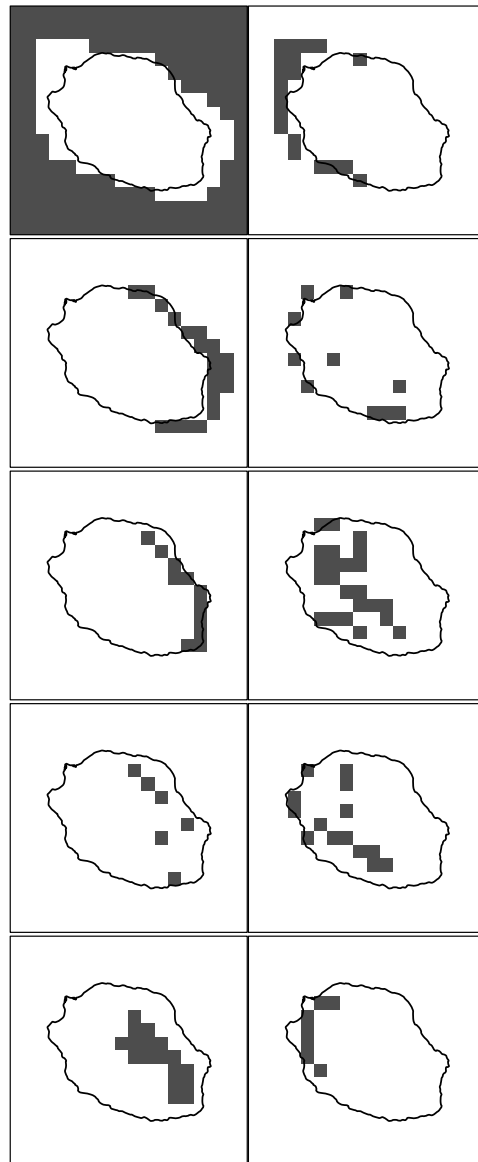
FIGURE E.6. – Visualisation séparée des 10 classes. Pour rappel, c'est le cas de classification choisi. Nous disposons les graphes selon la même répartition que pour la figure III.16.
