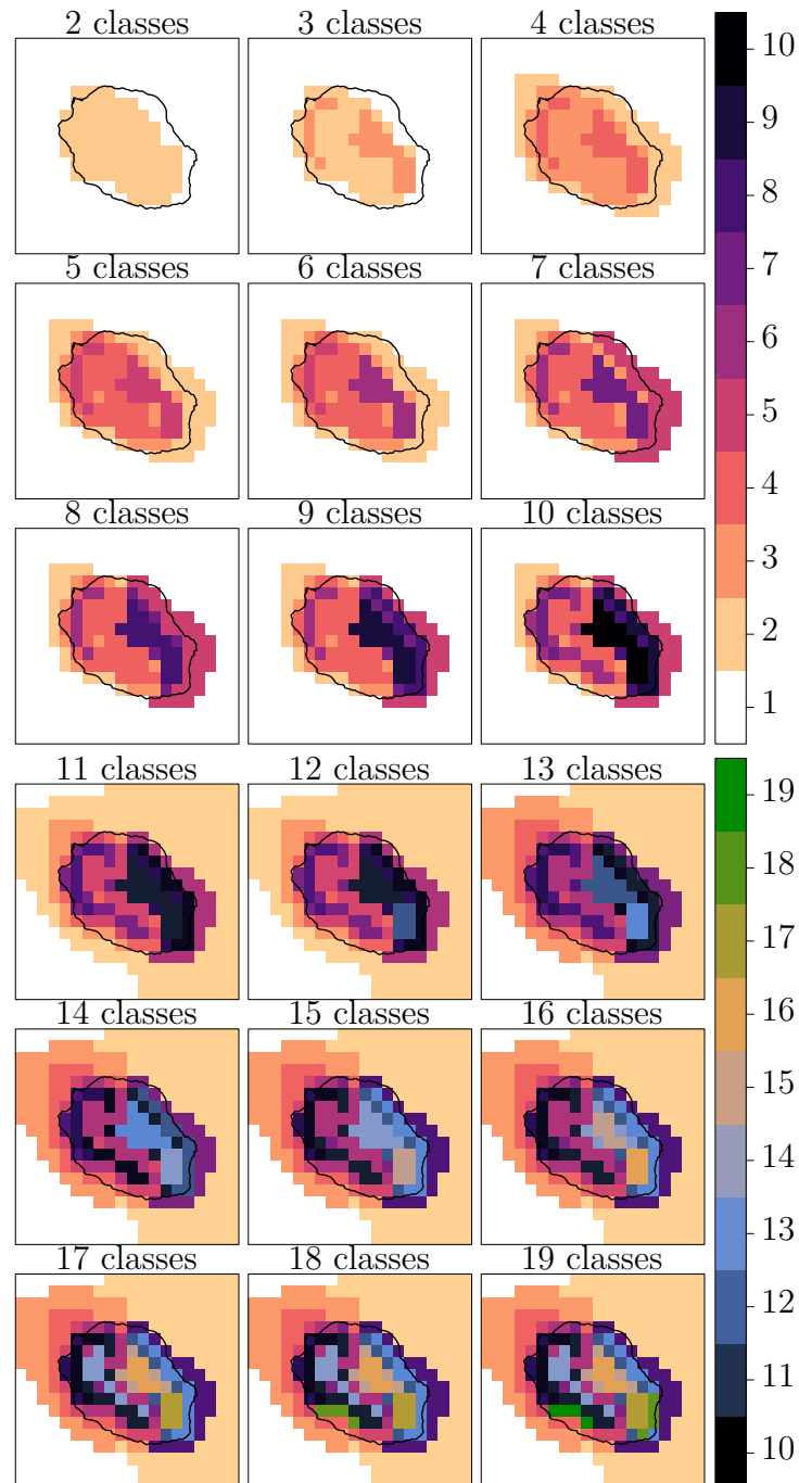
FIGURE E.5. – Cas de classification de 2 à 19 classes
