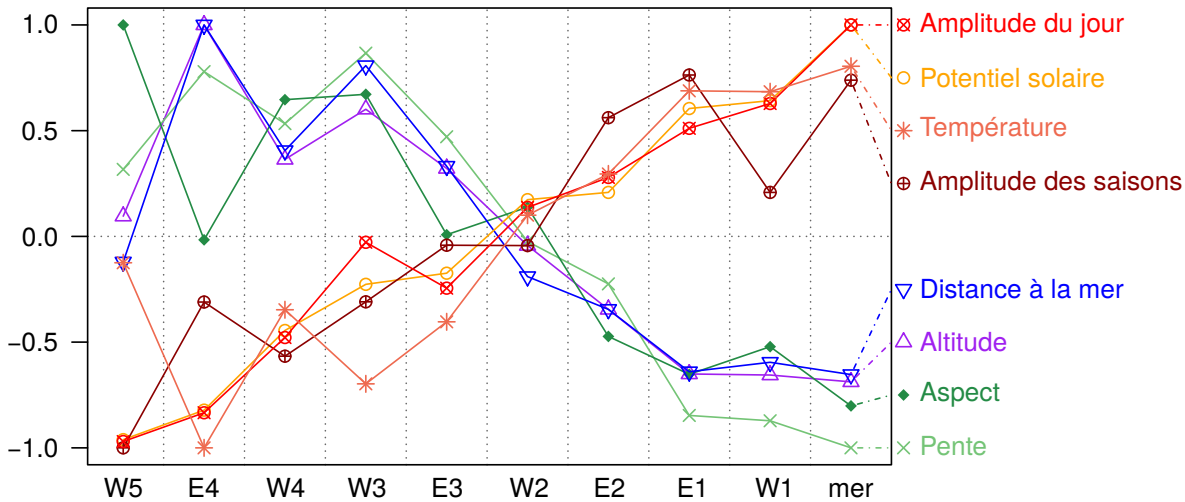
FIGURE IV.1. – Distribution relative des moyennes de chaque classe au regard des paramètres topographiques et solaires selon les différentes classes; Les classes sont rangées par potentiel solaire moyen croissant. Les paramètres solaires sont calculés à partir des données SARAH-E : le potentiel solaire est le rayonnement solaire global moyen, l'amplitude du jour est le maximum du rayonnement solaire du jour, l'amplitude des saisons est l'écart entre les extrema des amplitudes du jour de chacun des mois de l'année, la température provient des données de l'atlas climatique de Météo-France, soit une climatologie mensuelle reconstruite à 250 mètres de résolution par interpolation spatiale (Jumaux et al., 2011), Les paramètres topographiques sont calculés à partir d'un modèle numérique de terrain (MNT) à 30 mètres (NASA JPL, 2009) : l'altitude est la moyenne sur la zone équivalente que couvrent les pixels de la classe (à \sim 5 km), la distance à la mer est calculée entre le contour de La Réunion et chacun des pixels du MNT selon une distance calculée avec les coordonnées UTM et l'altitude, l'aspect et la pente sont calculés en utilisant la fonction terrain du package raster sous R.
