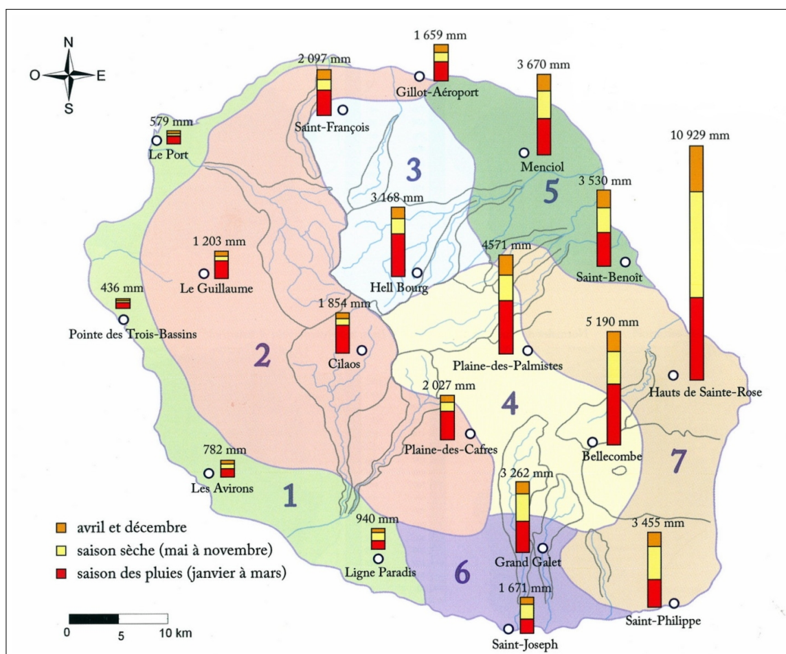
FIGURE I.21. – Répartition saisonnière des précipitations annuelles (normales 1981-2010) Figure reprise de Jumaux et al. (2011) . Les zones pluviométrique de l'île sont colorées et numérotées de 1 à 7. Les stations d'observations sont localisés par des cercles noirs.
