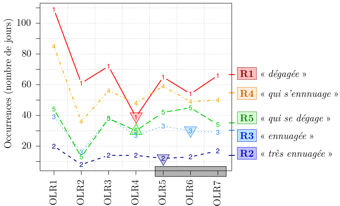
FIGURE F.5. – Occurrences des régimes de perturbations solaires selon les régimes d'Outgoing Longwave Radiation (OLR) par Fauchereau et al. (2009), version graphique de la table IV.4. Le rectangle gris rappelle les phases pendant lesquelles le maximum de convection est dans l'Océan Indien. Les cercles localisent les occurrences significatives, selon un test de significativité à 95 %, par des triangles montants (descendants) selon si la valeur est significativement supérieure (inférieure).
