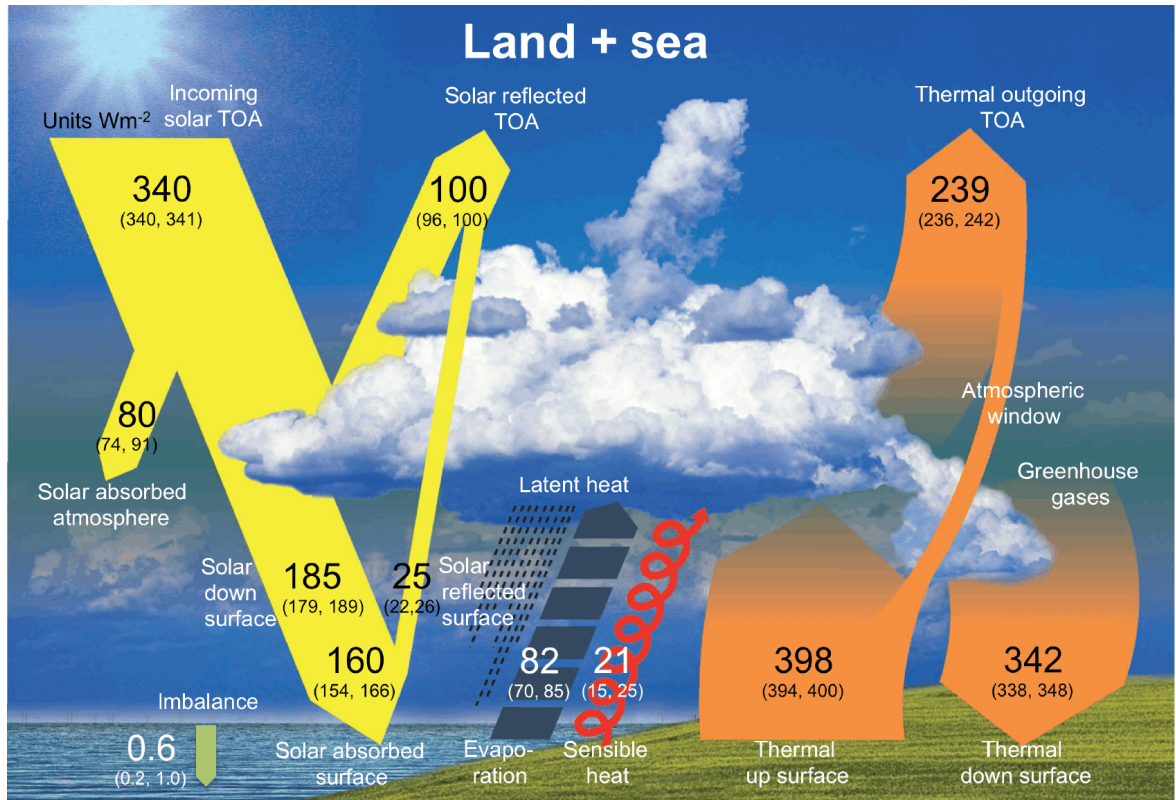
FIGURE I.6. – Schéma du bilan radiatif de la Terre, figure provenant de Wild et al. (2015a, 2017). Les nombres indiquent les meilleures estimations des amplitudes de chaque composante du bilan énergétique moyen mondial (en \text{W.m}^{-2} ) ainsi que leurs plages d'incertitude entre parenthèses, représentant les conditions climatiques actuelles au début du 21 ème siècle. Les flux au-dessus de l'atmosphère sont déterminés à partir des observations satellitaires du CERES. Les estimations du flux radiatif de surface sont dérivées de la structure de biais du modèle CMIP5 en ce qui concerne les observations des réseaux GEBA et BSRN, comme indiqué dans Wild et al. (2013, 2015a).
