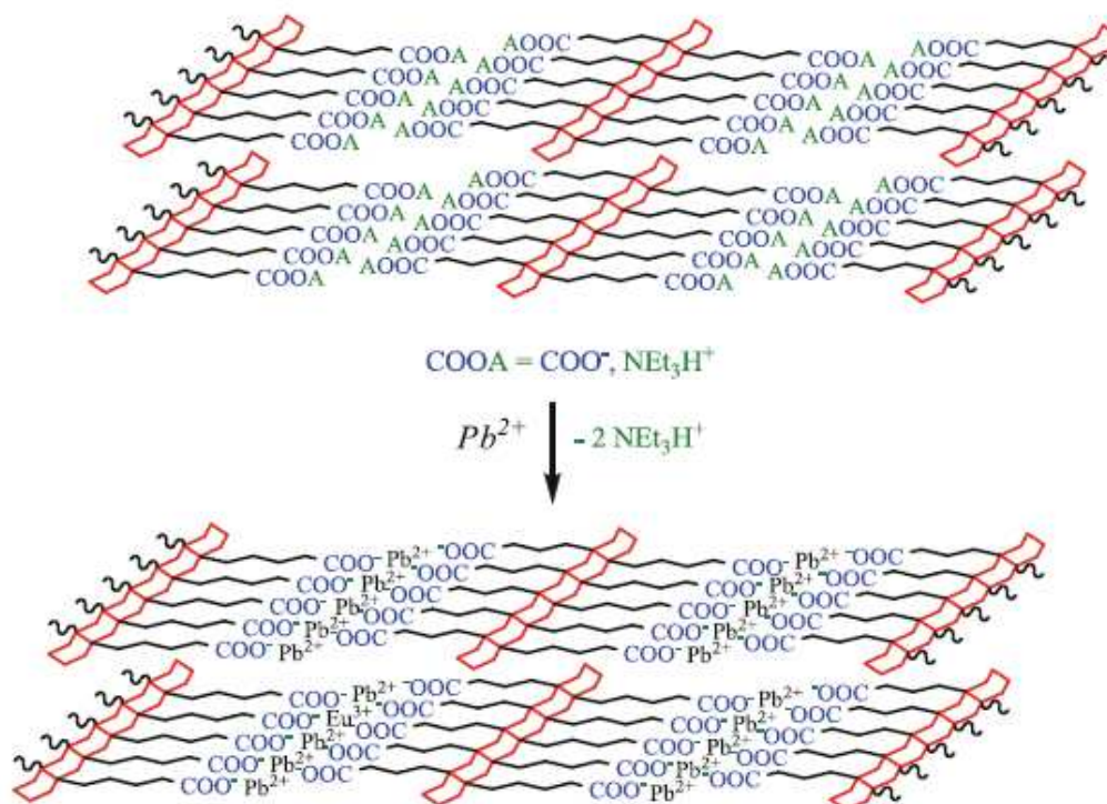
Figure 49 : Extraction du plomb par les matériaux mésoporeux.
