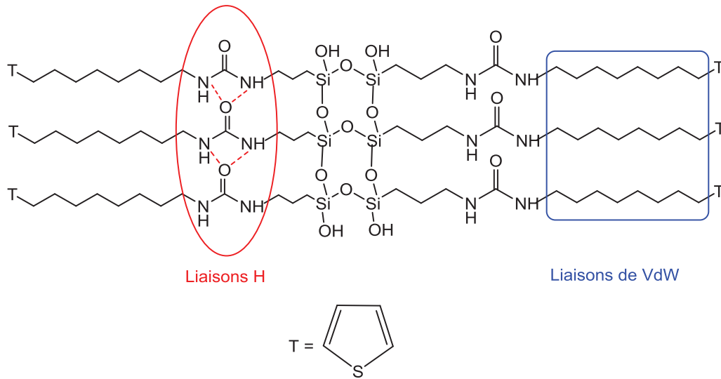
Figure 17 : Représentation schématique du matériau hybride SiO 2 /thiophène.
