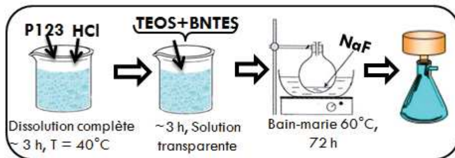
Schéma 15 : résumé sur le mode de synthèse du Si-SBA-15-CN
