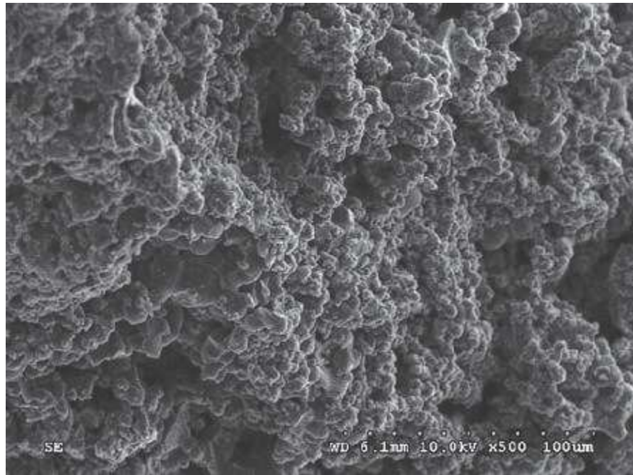
Figure 42 : Image par microscopie électronique à balayage du matériau O_{1.5}Si(CH_2)_3-COOH
