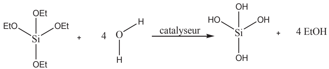
Equation 1: Hydrolyse du TEOS
