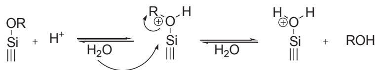
Figure 1: Hydrolyse par catalyse acide
