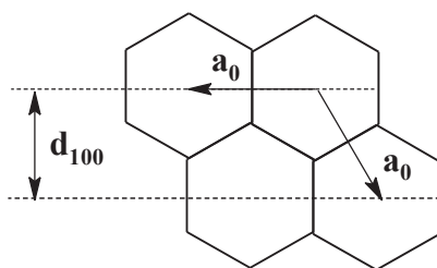
Figure 64 : Relation entre a_0 et d_{100} dans les matériaux mésoporeux de structure hexagonale.
