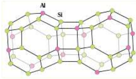
Figure 35 : répartition des atomes Al et Si dans une zéolithe de type Y (2 cavités \beta reliées par une cavité \gamma )
