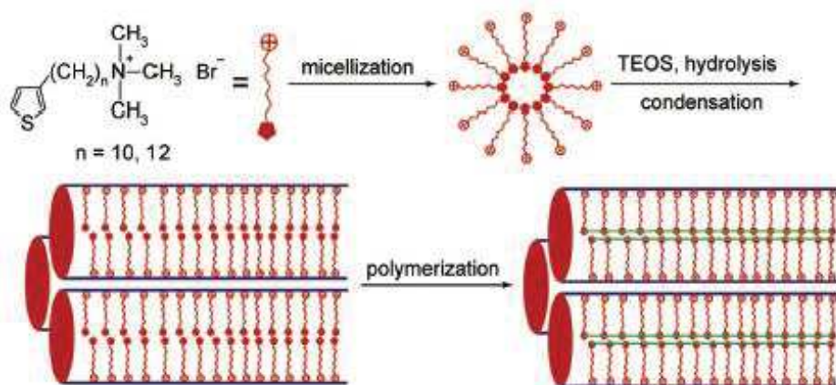
Figure 16: Formation de matériaux hybrides polythiophène/SiO 2 par polymérisation in situ [131].
