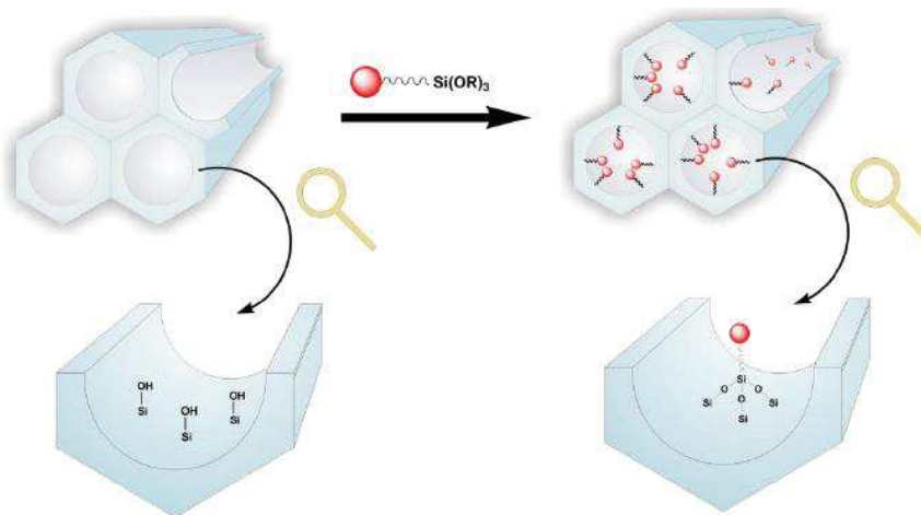
Figure 10: Fonctionnalisation par greffage
