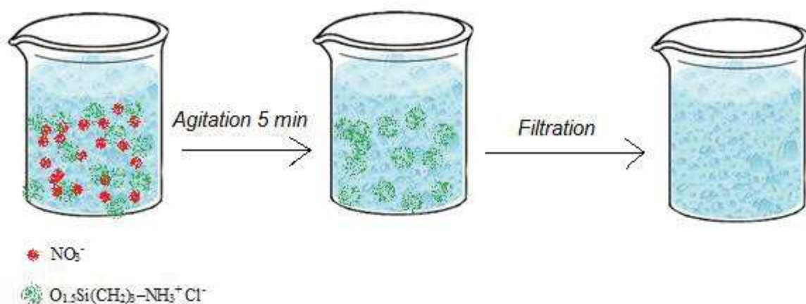
Figure 53 : Schéma de l'extraction des nitrates de l'eau
