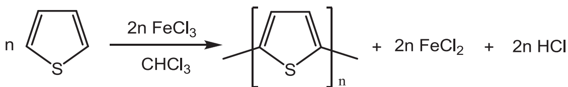
Schéma 3: Polymérisation oxydative par \text{FeCl}_3
