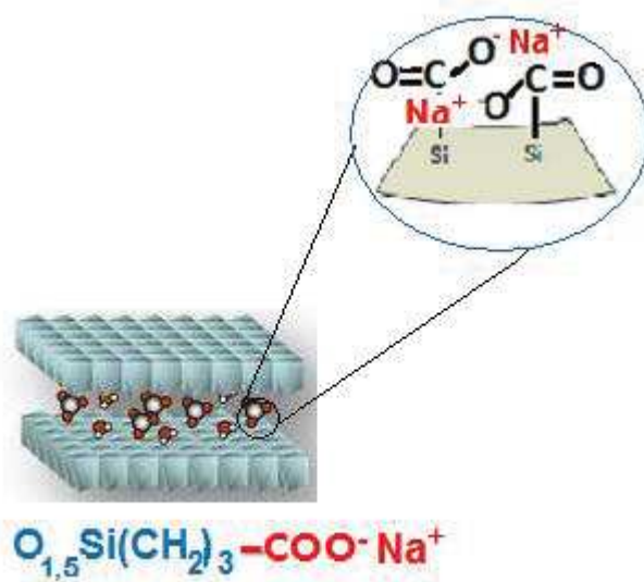
Figure 52 : Représentation schématique du matériau lamellaire fonctionnalisé par l'acrylate de sodium
