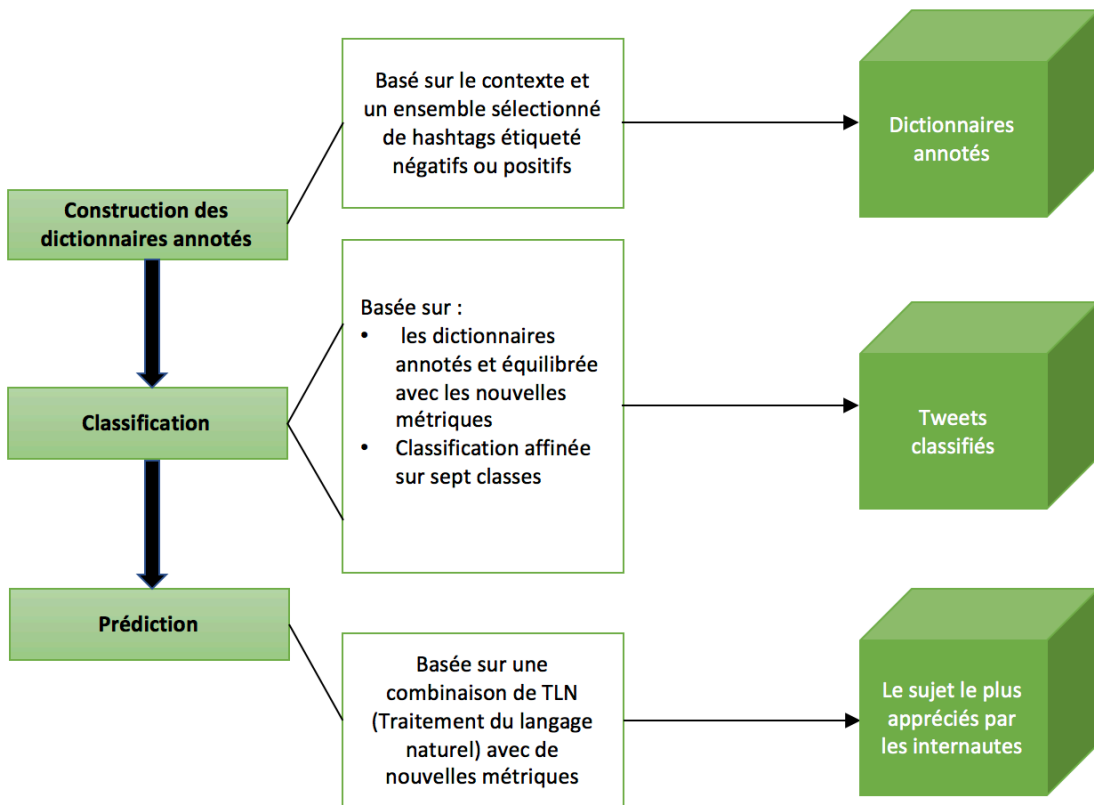
Figure 14: Les étapes de l'approche proposée
