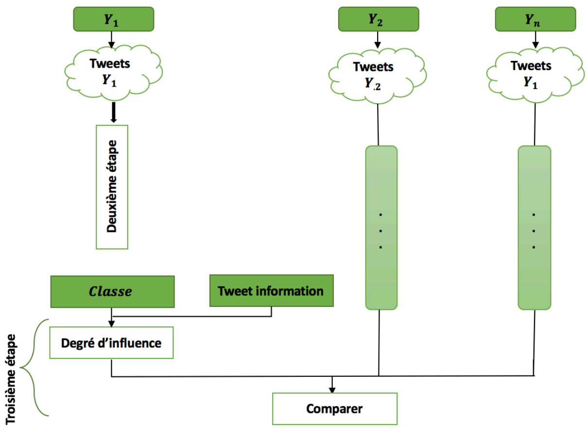
Figure 18: la troisième étape du modèle
