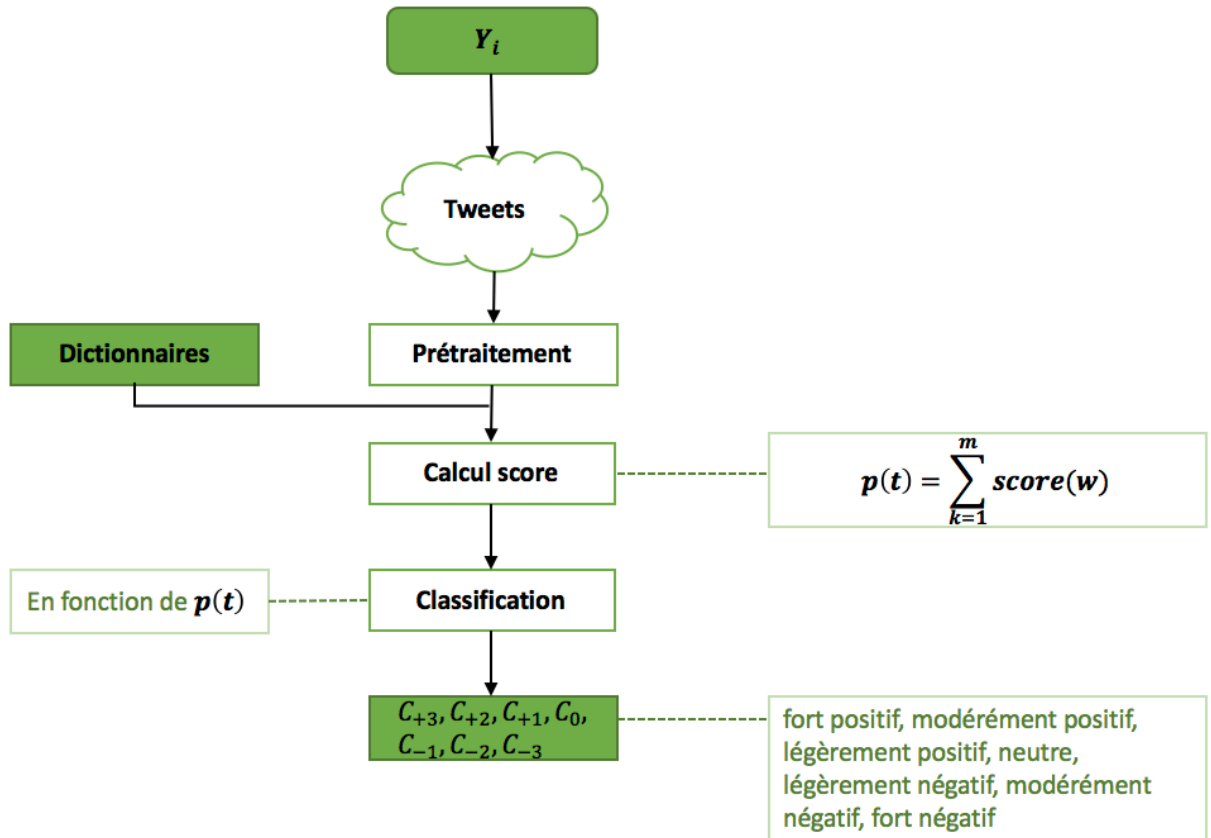
Figure 17: La deuxième étape du modèle
