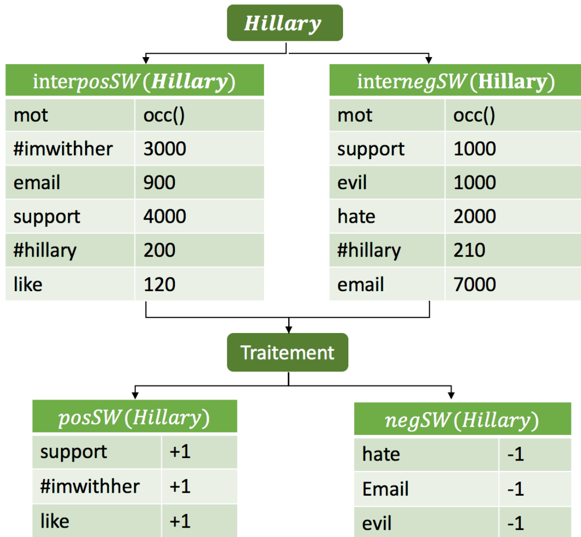
Figure 19: Exemple de construction de dictionnaire Hillary
