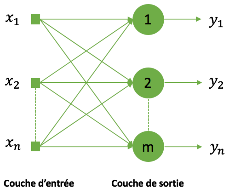
Figure 10: Exemple de Naïve Bayes monocouche
