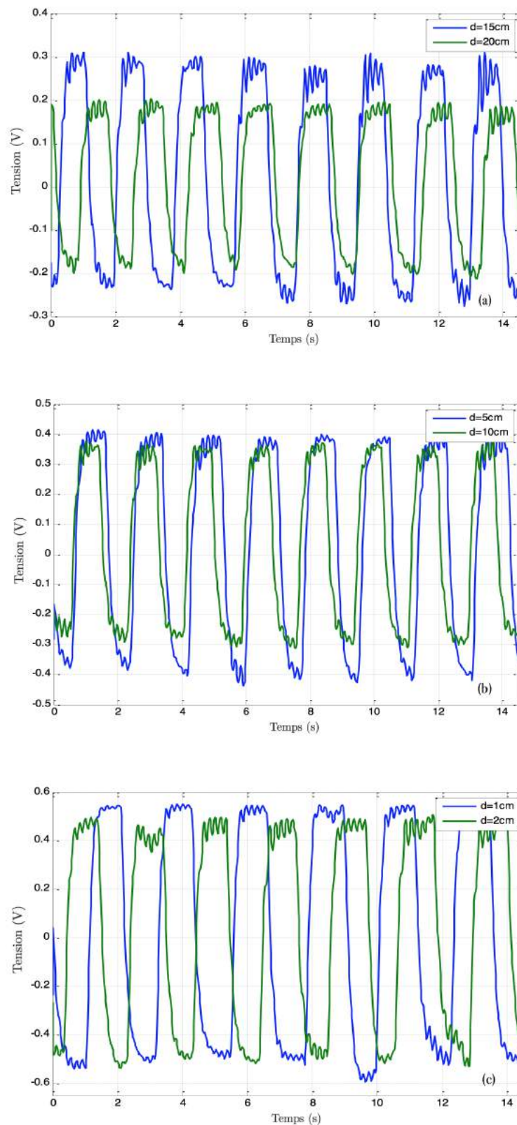
FIGURE 3.7: Évolution temporelle de la tension pyroélectrique aux bornes de la céramique pyroélectrique PZT pour différentes distances : (a) d = 15\text{cm} , 20\text{cm} , (b) d = 10\text{cm} , 5\text{cm} et (c) d = 2\text{cm} , 1\text{cm}
