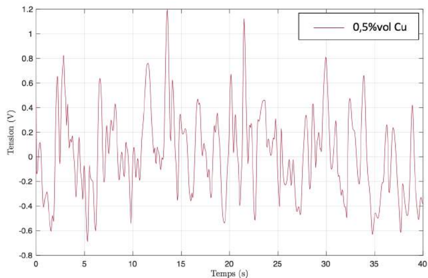
FIGURE 5.3: Evolution temporelle de la tension en sortie de la céramique en utilisant huile de colza + 0,5%vol de Cu
