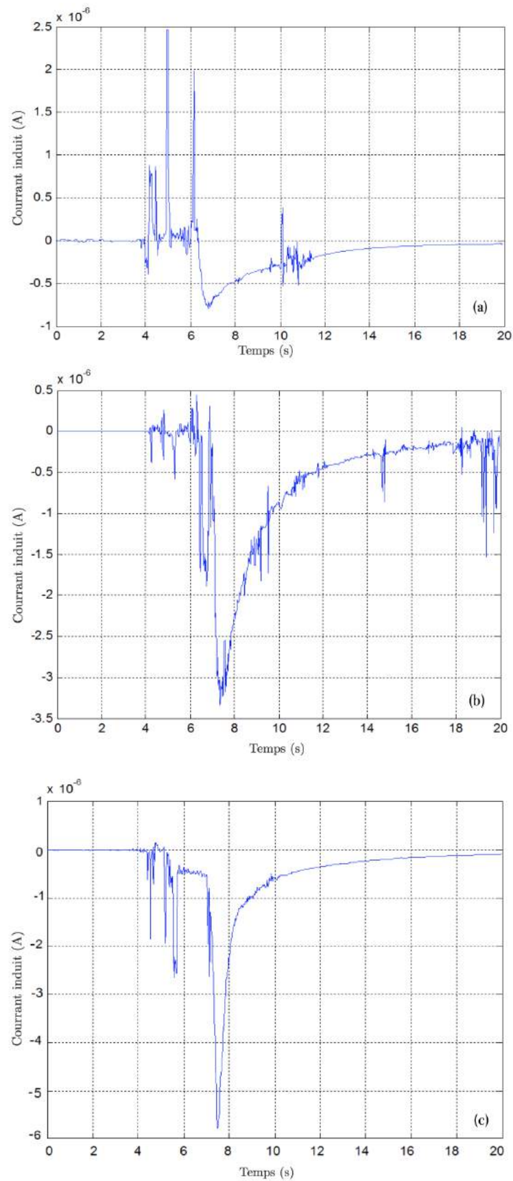
FIGURE 3.3: Courant généré par notre échantillon pour différentes températures : (a) 40^{\circ}\text{C} , (b) 60^{\circ}\text{C} et (c) 80^{\circ}\text{C}
