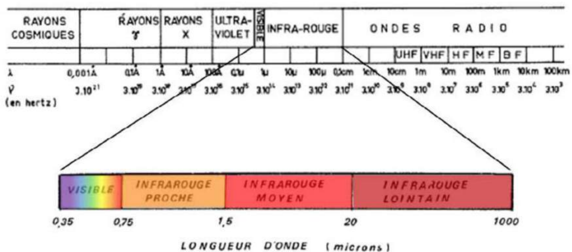
FIGURE 2.10: Ondes électromagnétiques [16].
