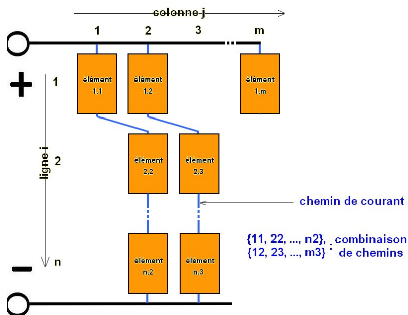
FIGURE 1.6 – Combinaisons dans une architecture
