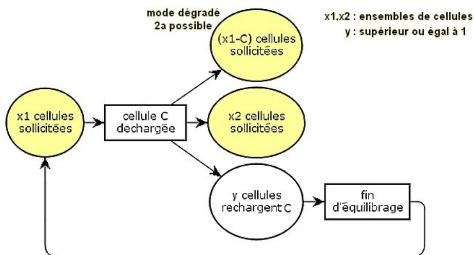
FIGURE 2.9 – Graphe de mode lorsqu'une cellule est déchargée
