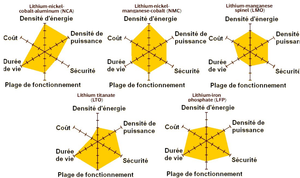
FIGURE 6.3 – Comparaison des performances spécifiques à chaque chimie usuelle [54]
