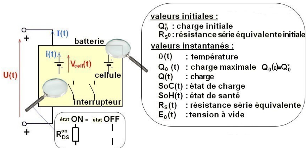
FIGURE 1.36 – Une batterie est composée de cellules et d'interrupteurs
