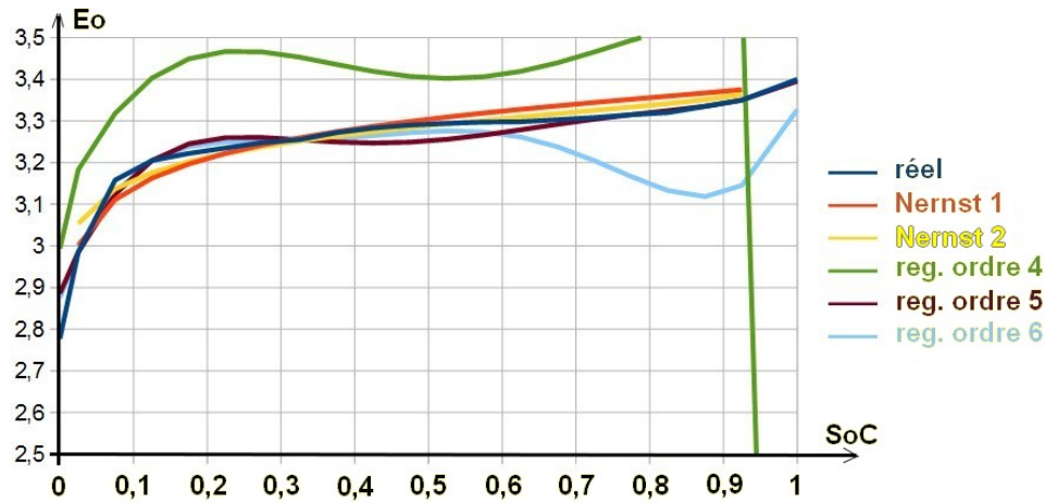
FIGURE 3.1 – Modélisation d'une courbe E_0(\text{SoC}) pour une cellule \text{LiFePO}_4
