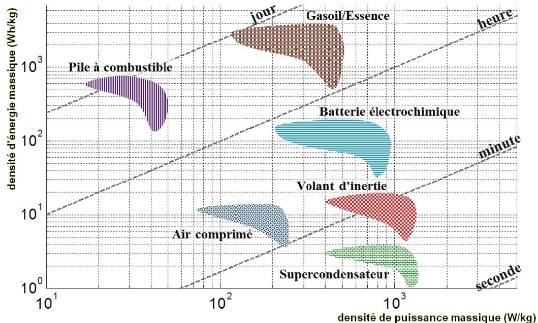
FIGURE 1.4 – Diagramme de Ragone pour différents SSEE [136]
