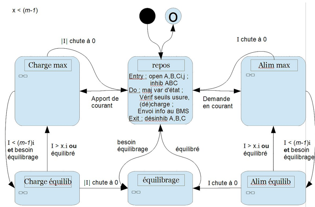
FIGURE 4.3 – Diagramme d'état SYSML d'une batterie
