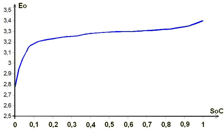
FIGURE 1.10 – Allure de la courbe fondamentale E_0 = f(\text{SoC}) pour une cellule \text{LiFePO}_4
