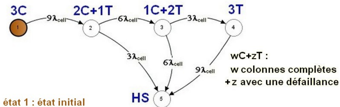
FIGURE 2.21 – Chaîne de Markov d'une architecture S3P3 « tolérante »
