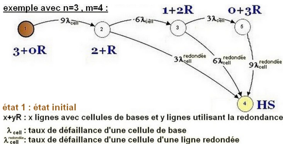
FIGURE 2.23 – Chaîne de Markov associée aux architectures C3C et PS
