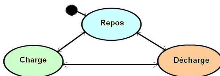
FIGURE 4.2 – Diagramme d’état d’une batterie
