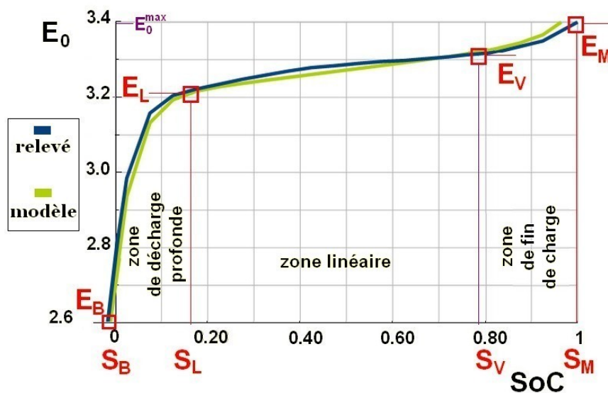
FIGURE 3.2 – Identification de trois zones distinctes sur la courbe E_0 = f(\text{SoC})
