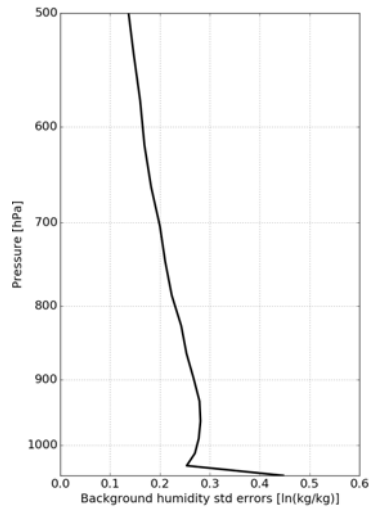
FIGURE 3.24 – Écart-types d’erreurs sur les profils d’humidité de la surface à 500 hPa, obtenus après pondération des erreurs fournies par le NWPSAF, par la contribution de chaque niveau de pression à la correction troposphérique humide.
