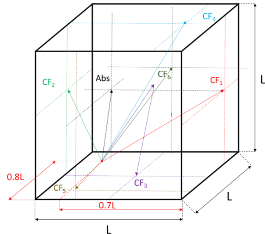
Fig. 21 – Calcul de facteurs de forme dans une cavité cubique.
