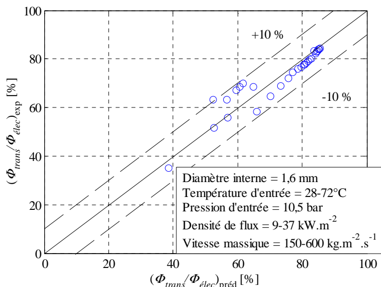
Figure 2-32 Evolution de la part de flux transmis constatée expérimentalement en fonction de la part de flux transmis prédite pour l'évaporateur
