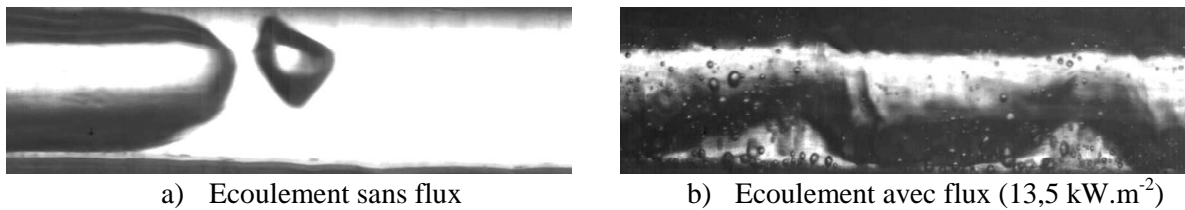
Figure 5-10 Images représentatives de l'écoulement pour G = 150 \text{ kg.m}^{-2}.\text{s}^{-1} , x = 0,2 et \beta = 30^\circ
