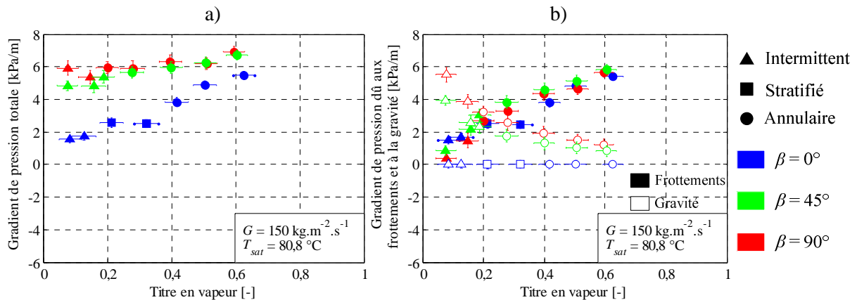
Figure 4-15 Evolution du gradient de pression totale (a) et des composantes du gradient de pression (b) en fonction du titre en vapeur pour un d_{int} = 1,6 \text{ mm} , G = 150 \text{ kg.m}^{-2}.\text{s}^{-1} , T_{sat} = 80,8 \text{ °C} et \beta = 0^\circ, 45^\circ et 90^\circ (ascendants)
