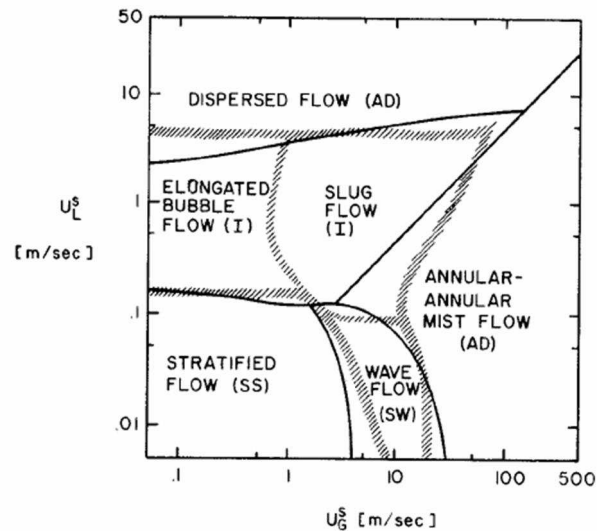
Figure 1-3 Carte d'écoulement de Taitel et Dukler (1976) comparée à la carte de Mandhane et al. (1974) (Taitel and Dukler, 1976)
