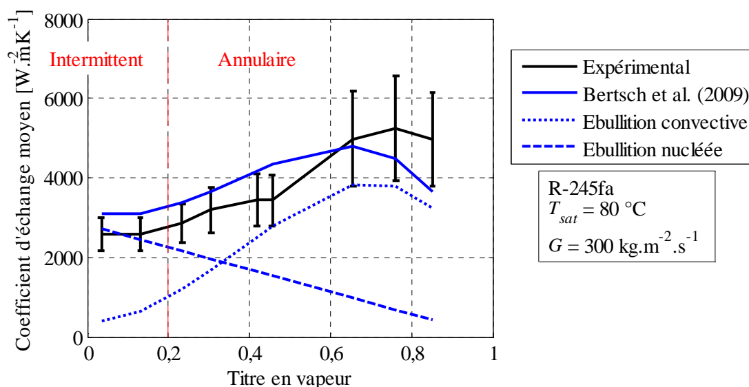
Figure 5-30 Evolution des prédictions du modèle de Bertsch et al. (2009) en fonction du titre en vapeur pour une vitesse massique de 300 \text{ kg.m}^{-2}.\text{s}^{-1} en configuration horizontale
