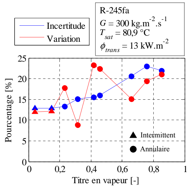
Figure 5-25 Evolution de l'incertitude et de la variation relative de \alpha sur la gamme d'inclinaison en fonction du titre en vapeur pour les tests réalisés à 300 \text{ kg.m}^{-2}.\text{s}^{-1}
