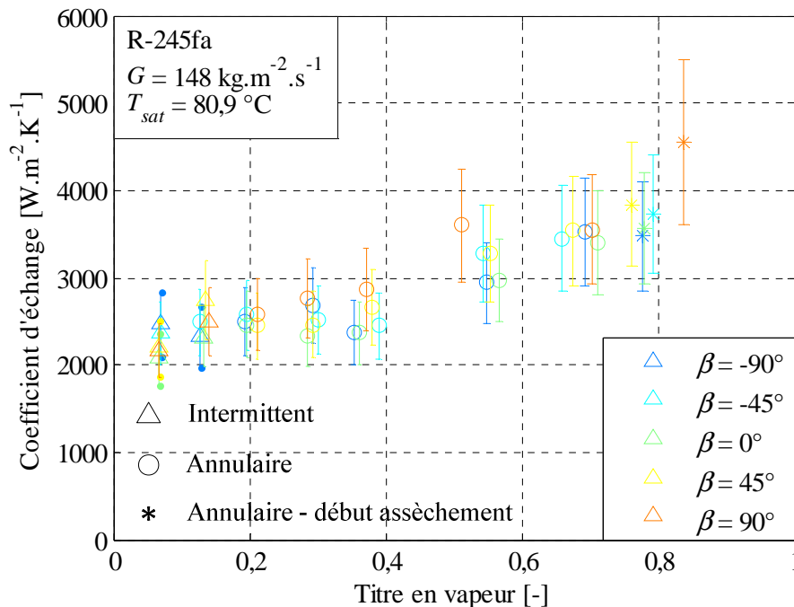
Figure 5-26 Evolution du coefficient d'échange avec le titre en vapeur pour une vitesse massique de 148 kg.m -2 .s -1 et des angles d'inclinaison de -90°, -45°, 0°, 45° et 90°
