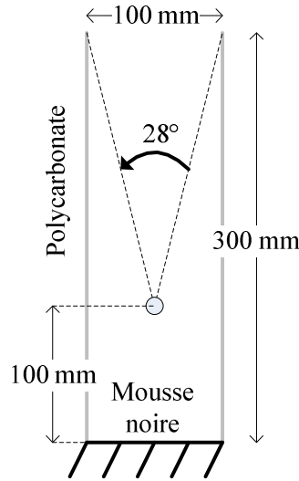
Figure C-1 Disposition de la mousse noire et des plaques en polycarbonate autour du tube en saphir
