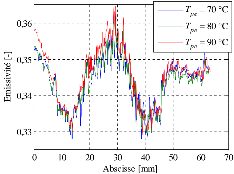
Figure 2-13 Profils d'émissivité pour une température de dépôt de T_{pe} = 70\text{ °C} , 80\text{ °C} et 90\text{ °C} et G = 2000\text{ kg.m}^{-2}.\text{s}^{-1}
