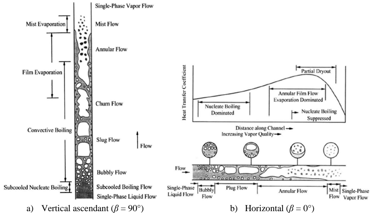
Figure 1-1 Schéma des régimes d'écoulement et des modes de transfert de chaleur en ébullition convective verticale ascendante (a) et horizontale (b) en macro-canal (Cheng et al., 2008)
