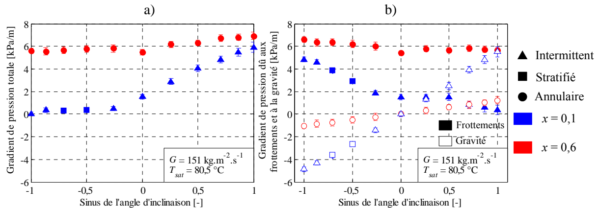
Figure 4-17 Evolution du gradient de pression totale (a) et des composantes du gradient de pression (b) en fonction du sinus de l'angle d_{int} = 1,6 \text{ mm} , G = 150 \text{ kg}\cdot\text{m}^{-2}\cdot\text{s}^{-1} , T_{sat} = 80,6^\circ\text{C} et x = 0,1 et 0,6
