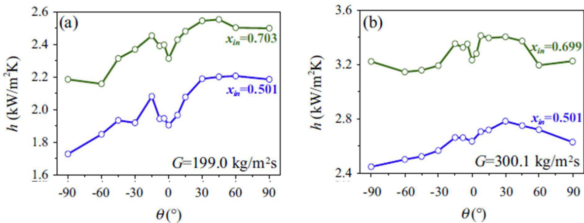
Figure 1-30 Evolution du coefficient d'échange avec l'inclinaison pour la condensation du R245fa dans une conduite de 14,81 mm de diamètre intérieur (Xing et al. (Xing et al., 2015))
