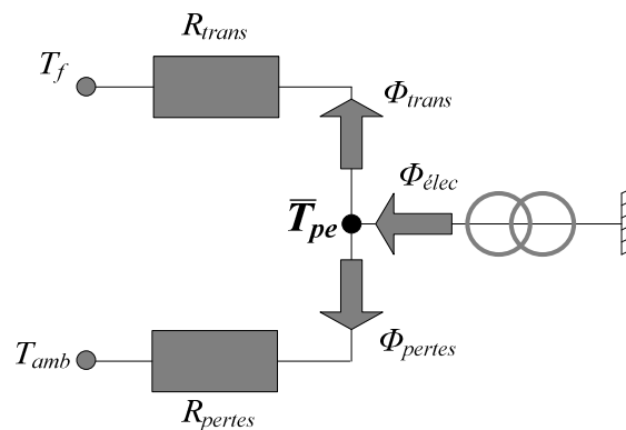
Figure 2-28 Schéma électrique équivalent du bilan global avec pertes thermiques du préchauffeur
