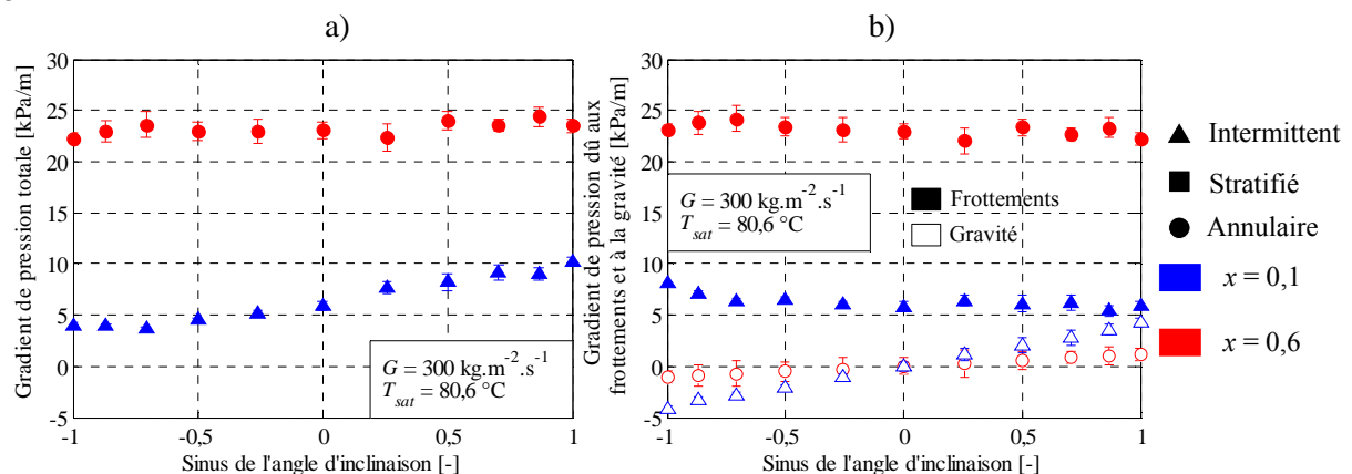
Figure 4-18 Evolution du gradient de pression totale (a) et des composantes du gradient de pression (b) en fonction du sinus de l'angle d_{int} = 1,6 \text{ mm} , G = 300 \text{ kg}\cdot\text{m}^{-2}\cdot\text{s}^{-1} , T_{sat} = 80,6^\circ\text{C} et x = 0,1 et 0,6
