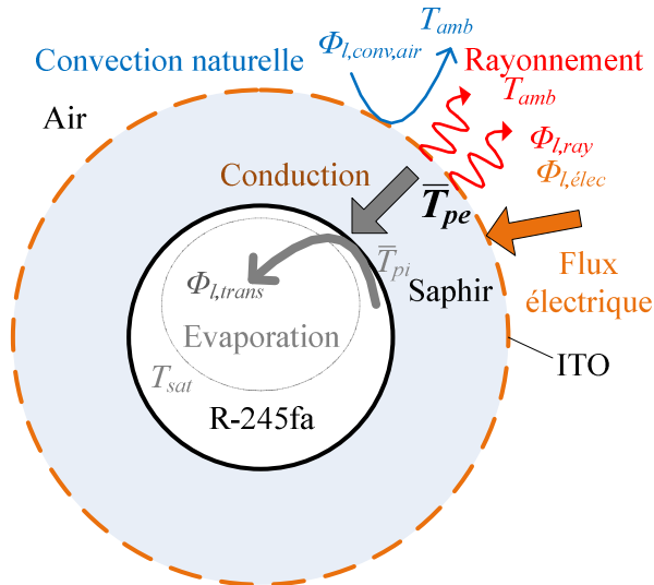
Figure 2-21 Bilan thermique sur une section
