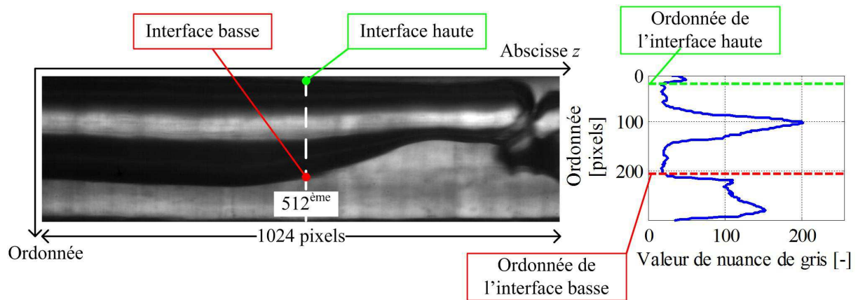
Figure 3-2 Image d'un écoulement poche-bouchon et profil de gris correspondant
