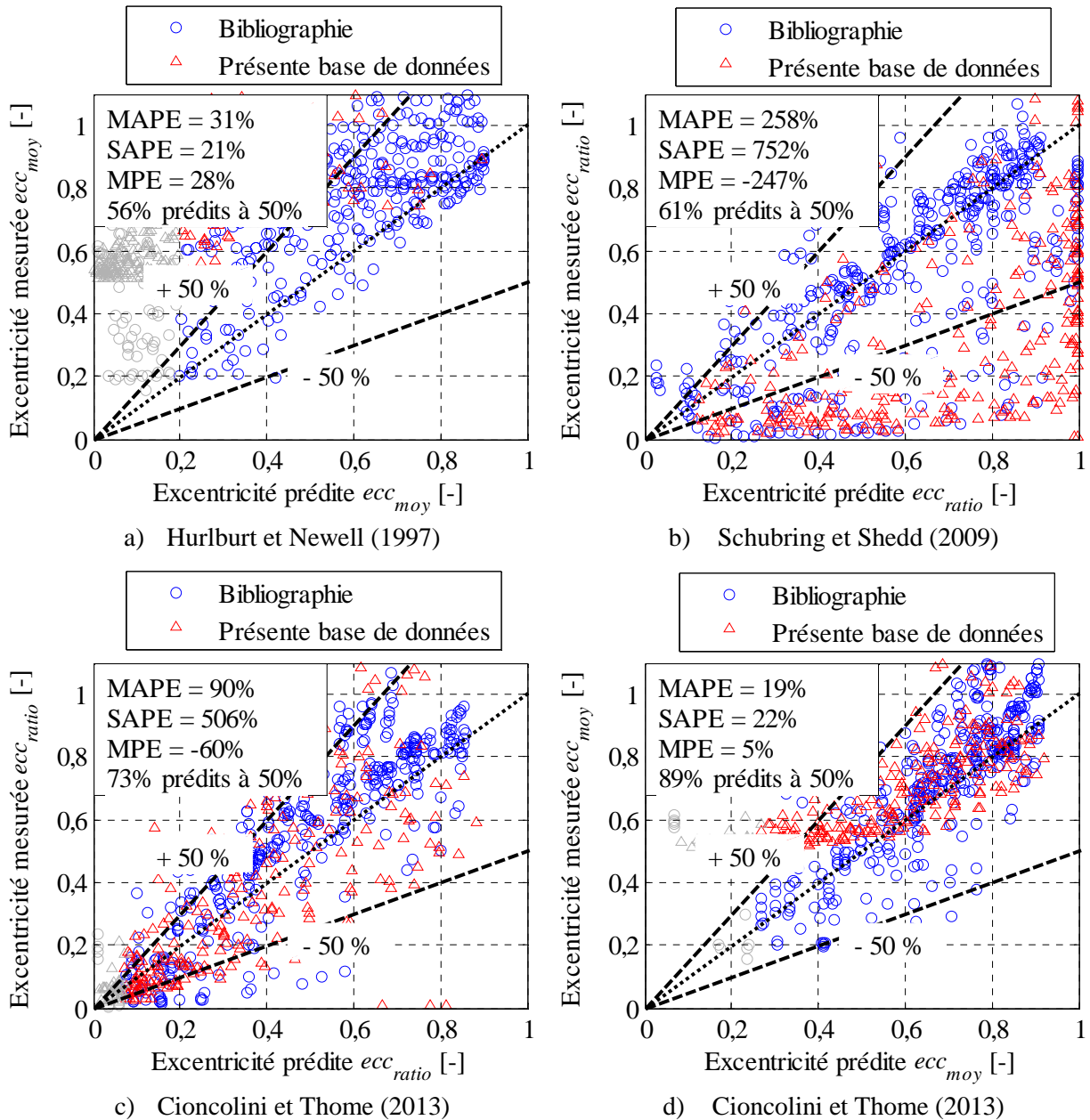
Figure 3-10 Excentricité mesurée en fonction de l'excentricité prédite pour les corrélations de a) Hurlburt et Newell (1997), b) Schubring et Shedd (2009), c) et d) Cioncolini et Thome (2013)
