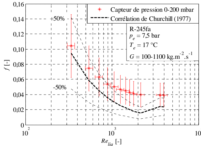
Figure 2-37 Comparaison des coefficients de frottement expérimentaux et prédits par la corrélation de Churchill (1977)
