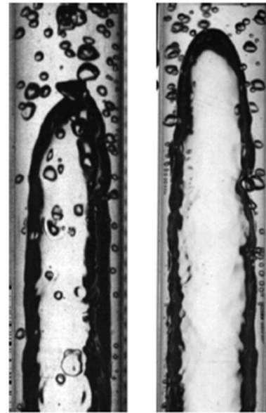
Figure 1-22 Images d'écoulements à poches-bouchons avec flux imposé non nul (Narcy et al., 2014)
