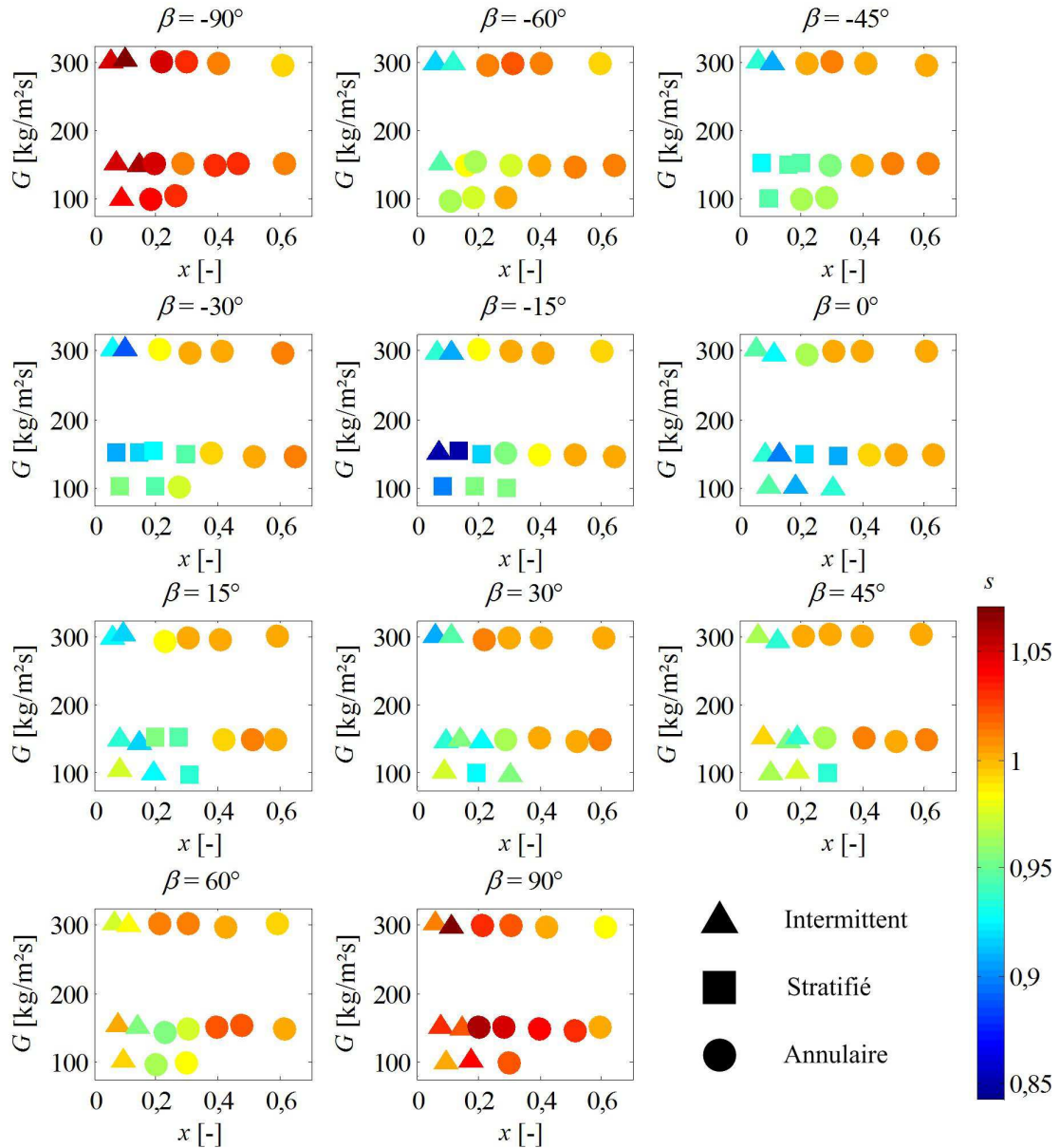
Figure 3-19 Cartes d'évolution du paramètre de symétrie en fonction de la vitesse massique et du titre en vapeur pour les écoulements ascendants et descendants inclinés à 0°, 15°, 30°, 45°, 60° et 90°
