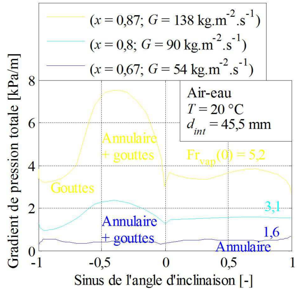
Figure 4-14 Evolution du gradient de pression totale avec le sinus de l'angle d'inclinaison d'après l'étude de Spedding et al. (1982) pour des titres en vapeur supérieurs à 0,4
