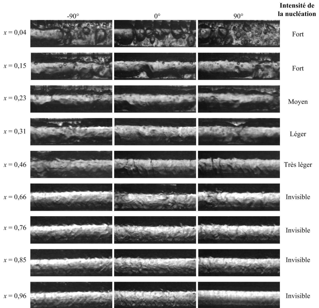
Figure 5-5 Evolution de l'écoulement et de l'intensité de la nucléation avec le titre en vapeur pour une vitesse massique de 300 \text{ kg.m}^{-2}.\text{s}^{-1} , une densité de flux transmis de 13,5 \text{ kW.m}^{-2} pour les configurations verticales et la configuration horizontale
