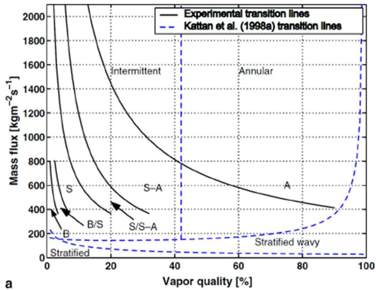
Figure 1-6 Superposition des cartes d'écoulement de Revellin et al. (2006) et de Kattan et al. (1998)
