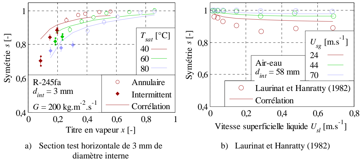
Figure 3-16 Prédiction de la symétrie pour des points de a) la base de donnée en section horizontale avec des températures de saturation de 40, 60 et 80 °C et une vitesse massique de 200 \text{ kg.m}^{-2}.\text{s}^{-1} , b) la base de données de Laurinat et Hanratty (1982) pour des vitesses superficielles de l'air de 24, 44 et 70 m.s -1
