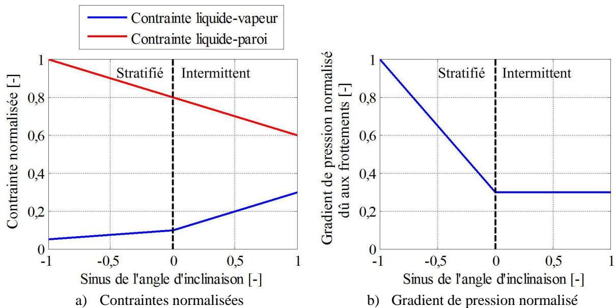
Figure 4-20 Schéma de l'évolution (a) des contraintes normalisées avec l'inclinaison ; (b) du gradient de pression dû aux frottements avec l'inclinaison
