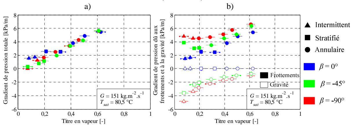
Figure 4-16 Evolution du gradient de pression totale (a) et des composantes du gradient de pression (b) en fonction du titre en vapeur pour un d_{int} = 1,6 \text{ mm} , G = 151 \text{ kg.m}^{-2}.\text{s}^{-1} , T_{sat} = 80,5 \text{ °C} et \beta = 0^\circ, -45^\circ et -90^\circ (descendants)
