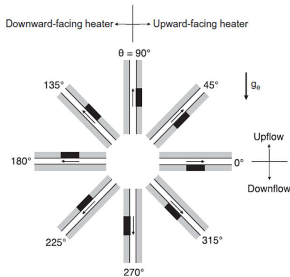
Figure 1-32 Schéma du chauffage asymétrique pour les inclinaisons testées par Konishi et al. (2013)
