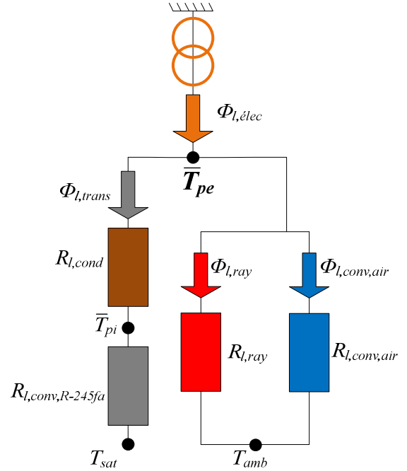
Figure 2-22 Schéma électrique équivalent du bilan local
