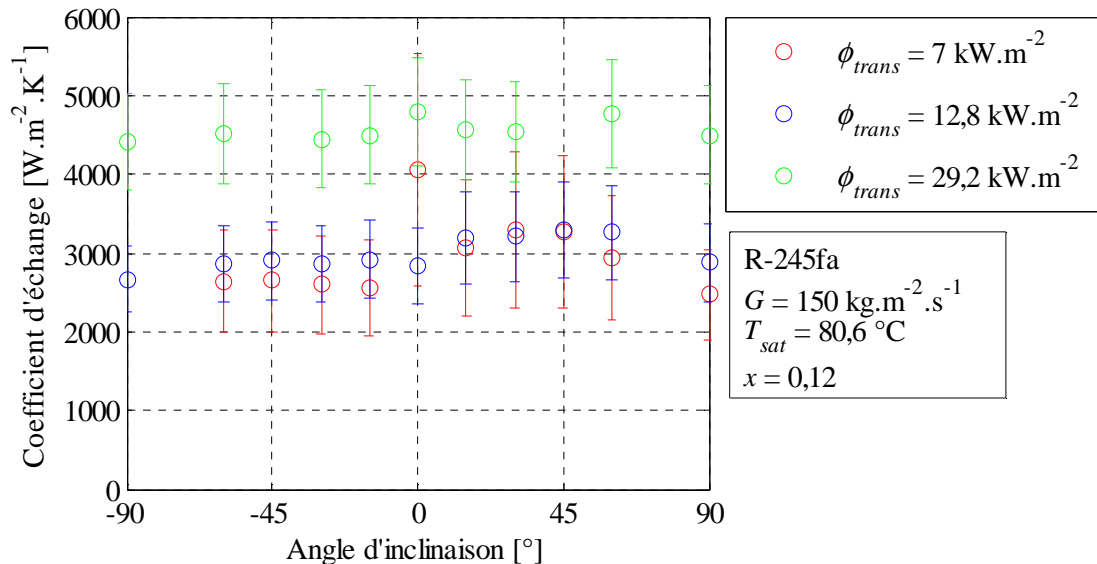
Figure 5-22 Evolution du coefficient d'échange avec l'angle d'inclinaison pour une température de saturation de 80,6 \text{ °C} , un titre en vapeur de 0,12, une vitesse massique de 150 \text{ kg.m}^{-2}.\text{s}^{-1} et des densités de flux transmis de 7, 12,8 et 29,2 \text{ kW.m}^{-2}
