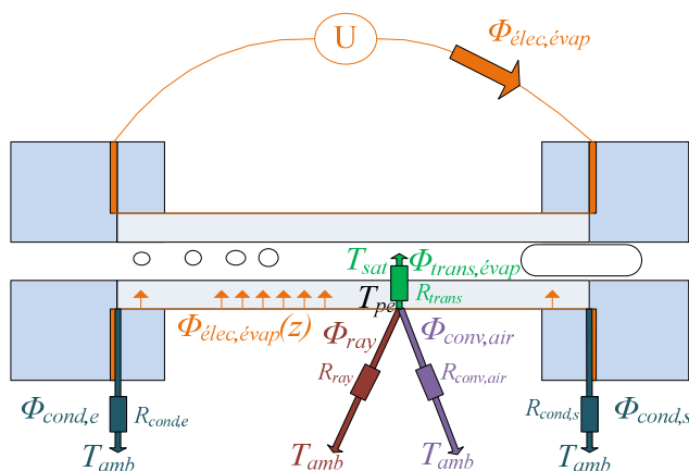
Figure 2-33 Schéma du Modèle thermique global de l'évaporateur
