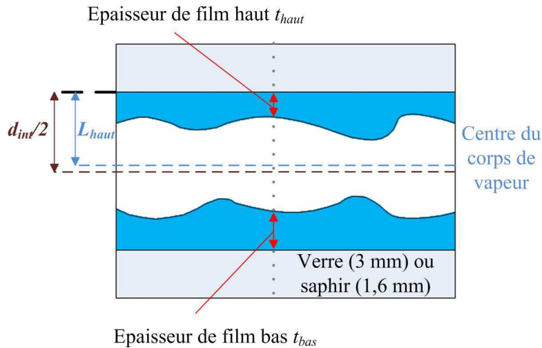
Figure 3-1 Position du centre du corps de vapeur
