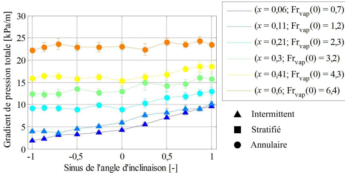
Figure 4-10 Evolution du gradient de pression totale avec le sinus de l'angle d'inclinaison pour d_{int} = 1,6 \text{ mm} , G = 300 \text{ kg.m}^{-2}.\text{s}^{-1} et x = 0,06, 0,11 et 0,21, 0,3, 0,41 et 0,6
