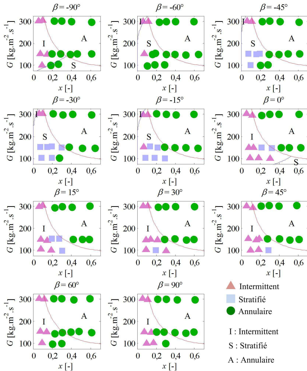
Figure 3-26 Cartes d'écoulement du modèle de Crawford et al. (1985)
