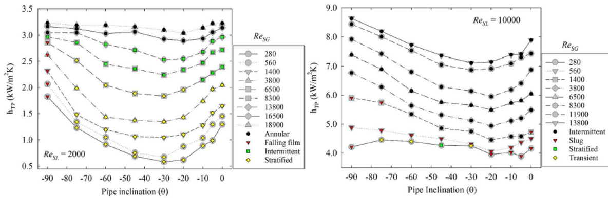
Figure 1-27 Evolution du coefficient d'échange avec l'angle d'inclinaison pour différents nombres de Reynolds superficiels de liquide et de gaz en écoulement incliné descendant (Bhagwat and Ghajar, 2017)
