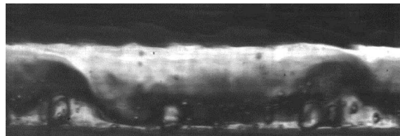
Figure 5-21 Image représentative de l'écoulement pour G = 600 \text{ kg.m}^{-2}.\text{s}^{-1} , x = 0,06 , \phi = 13,5 \text{ kW.m}^{-2} dans le cas horizontal
