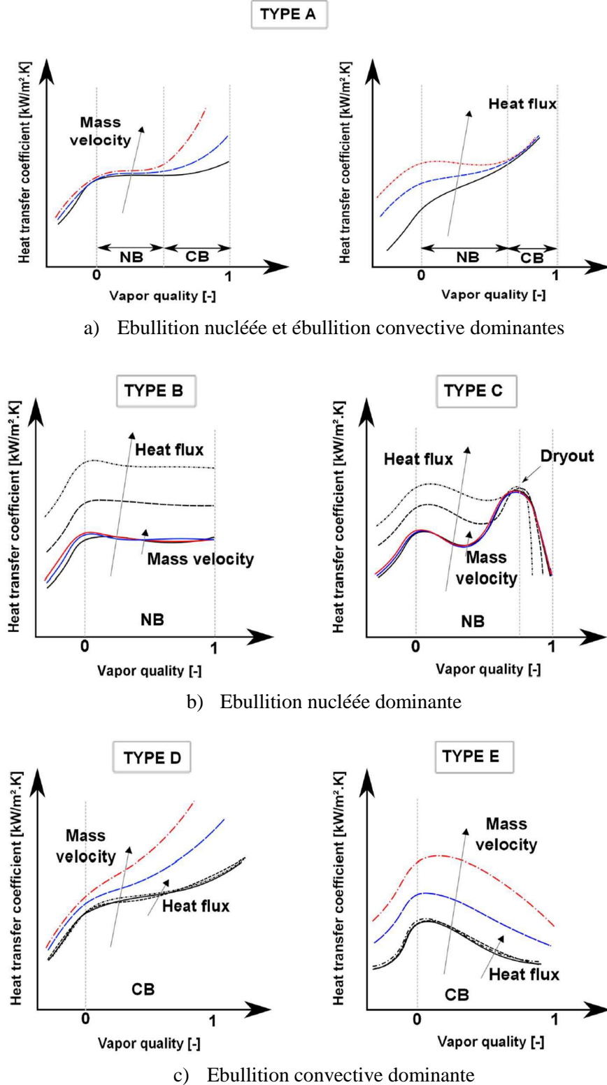
Figure 1-23 Types d'évolutions du coefficient d'échange avec le titre en vapeur dans les cas d'ébullition convective et ébullition nucléée dominantes (a), d'ébullition nucléée dominante (b) et d'ébullition convective dominante (c) (CB : ébullition convective ; NB : ébullition nucléée) (Charnay et al., 2014)
