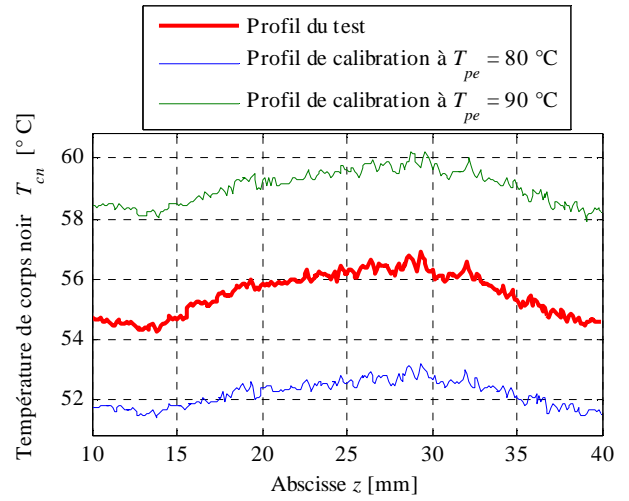
Figure 2-16 Profils de température de corps noir après rephasage
