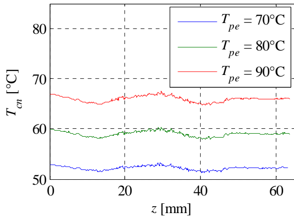
Figure 2-10 Exemple de profil de température moyenne de corps noir le long du tube pour différentes températures réelles de paroi
