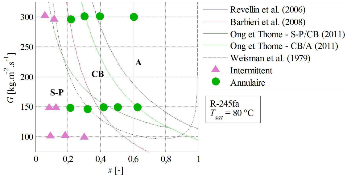
Figure 3-23 Transitions entre les régimes d'écoulements intermittent et annulaire prédites par Revellin et al. (2006), Barbieri et al. (2008), Ong et Thome (2011) et Weisman et al. (1979)
