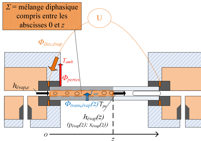
Figure 2-31 Bilan thermique global du système {mélange diphasique compris entre l'abscisse 0 et z }
