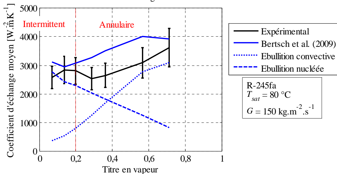
Figure 5-29 Evolution des prédictions du modèle de Bertsch et al. (2009) en fonction du titre en vapeur pour une vitesse massique de 150 \text{ kg.m}^{-2}.\text{s}^{-1} en configuration horizontale
