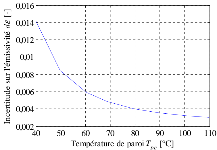
Figure 2-14 Evolution de l'incertitude sur l'émissivité avec la température de paroi
