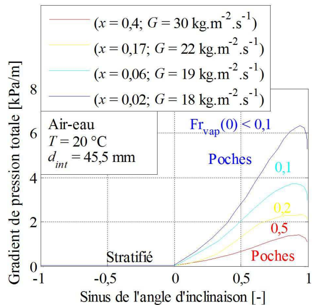
Figure 4-12 Evolution du gradient de pression totale avec le sinus de l'angle d'inclinaison de l'étude de Spedding et al. (1982) pour des titres en vapeur inférieurs à 0,4
