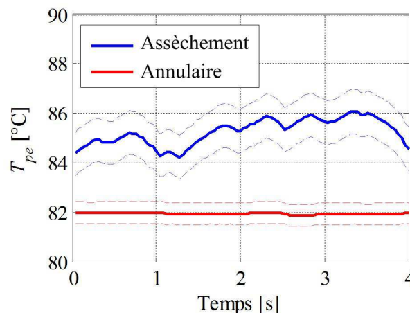
Figure 5-31 Evolution temporelle de la température de paroi extérieure dans les cas d'un régime d'assèchement et d'un régime annulaire
