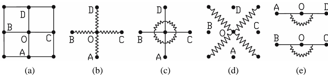
Figure 1.32 Modélisation d'une particule O connectée à ses quatre voisins (a) avec modélisation de l'élongation (b), du cisaillement (c) et (d), et de la flexion (e) [SZE 05]
