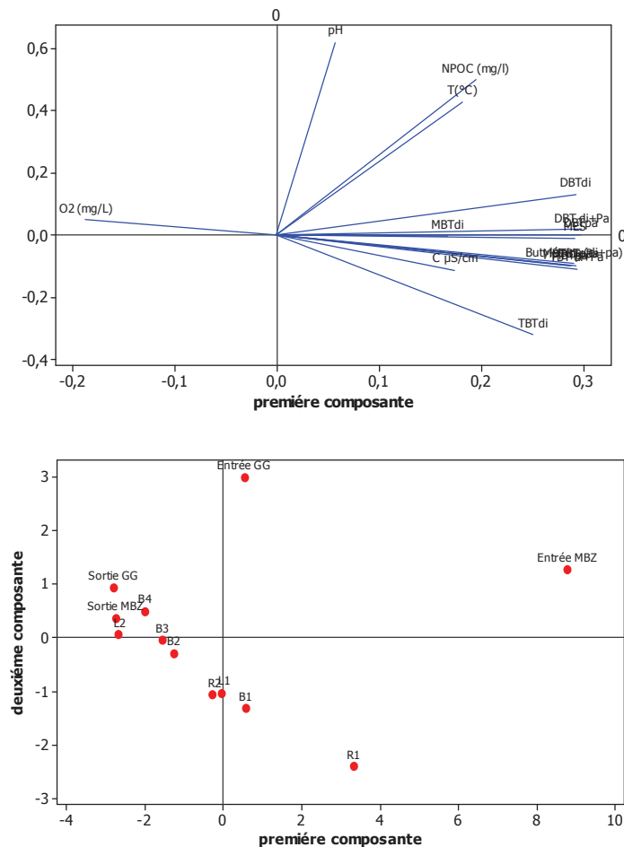
Figure 24 : Analyse en composantes principale des concentrations en butylétain dans le surnageant (matrices dissoutes et particulaires) et les paramètres physicochimique mesuré in-situ
