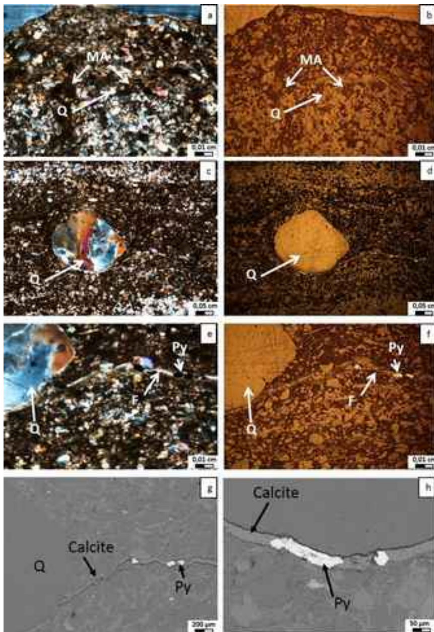
Figure 5.5 - Micrographies (FM5): (a, b) de la matrice argileuse brunâtre (MA) emballant des passages composés presque exclusivement de quartz (Q); (c, d) claste quartzueux polycristallin (Q) de taille millimétrique; (e, f) disposition disymétrique de lamines indiquant un courant de la gauche vers la droite et montrant la présence d'un filonnet (F) localisé dans la zone de plus faible énergie, et (g, h) partiellement rempli de calcite et ponctuellement par des granules pyriteux (Py).
