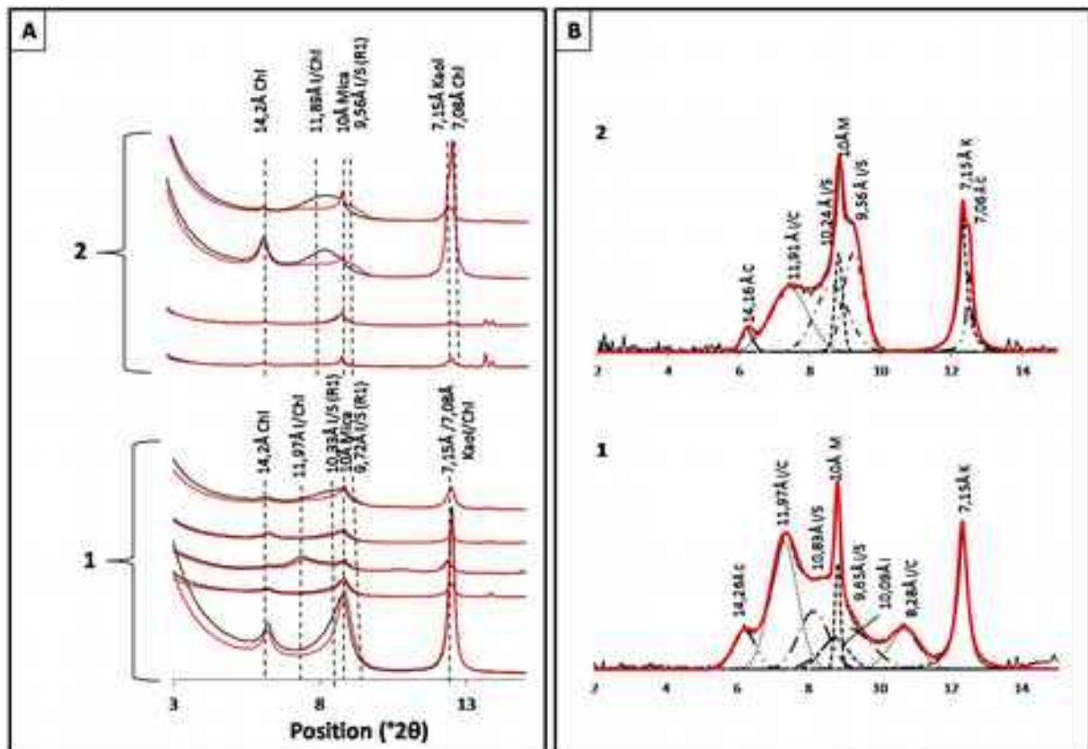
Figure 5.42 Diffractogrammes des préparations orientées (<2 µm) séchées à l’air (noir) et saturées à l’éthylène glycol (rouge) montrant : A) l’évolution des minéraux interstratifiés dans les séquences V2lom (A1) et V2yam (A2) de la formation FM; B) les déconvolutions types des fractions <2 µm glycolées des séquences V2lom (B1) et V2yam (B2).
