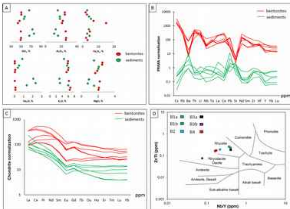
Figure 6.15 A) Comparaison des teneurs en éléments majeurs entre les bentonites et leurs sédiments hôtes sous- et sus-jacents dans les formations FM et FY du bassin de Podilya; B) Spider diagramme montrant la distribution des éléments traces normalisés PRIMA (Thompson et al. , 2012); D) Position des bentonites par rapport au champ de compositions des rhyolites dans le diagramme Nb/Y-Zr/Ti (d'après Winchester & Floyd, 1977).
