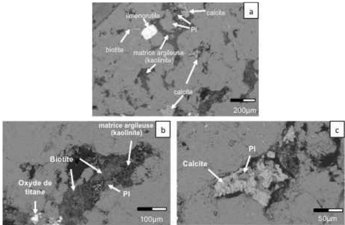
Figure 5.33 Micrographies MEB (UUF33) montrant : (c) la présence de ciments argileux riche en kaolinite et calcique dans la porosité des niveaux quartzeux; (d) du détail de la matrice argileuse (kaolinite) (d) et calcique (e) dans l'espace entre granulaire (Annexe 2 Tableau 6.2).
