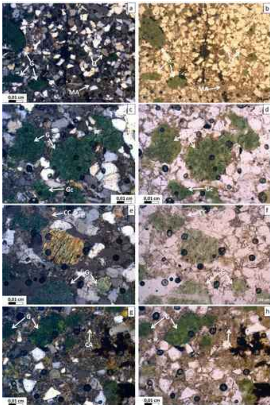
Figure 5.37 Micrographies (UUF40): (a, b) du faciès grésopélique quartzeux (Q) riche en glauconite (G) et cimenté par une matrice argileuse (MA); (c, d) d'amas framboïdaux de glauconite (G) faisant ciment (Gc) ; (e, f) plage micacée chloritisée (Ch) et ciment calcique (CC) ; (g, h) hétérogénéité de teintes de la glauconite traduisant la variation de ses teneurs en Mg.
