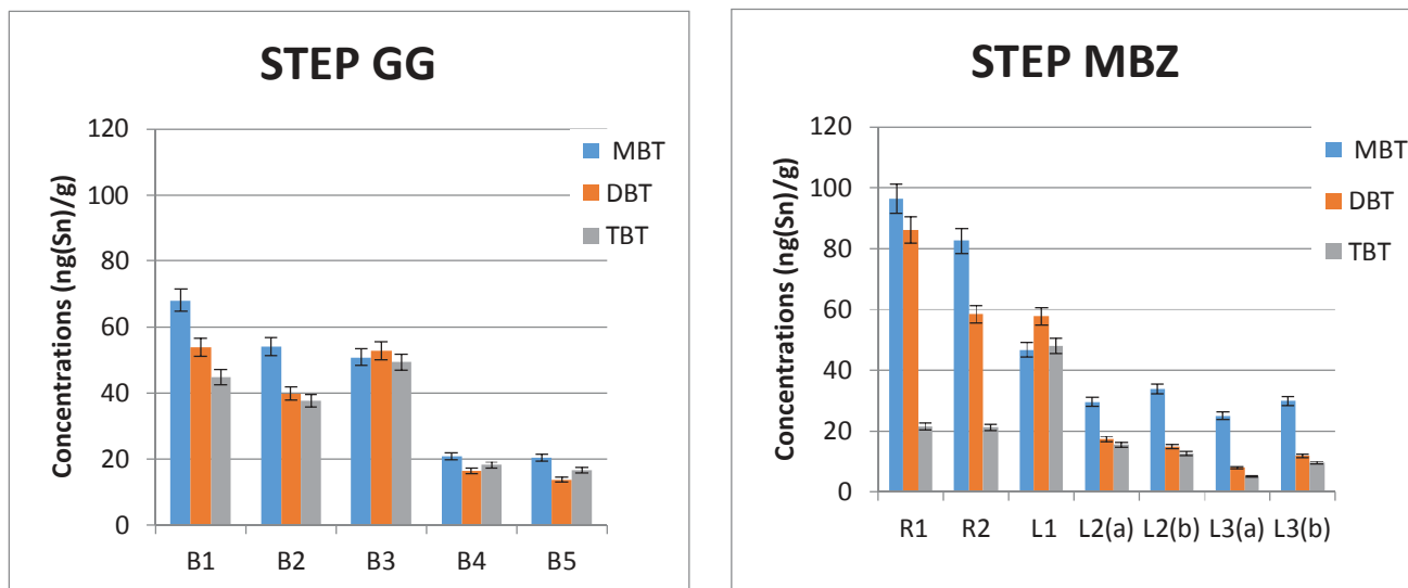
Figure 25: Concentrations moyennes en butylétains dans les boues de fond de chaque bassin (a-
