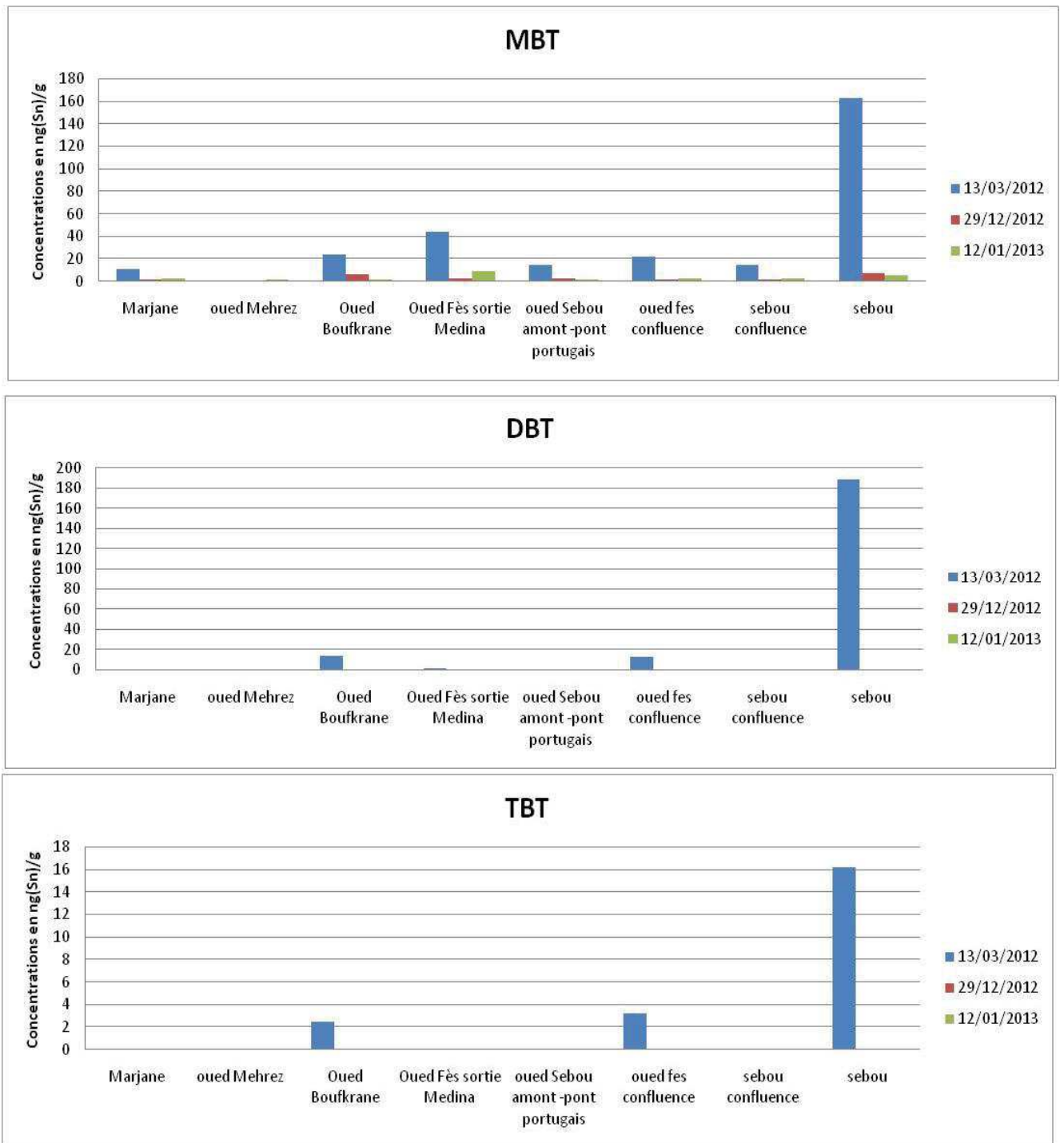
Figure 43 : Concentrations en ng(Sn)/g en MBT, DBT, et TBT mesuré dans les sédiments provenant de chaque point de prélèvement
