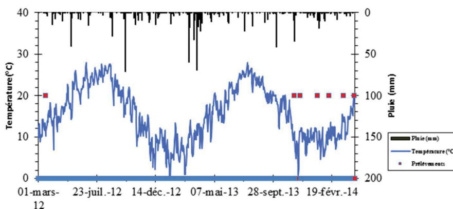
Figure 7 : Campagnes de prélèvements, chroniques de pluie (mm) et de température de l'air (°C)
