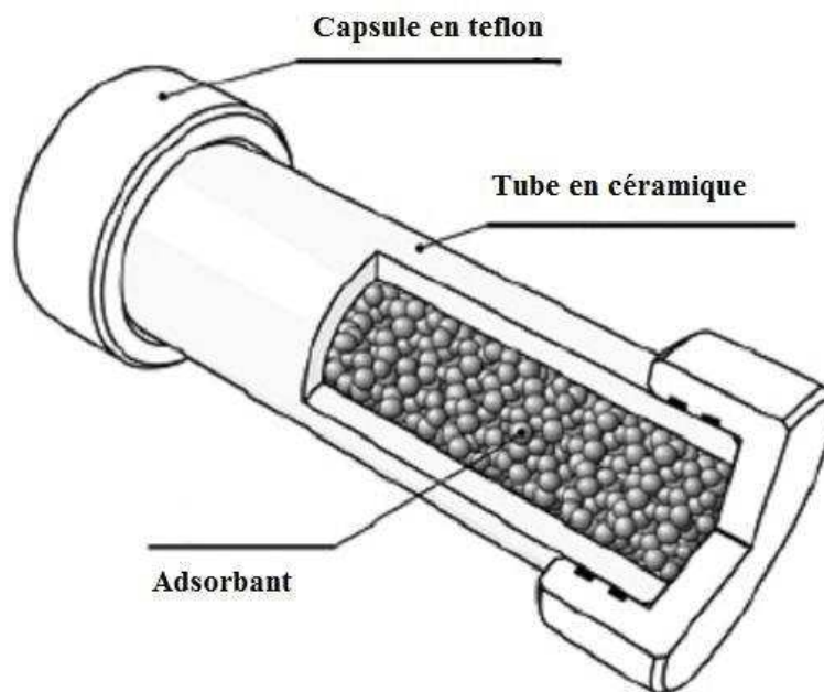
Figure 34 : Schéma d'un dosimètre en céramique (d'après Nyoni et al., 2010)
