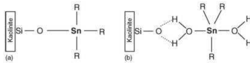
Figure 3 : Schéma d'adsorption du TBT sur le groupe Si-O à la surface de la kaolinite(a) adsorption d'une molécule de TBT tétraèdre et (b) adsorption d'une molécule de TBT trigonal-bipyramidal hydraté, R correspond au groupe butyl. (d'après Hoch et Bandara, 2005)
