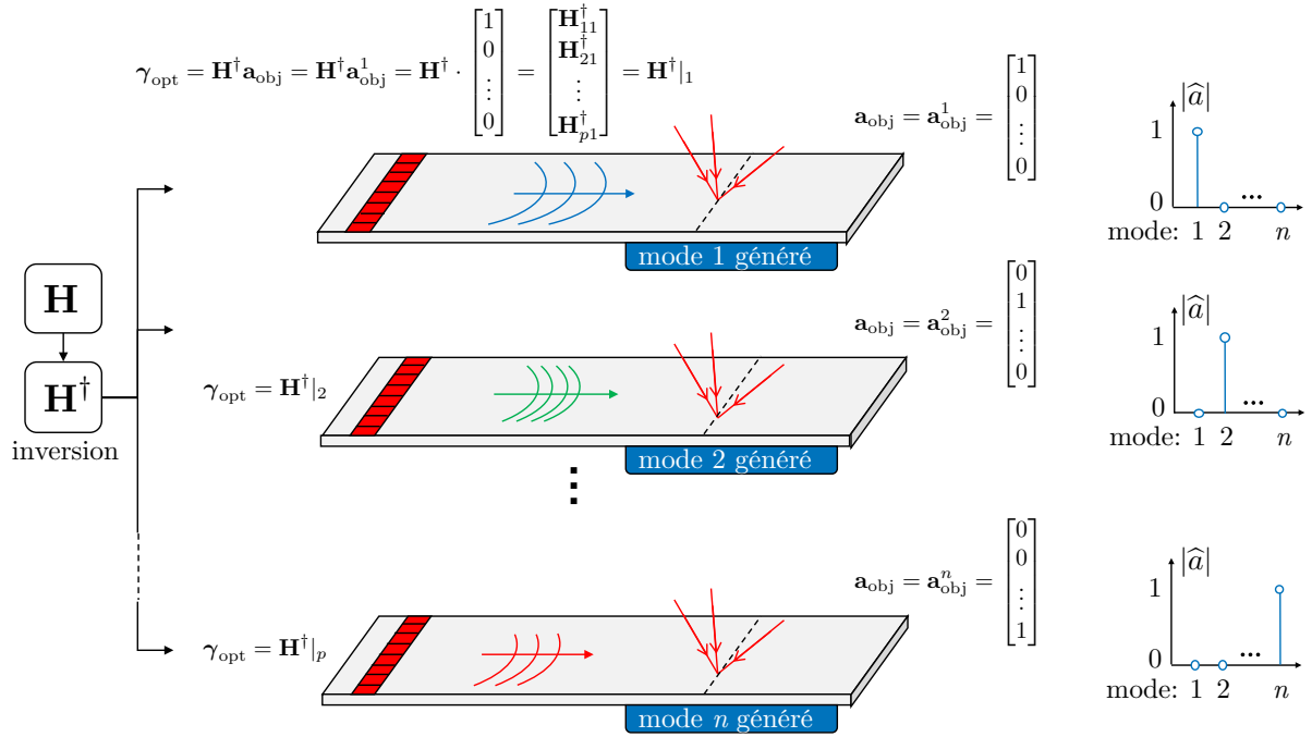
FIGURE 3.5 – Illustration de l'excitation simultanée des éléments afin de générer chaque mode de manière pure.
