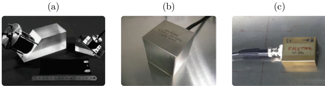
FIGURE 2.10 – Exemples de sondes ultrasonores au contact : (a) sonde à incidence oblique montée sur sabot [13], (b) sonde multi-élément [59] et (c) EMAT [9] .
