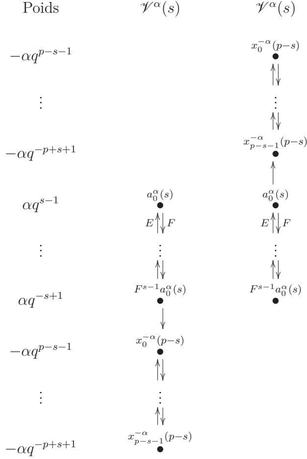
FIGURE I.2.B – Représentation diagrammatique de \mathcal{V}^\alpha(s) et \bar{\mathcal{V}}^\alpha(s) .
