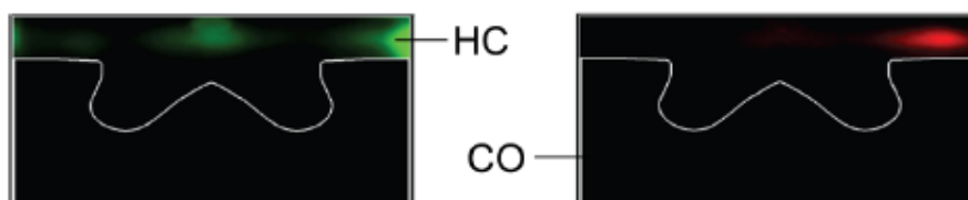
Figure 16: Visualisation LIF d'HC et CO dans le cylindre [4]
