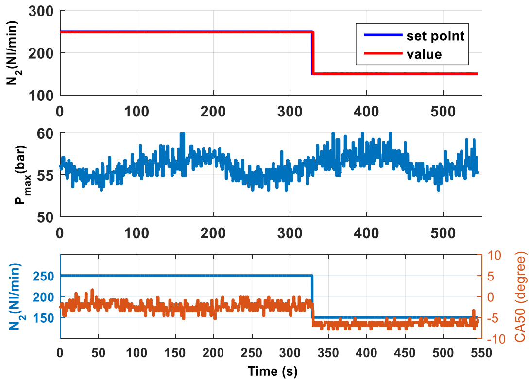
Figure 179 : variation de P_{max} et CA50 lors d'un échelon descendant d'EGR à charge élevée
