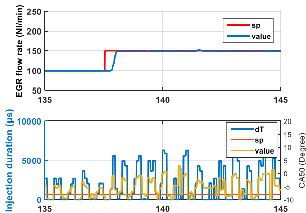
Figure 253: CA50 mesurée et consigne avec contrôle lors de transition entre deux points de fonctionnement
