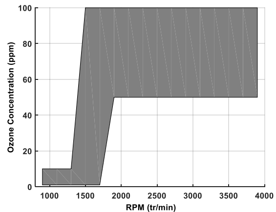
Figure 115: concentration d'ozone pour différents régimes
