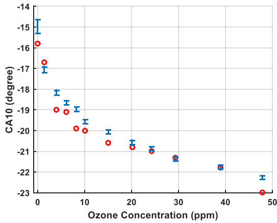
Figure 263: CA10 en fonction de la concentration d'ozone
