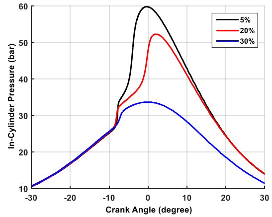
Figure 96: Pression cylindre en fonction de l'angle vilebrequin pour différents taux d'EGR ( \phi=0.7 ; rpm=900 tr/min)
