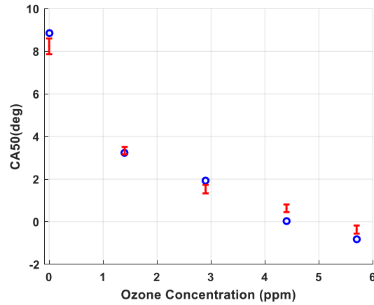
Figure 78: CA50 en fonction de la concentration d'ozone
