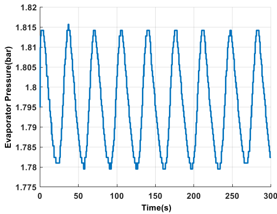
Figure 303: pression de l'évaporateur en fonction du temps
