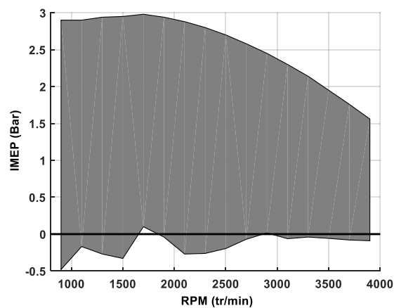
Figure 118: cartographie d'IMEP
