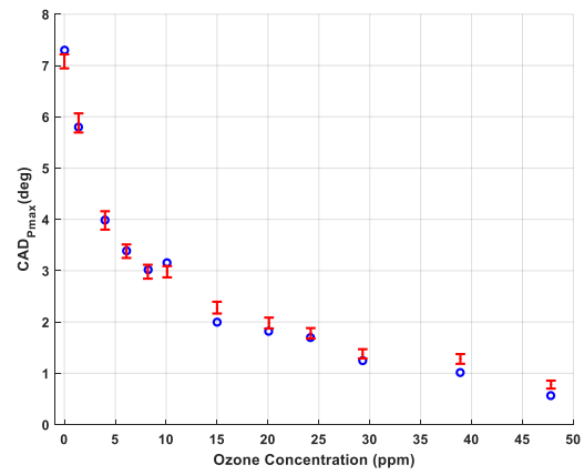
Figure 74: CAD_{P_{max}} en fonction de la concentration d'ozone
