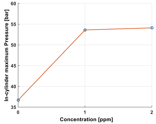
Figure 126: P_{max} pour 0°C et différentes concentration d'ozone
