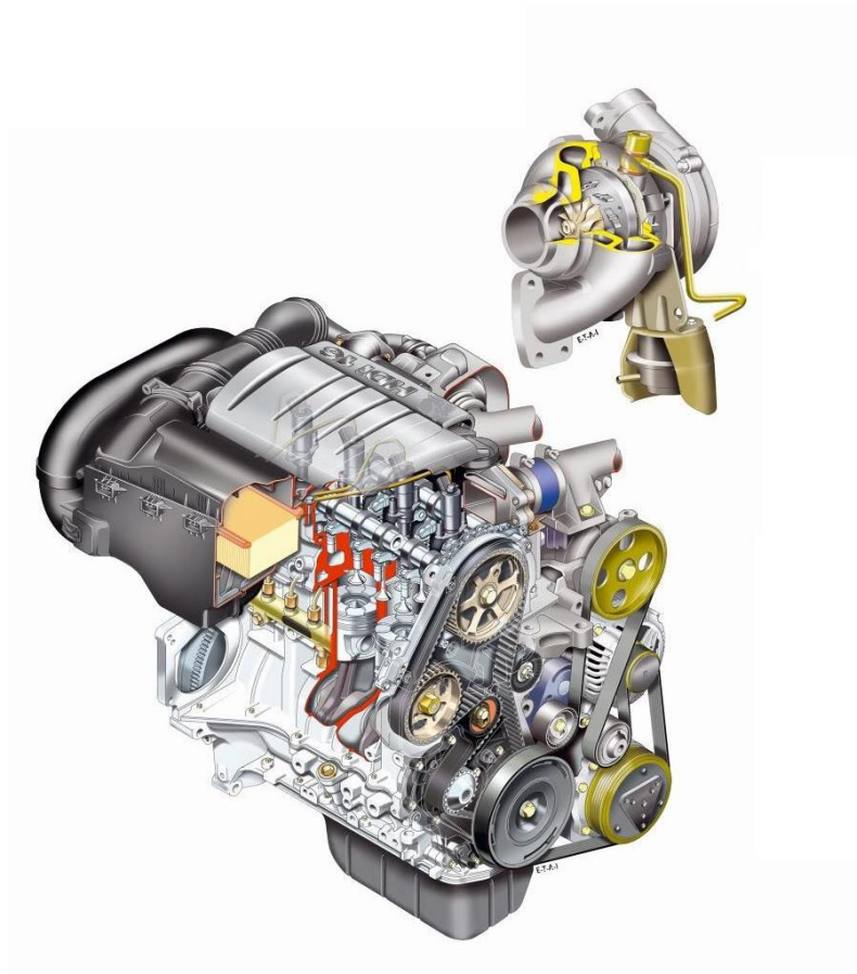
Figure 130: moteur DV6 TED4
