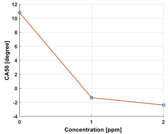
Figure 128: CA50 pour 0°C et différentes concentration d'ozone
