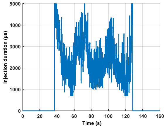
Figure 230: durée d'ouverture de l'injecteur
