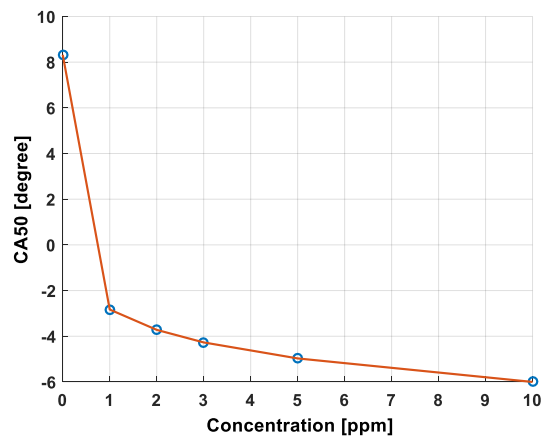
Figure 92: CA50 en fonction de la concentration d'O 3
