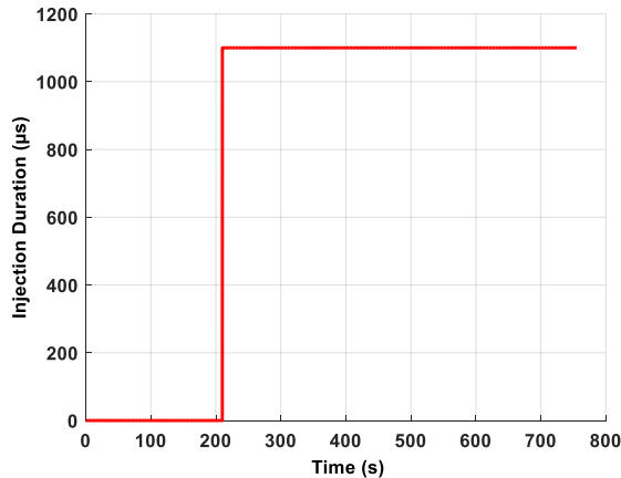
Figure 192: durée d'ouverture de l'injecteur
