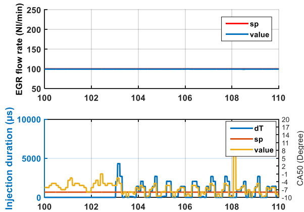
Figure 251: CA50 mesurée et consigne avec contrôle pour un même point de fonctionnement
