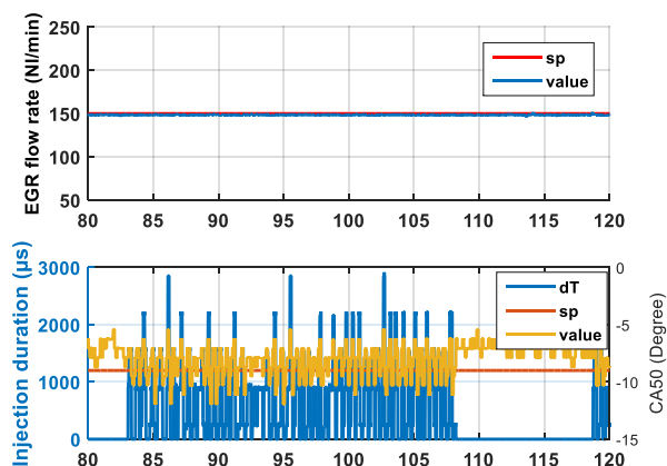
Figure 241: CA50 du point (8200µs, 150 NI/min) sans et avec contrôle
