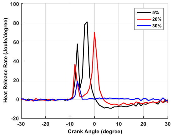
Figure 95: taux de dégagement de chaleur en fonction de l'angle vilebrequin pour différents taux d'EGR ( \phi=0.7 ; rpm=900 tr/min)
