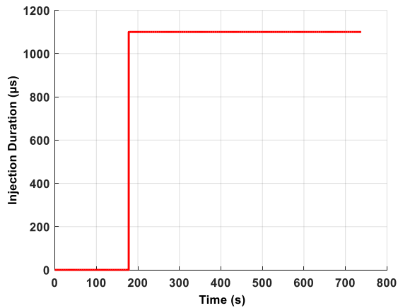
Figure 186: durée d'ouverture de l'injecteur
