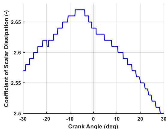
Figure 70: évolution de C_0 au cours du cycle
