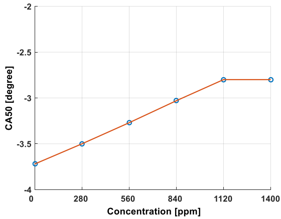
Figure 88: CA50 en fonction de la concentration de CH 2 O
