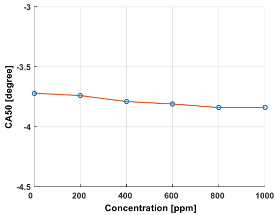
Figure 90: CA50 en fonction de la concentration de H 2
