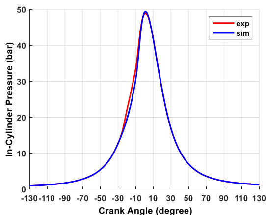
Figure 223 : pression cylindre expérimentale et simulée en fonction d'angle vilebrequin
