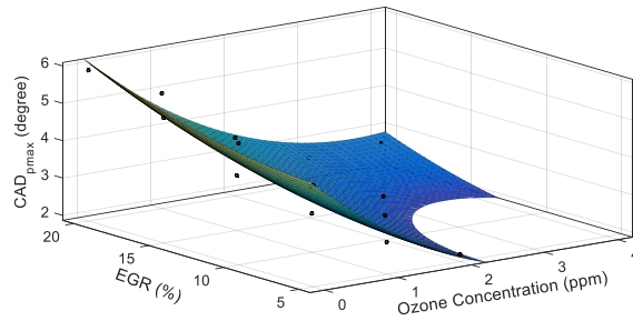
Figure 167: CAD_{pmax} en fonction de la concentration d'ozone et du taux d'EGR
