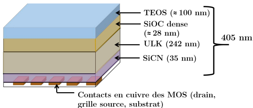
Figure 3-7 Vue 3D schématisée d'un substrat issu des plaques 300 mm de diamètre provenant de STMicroelectronics et utilisées pour la fabrication de dispositifs.
