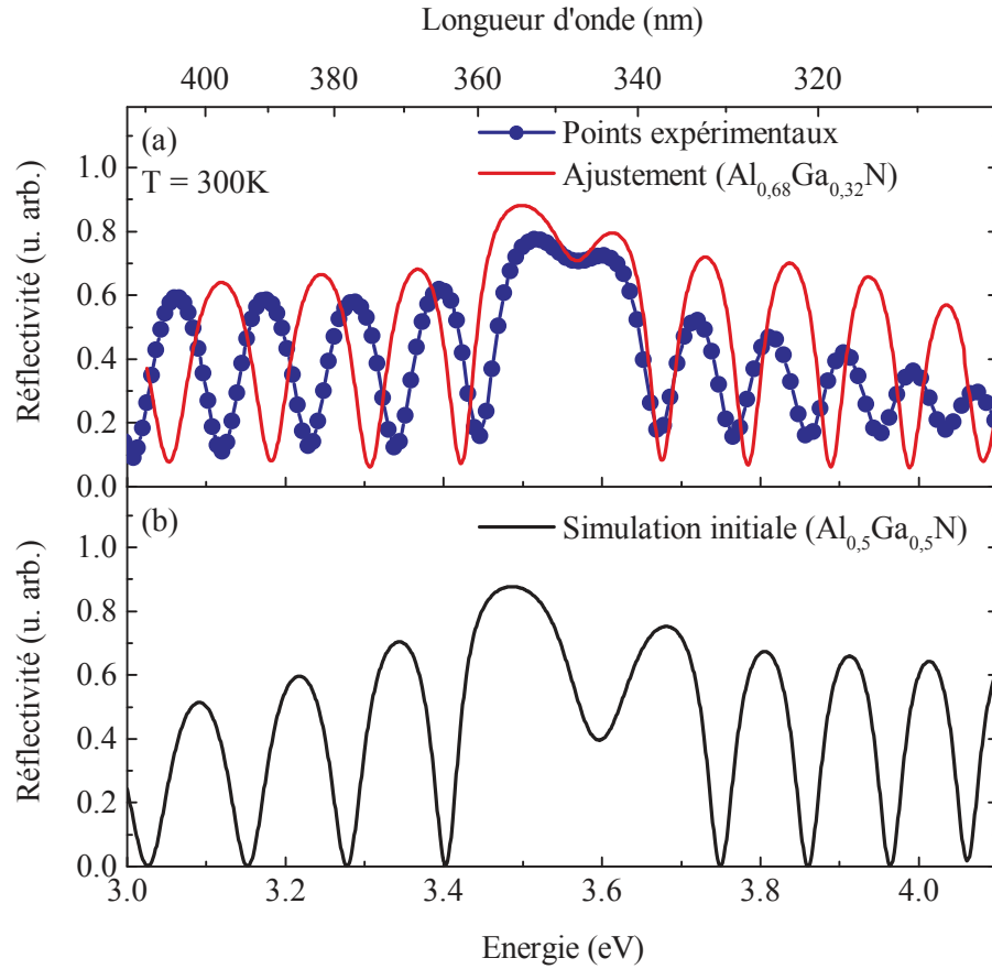
FIGURE 2.32 – (a) Réflectivité de la microcavité Al_{0,5}Ga_{0,5}N (A1833) et son ajustement représenté respectivement par des points bleus et un trait continu rouge. (b) Calcul initial de la réflectivité.
