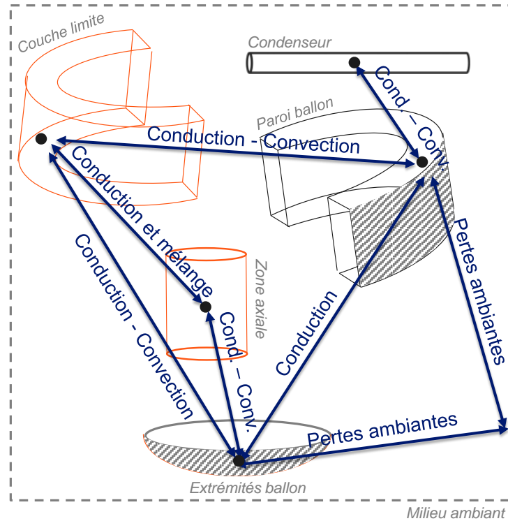
Figure II-11. Illustration des échanges thermiques considérés dans le bilan d'énergie par zone du ballon. Partie fluide en orange et solide en grise.
