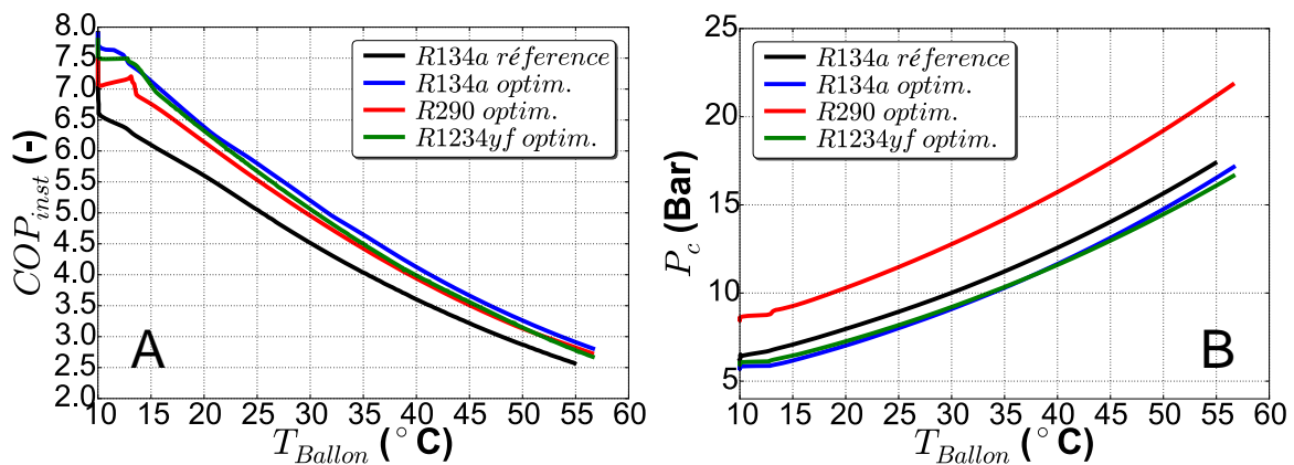
Figure V-4. COP instantané (A) et pression de condensation (B) des CET optimisés pour le R134a, le propane et le R1234yf par rapport au CET de référence au R134a
