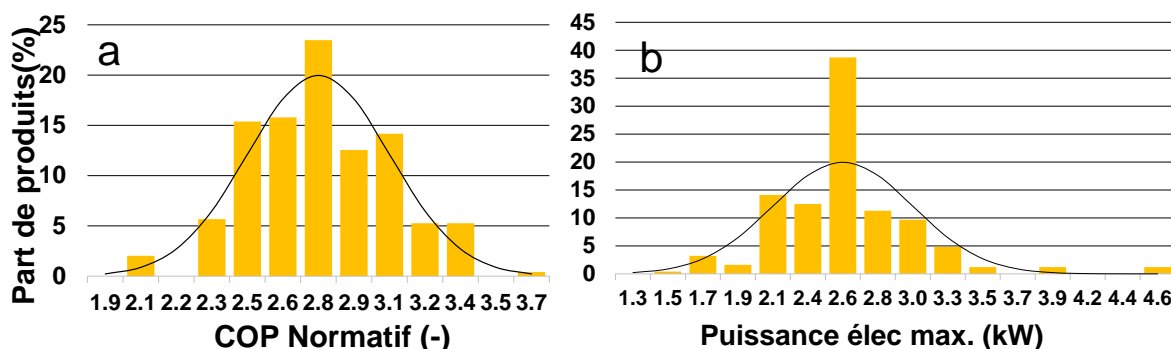
Figure I-13. Répartition des COP normatif et puissance électrique maximales des CET du marché. Source : [33]
