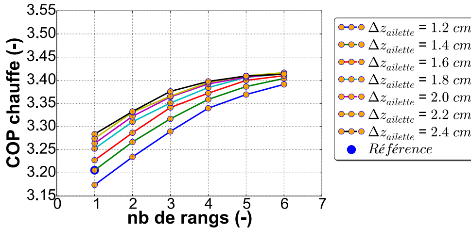
Figure IV-40. Influence de la profondeur d'ailette sur le COP de chauffe pour différents nombres de rangs de l'évaporateur et 24 tubes par rang
