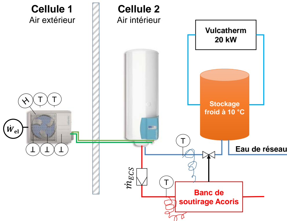
Figure III-2. Banc d'essai à EDF Lab
