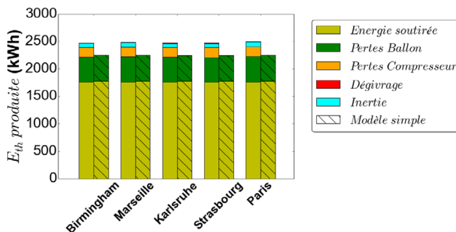
Figure IV-9. Comparaison de l'énergie thermique produite annuellement prédite par le modèle simplifié à celle calculée à l'aide du modèle détaillé pour différents climats
