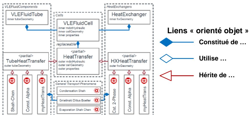
Figure II-5. Architecture orientée objet d'une cellule de fluide frigorigène sous TIL© pour le bilan d'énergie. Source : [90] [86]
