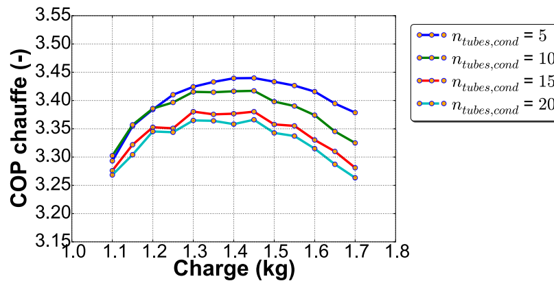
Figure IV-32. Variation du COP de chauffe pour une surface d'échange de condenseur de 1,46 m 2 , un diamètre des tubes condenseur de 3 mm et différents nombres de tubes par passe
