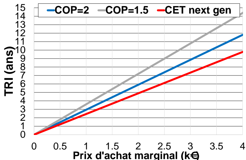
Figure V-27. Temps de retour sur investissement par rapport au prix marginal d'achat de différents CET par rapport à un CEJ
