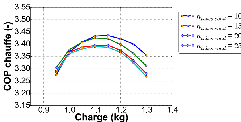
Figure IV-33. Variation du COP de chauffe pour une surface d'échange du condenseur de 1,46 m 2 , un diamètre des tubes condenseurs de 2 mm et différents nombres de tubes par passe
