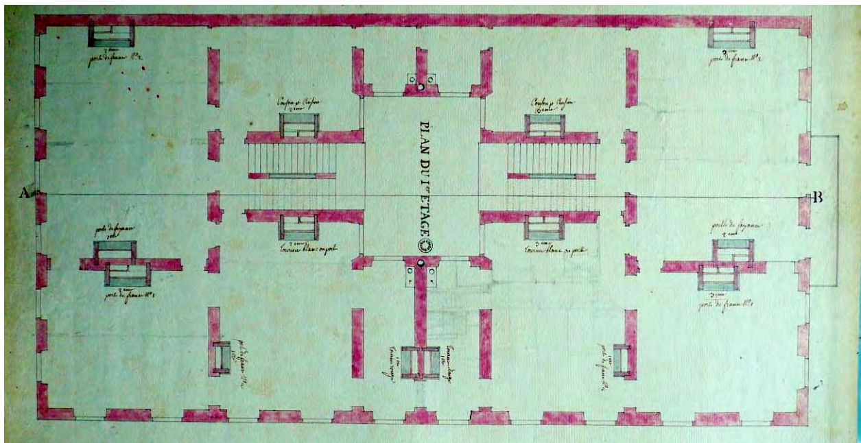
ill. 63b Maison « Trois-Façades » (milieu des années 1760). Plan du premier étage. H : 0,555 ; L : 0,350. Plume, lavis rose. AML : 3 SMO 155/5
