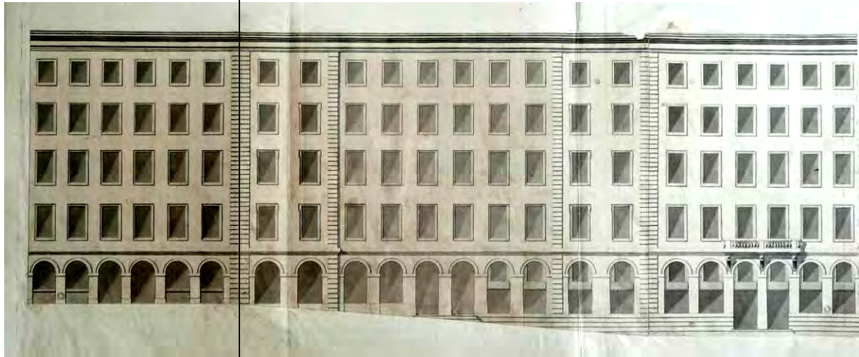
ill. 63a [p. 274] Maison « Trois-Façades » (milieu des années 1760). Développement des façades : rue royale, rue Violi, quai Lassagne. H : 0,545 ; L : 1,020. Plume et lavis gris. AML : 2 SMO 34.
