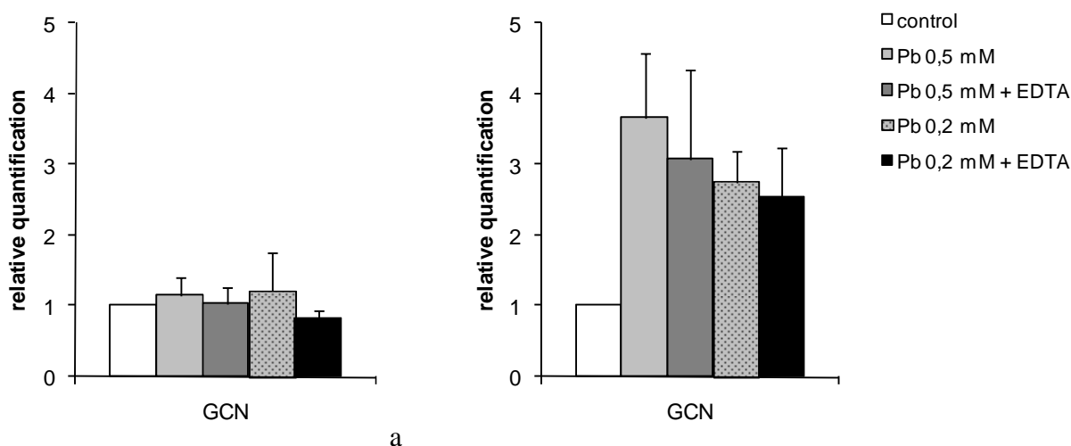
Figure 25 : Quantification des transcrits d'ARNm de LsGCN par PCR en temps réel dans les racines (a) et feuilles (b) de plantes de Lathyrus sativus , cultivées, huit jours, dans du milieu Hoagland (1/10) sans phosphate additionné de 0.5 mM Pb(NO_3)_2 , 0.5 mM Pb(NO_3)_2 + 0.5 mM EDTA, 0.2 mM Pb(NO_3)_2 , 0.2 mM Pb(NO_3)_2 + 0.2 mM EDTA ou non (control). LspUBQ a été utilisé comme gène de référence (n=3).
